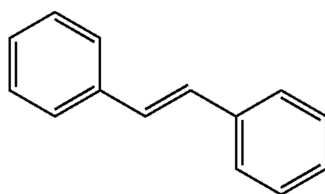
Trans-stilbene
