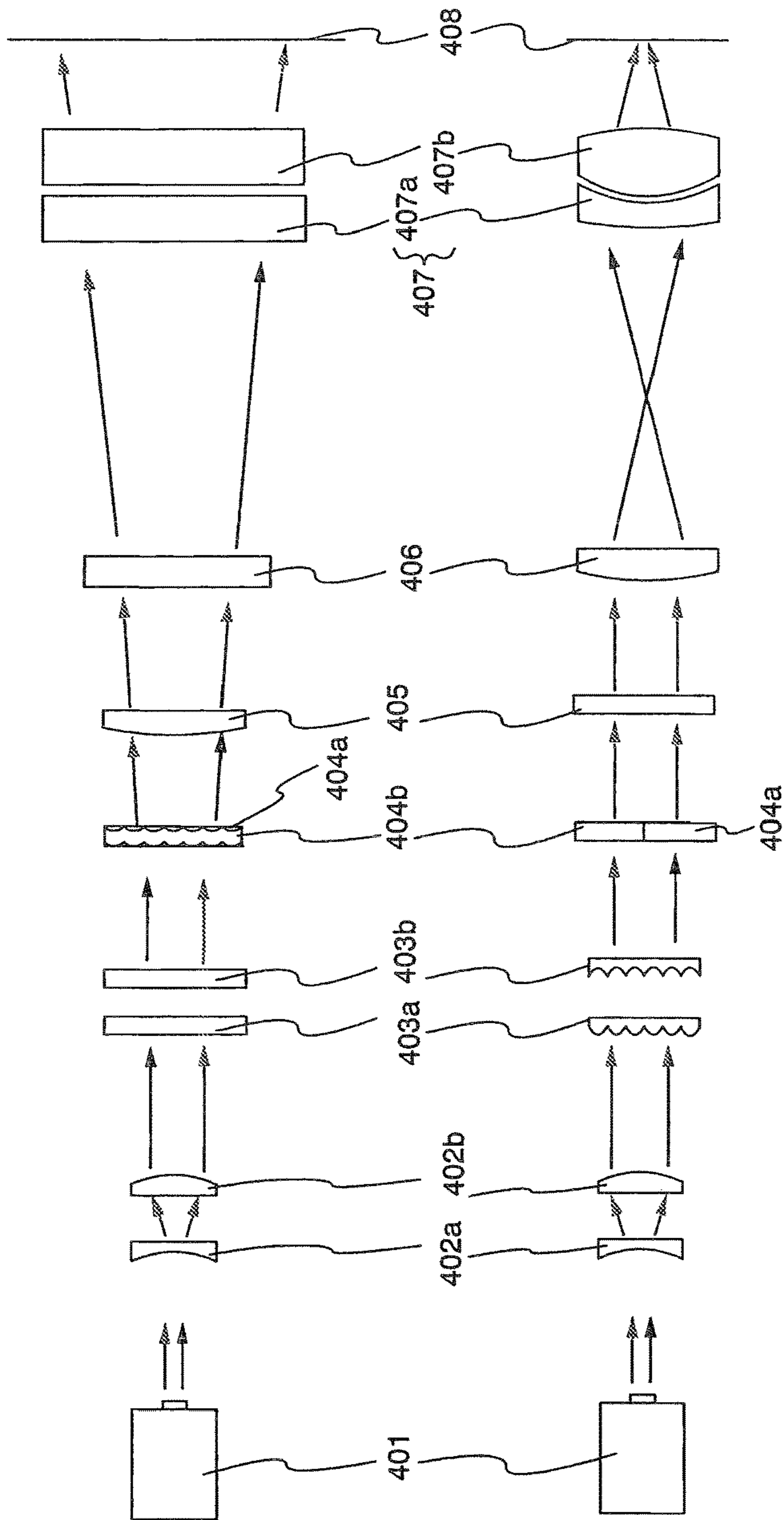
FIG. 4A
