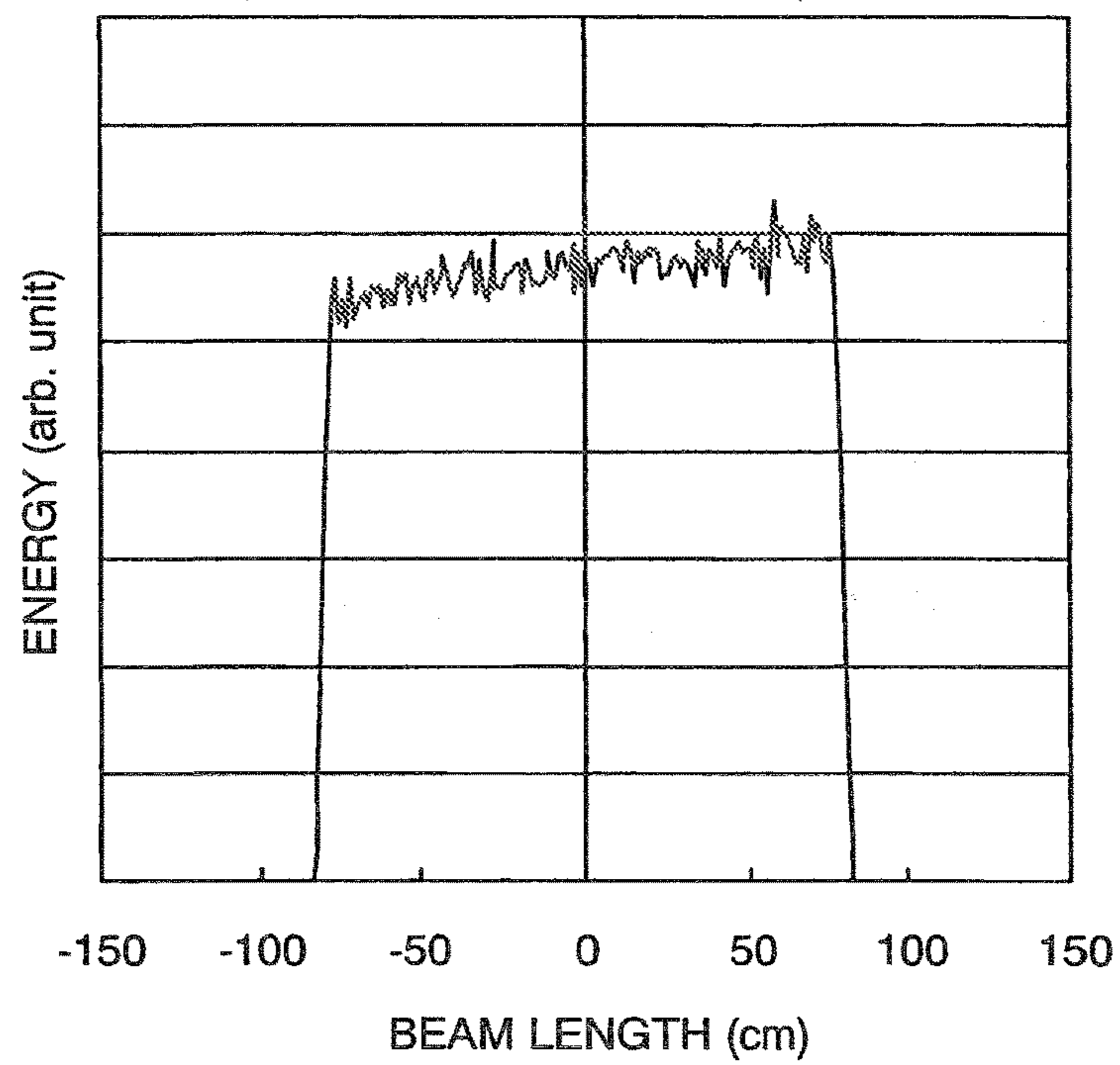
FIG. 5B
