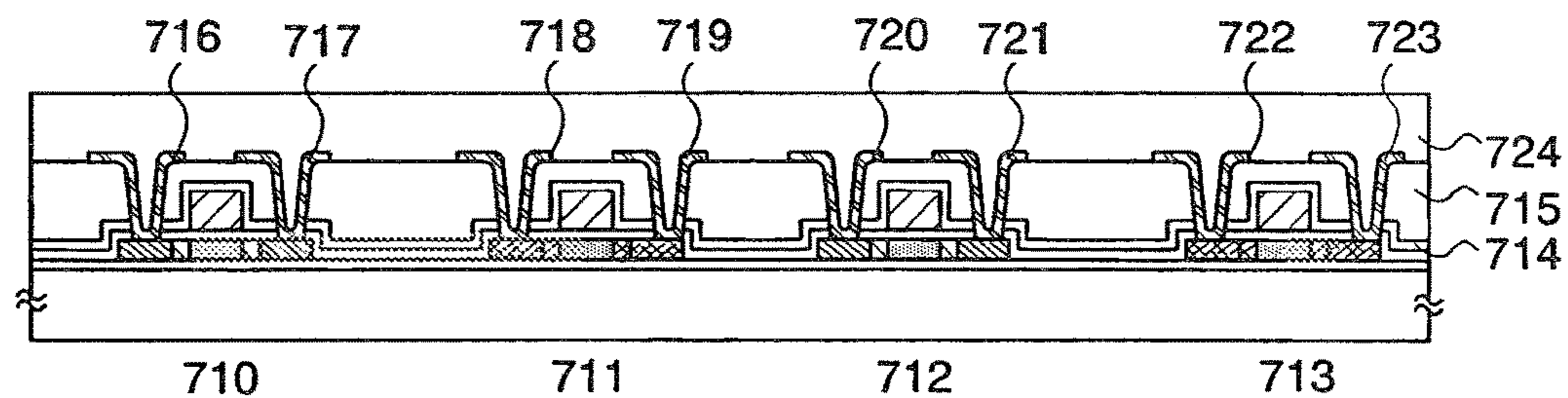
FIG. 7D
