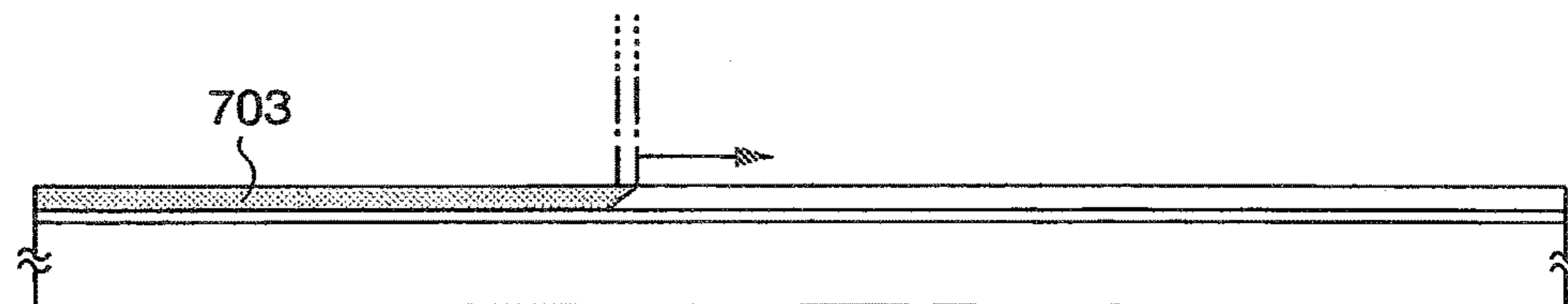
FIG. 7B
