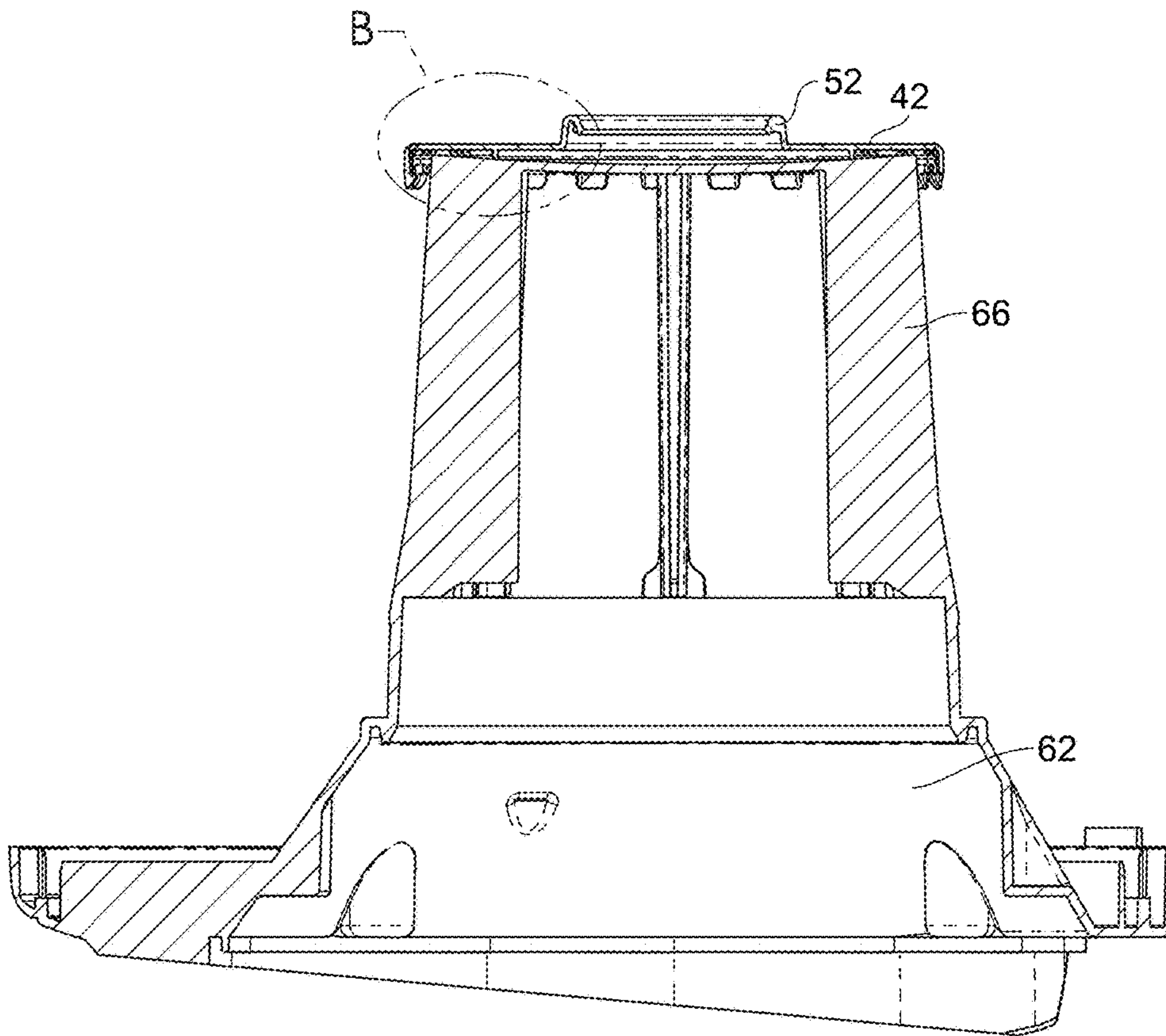
SECTION A-A
