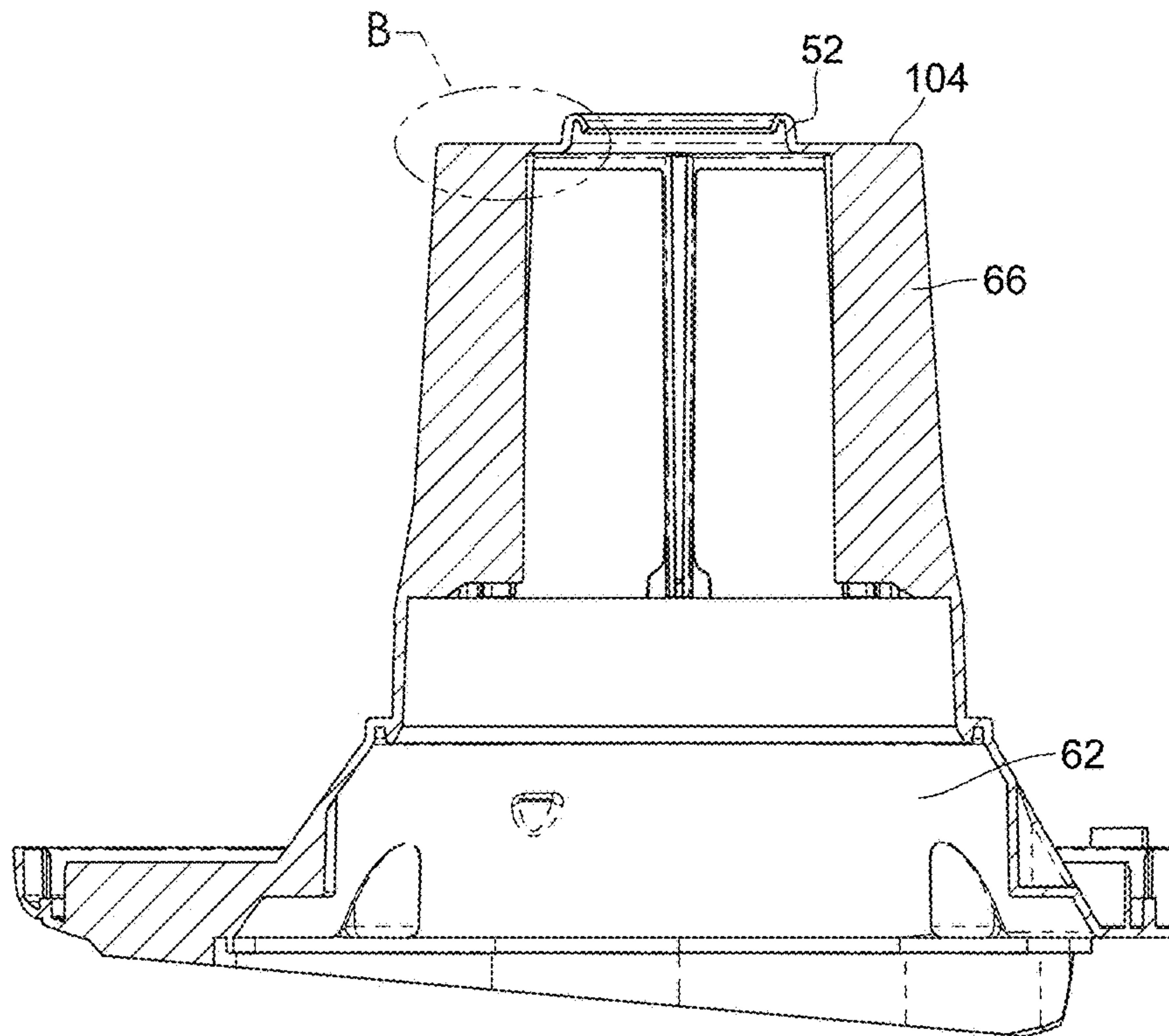
SECTION A-A
