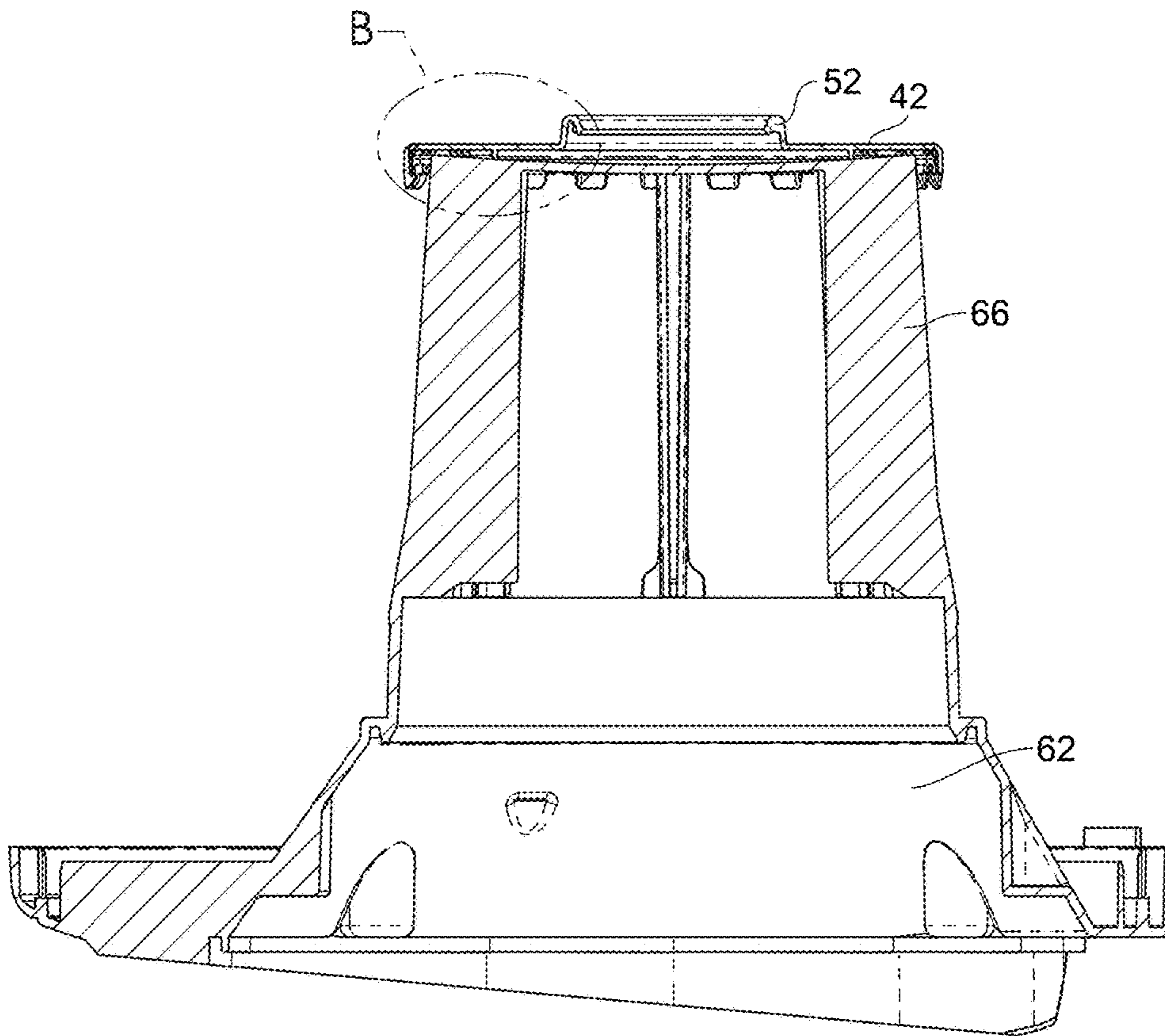
SECTION A-A
