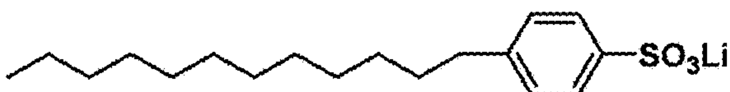
lithium 4-dodecylbenzenesulfonate
