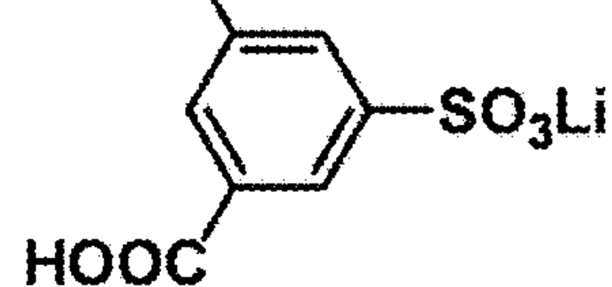
lithium 3,5-dicarboxybenzenesulfonate
