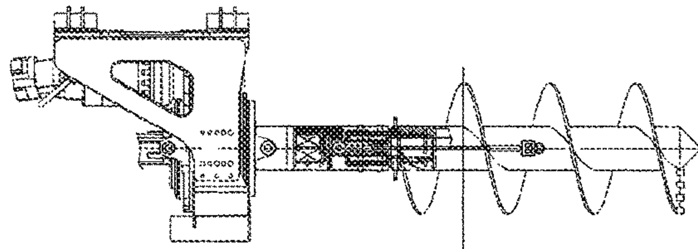
Fig. 6D
