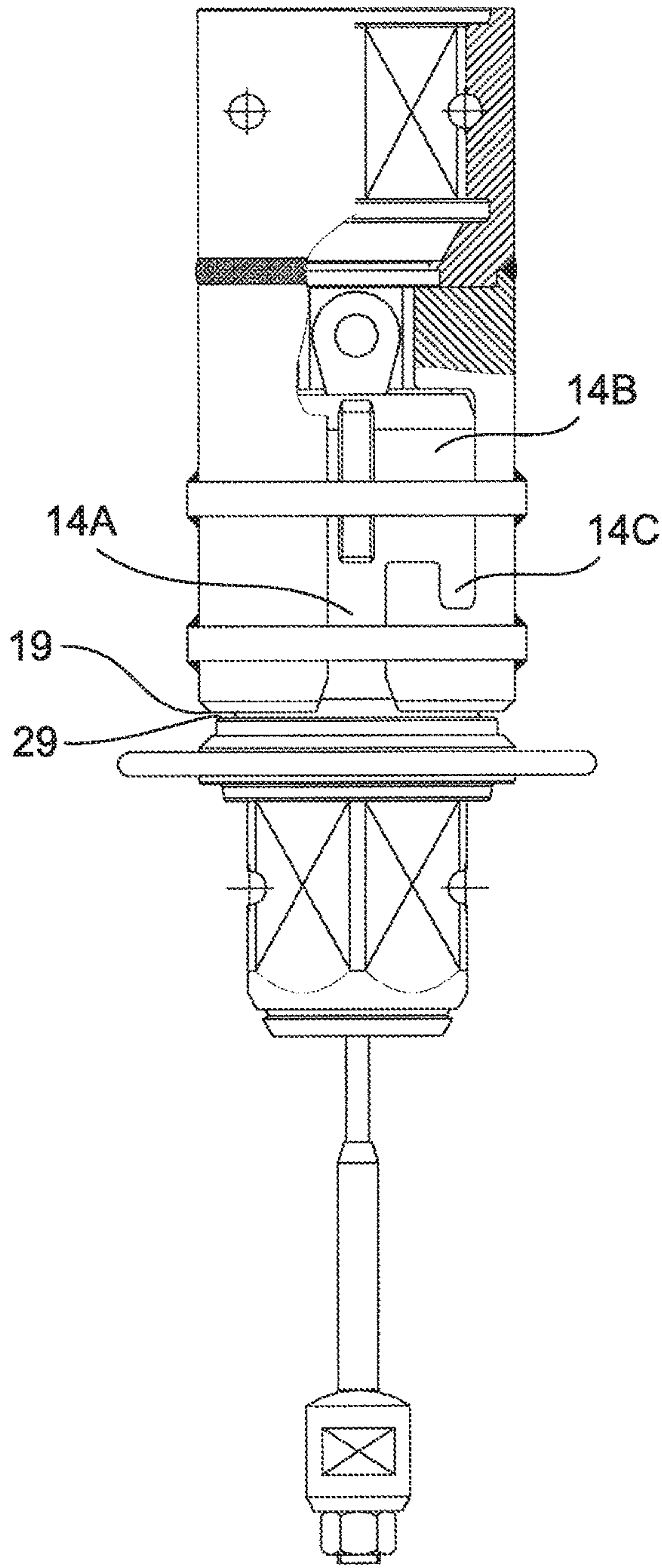
Fig. 2A
