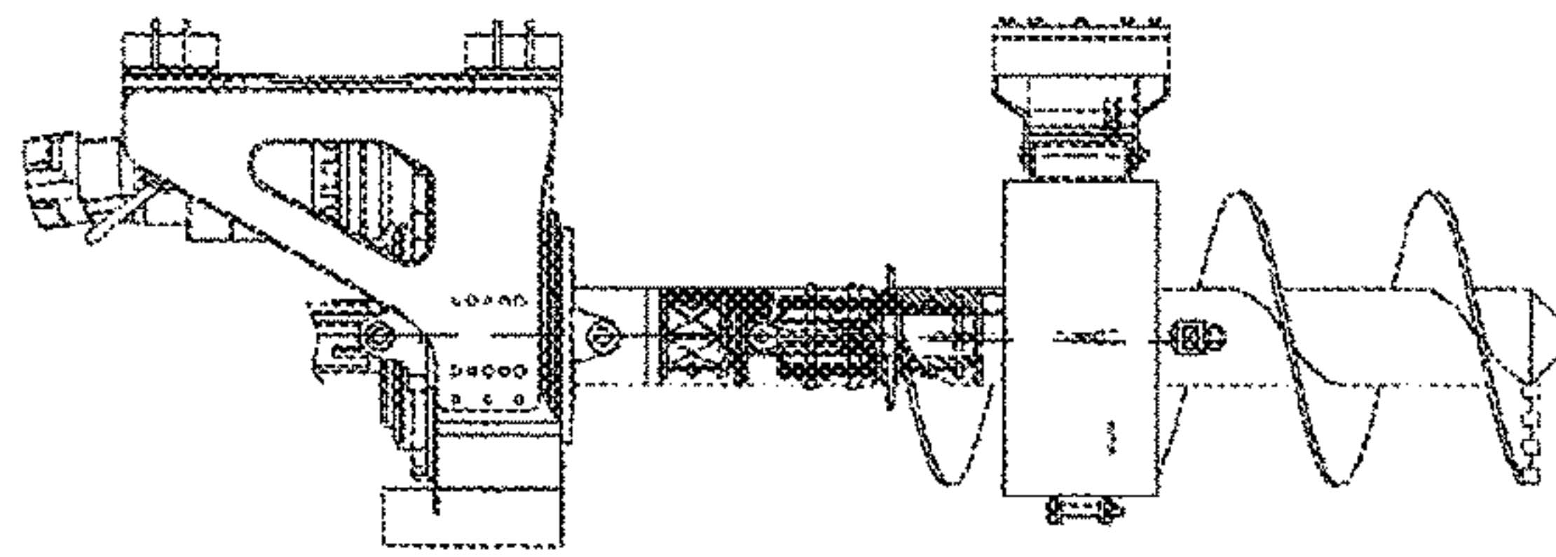
Fig. 6B
