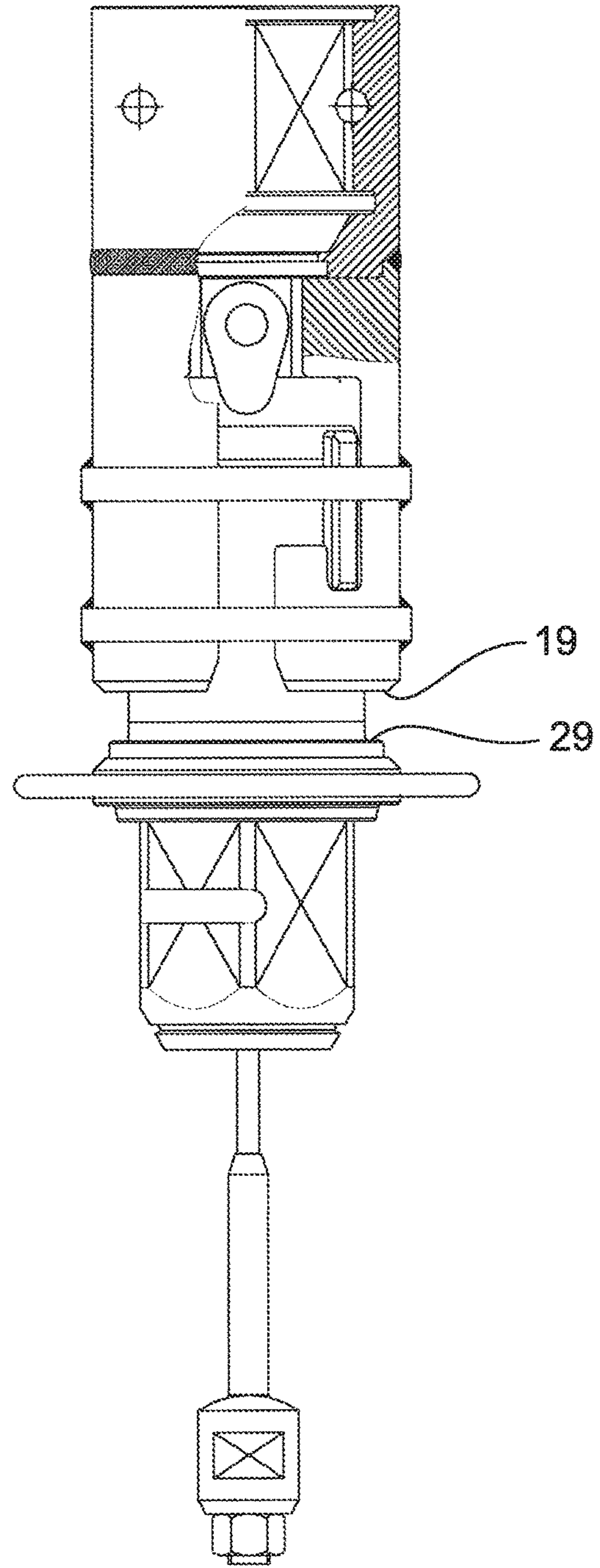
Fig. 2B
