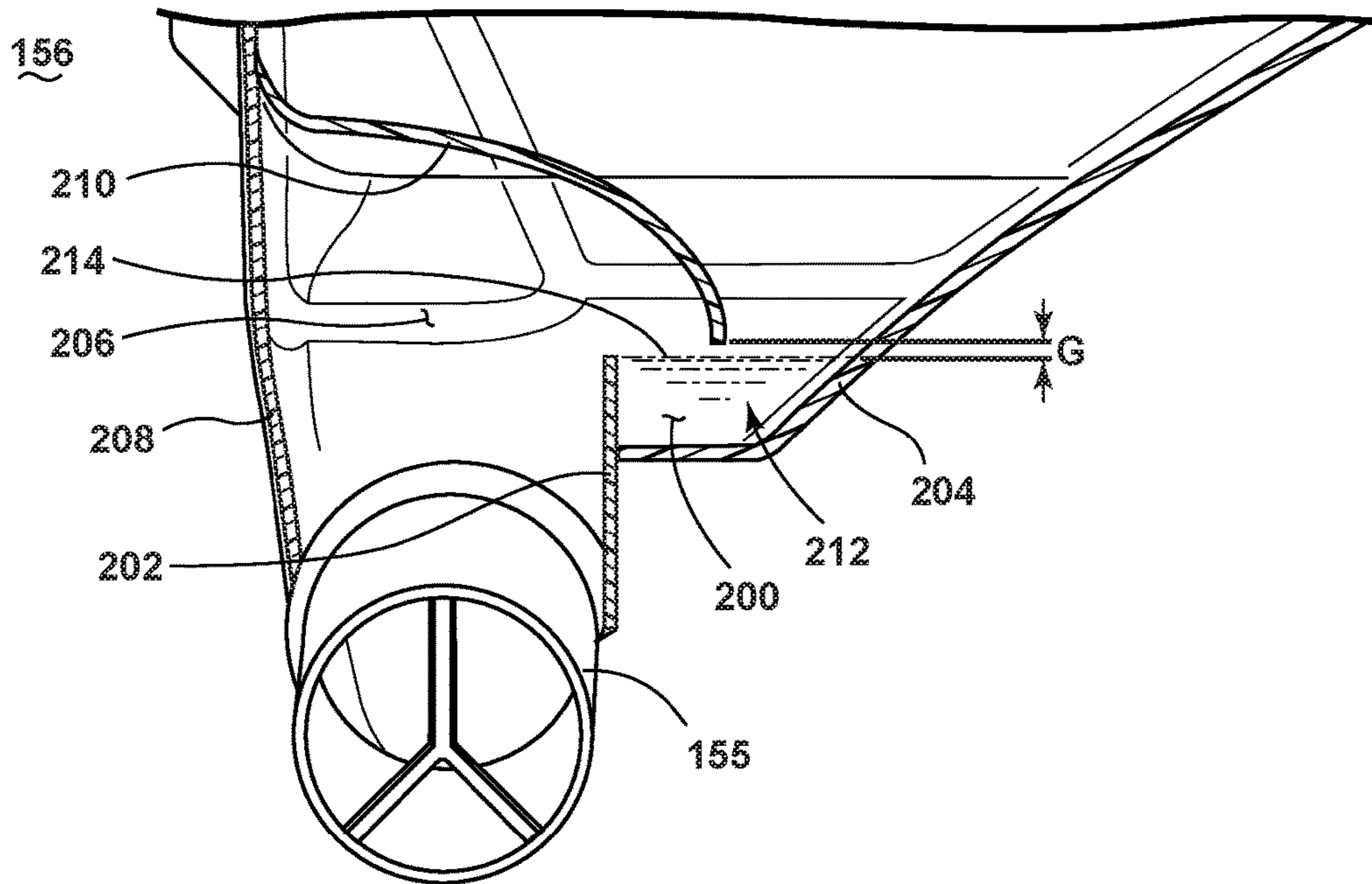
FIG. 9A
