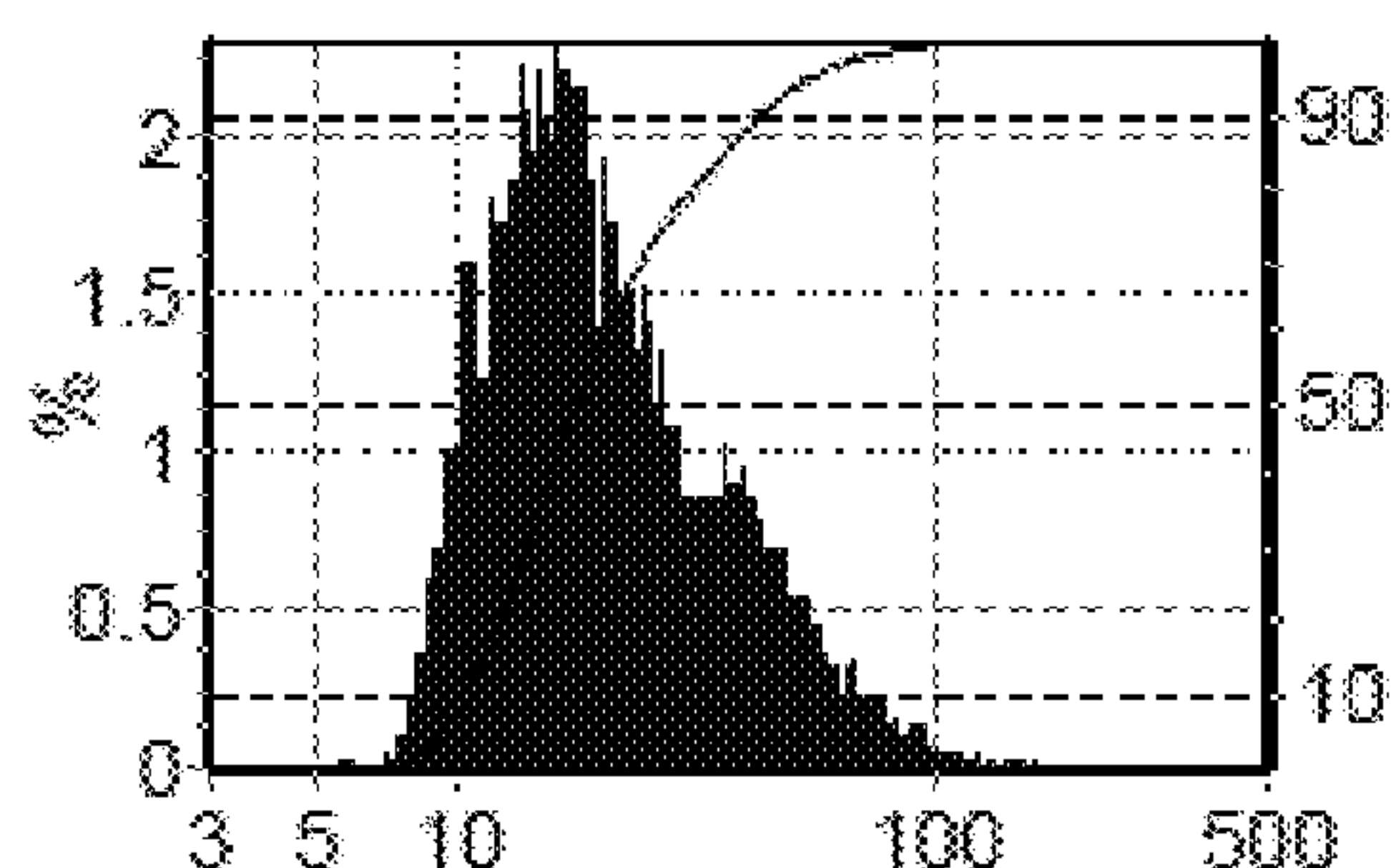
Feret Width
