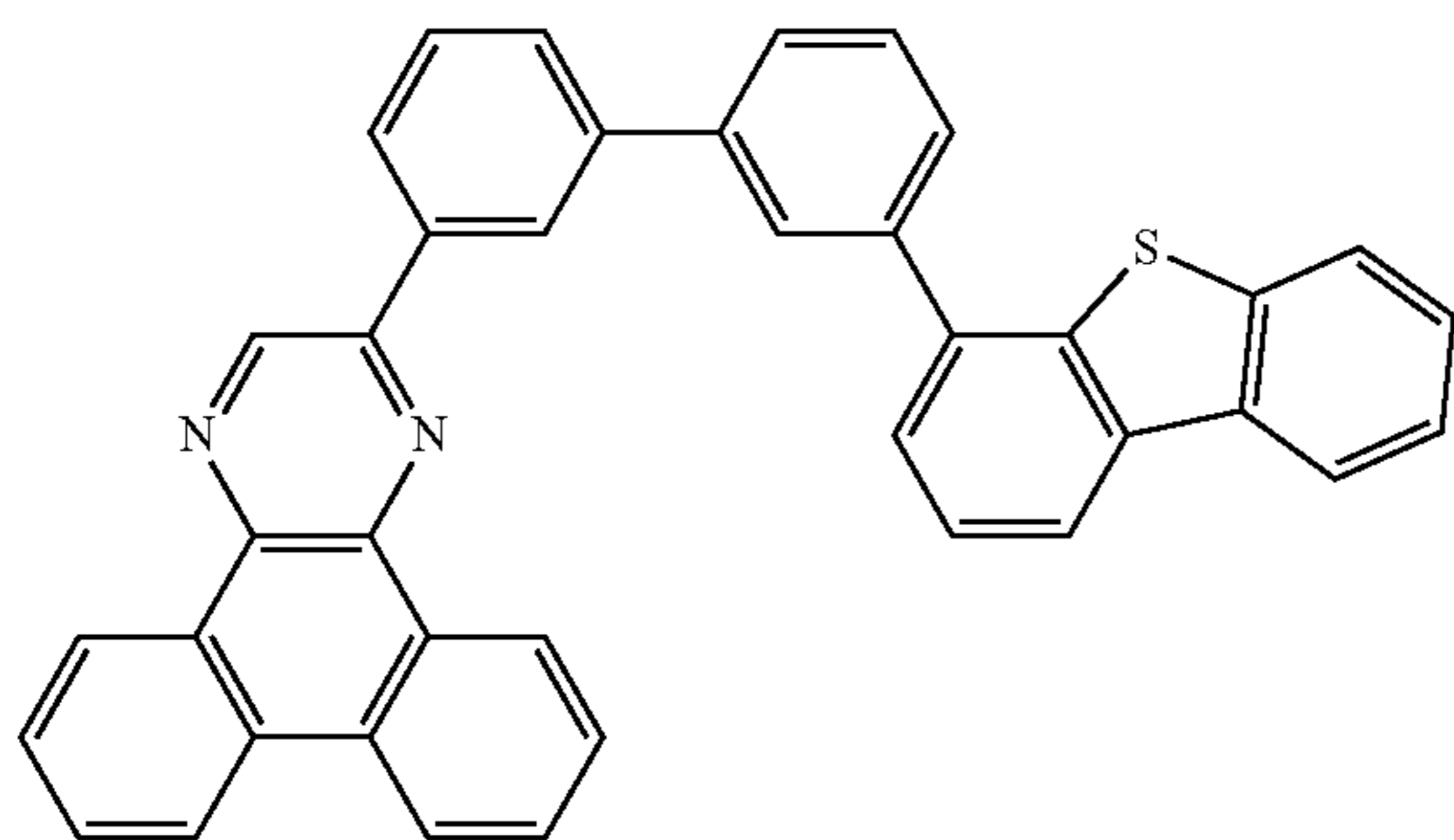
2mDBTPDBq-II
