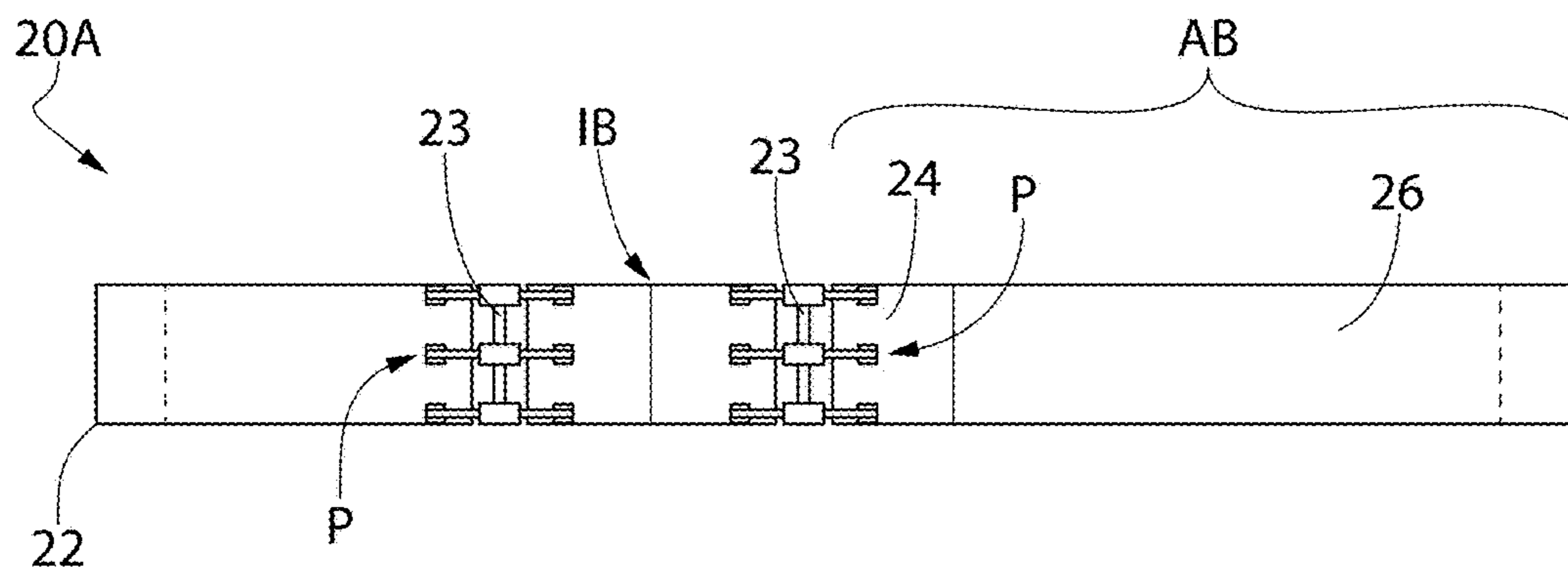
FIG. 5A
