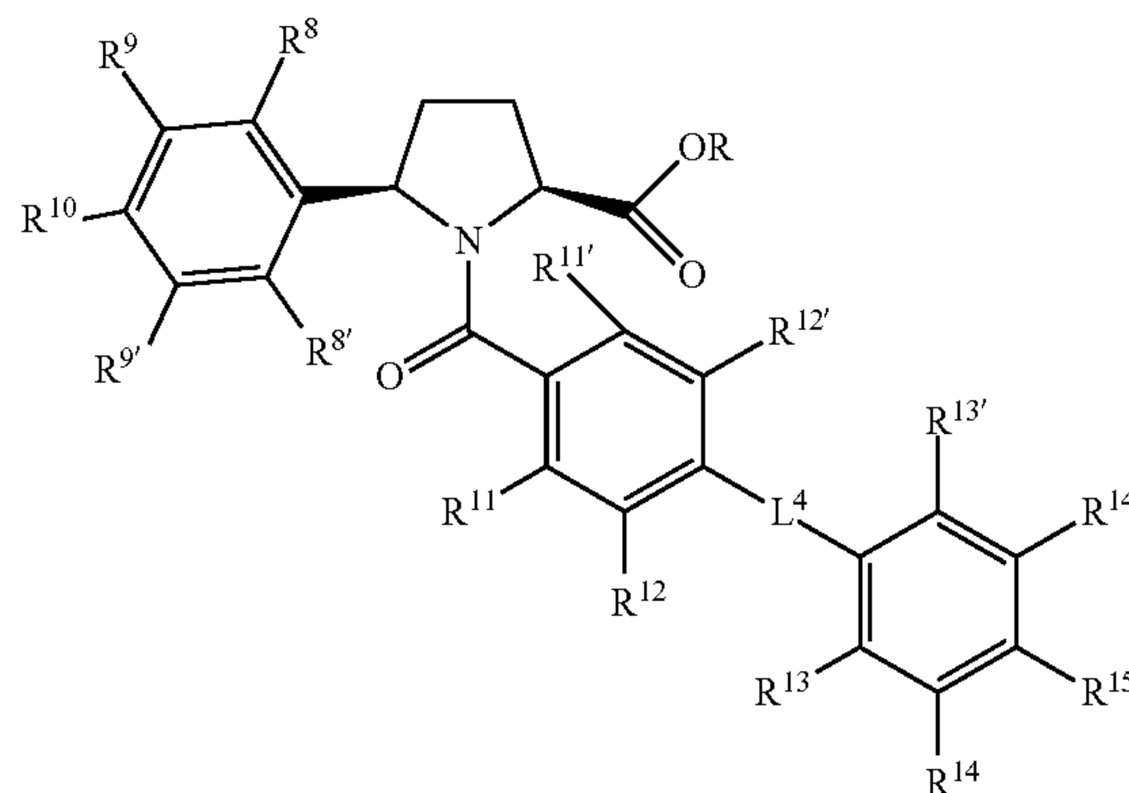
Ib-1h
