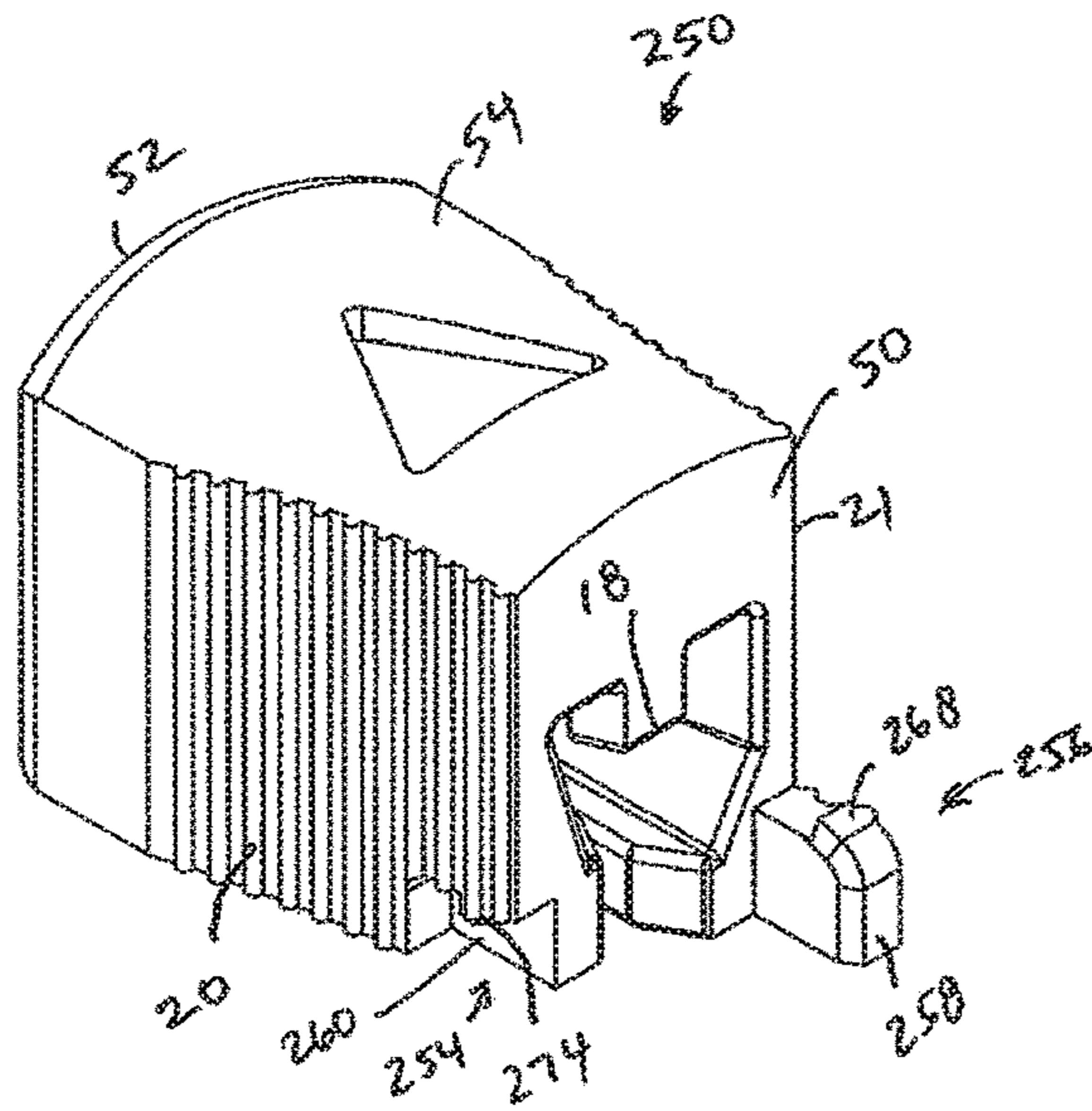
FIG. 23
