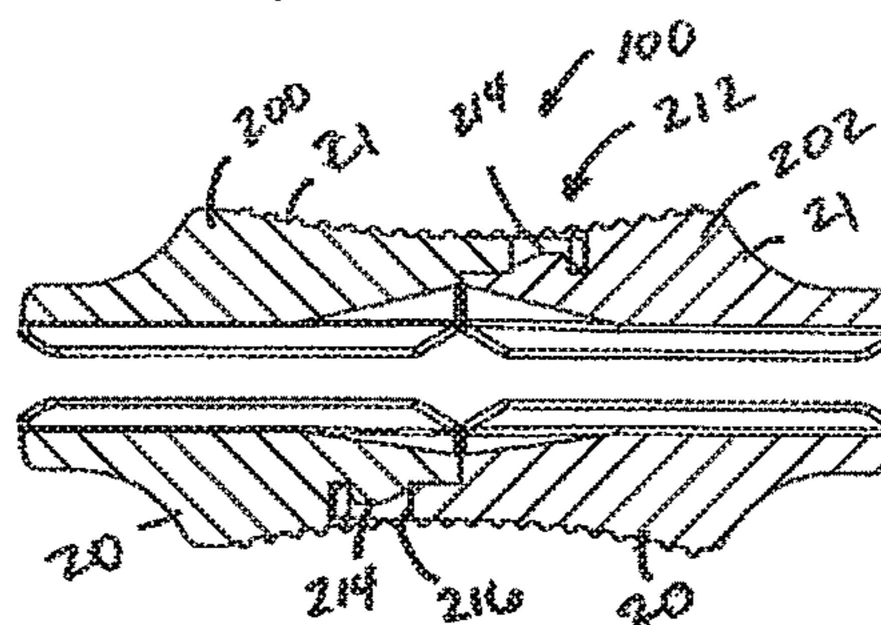
FIG. 12
