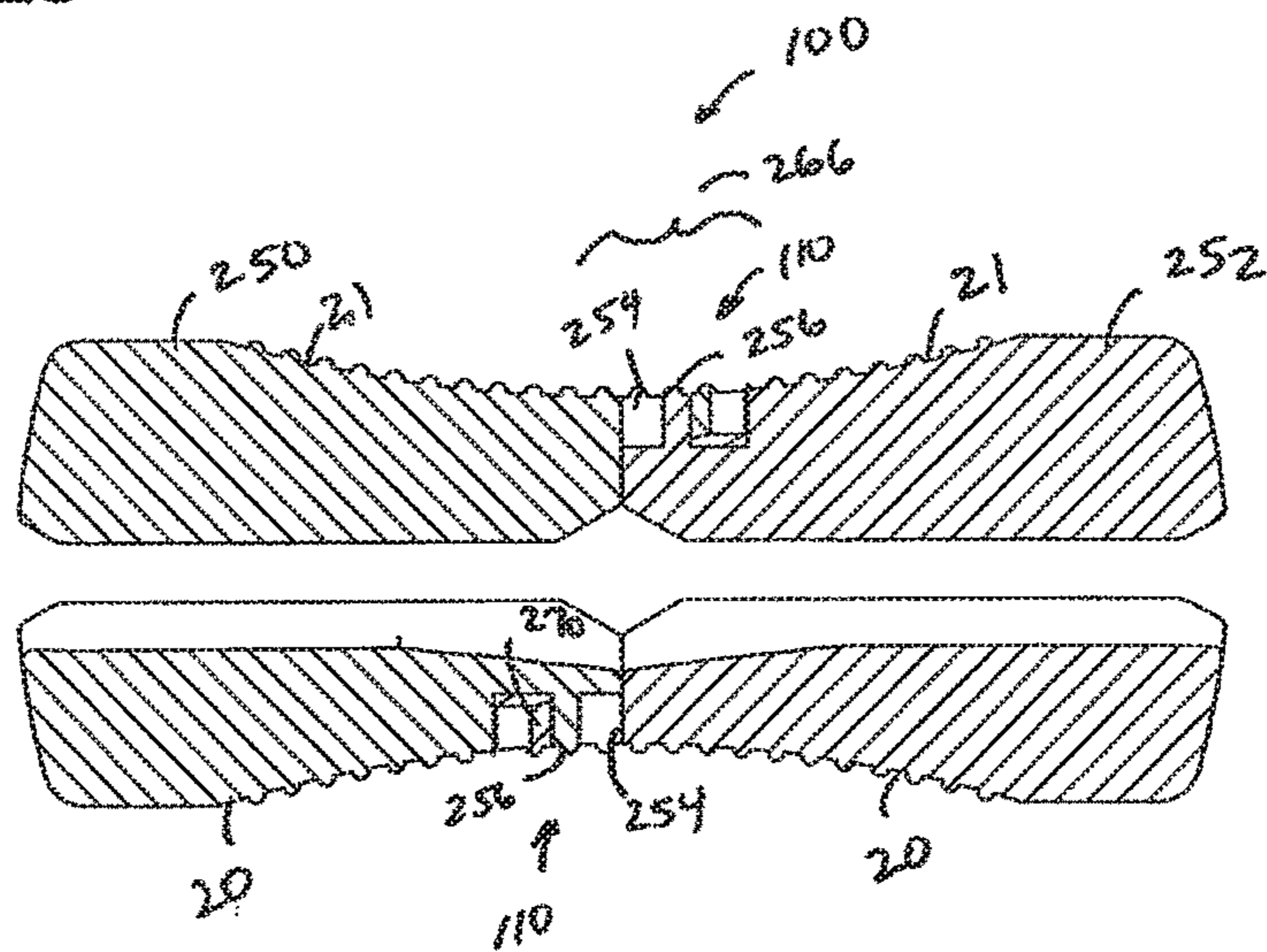
FIG. 28
