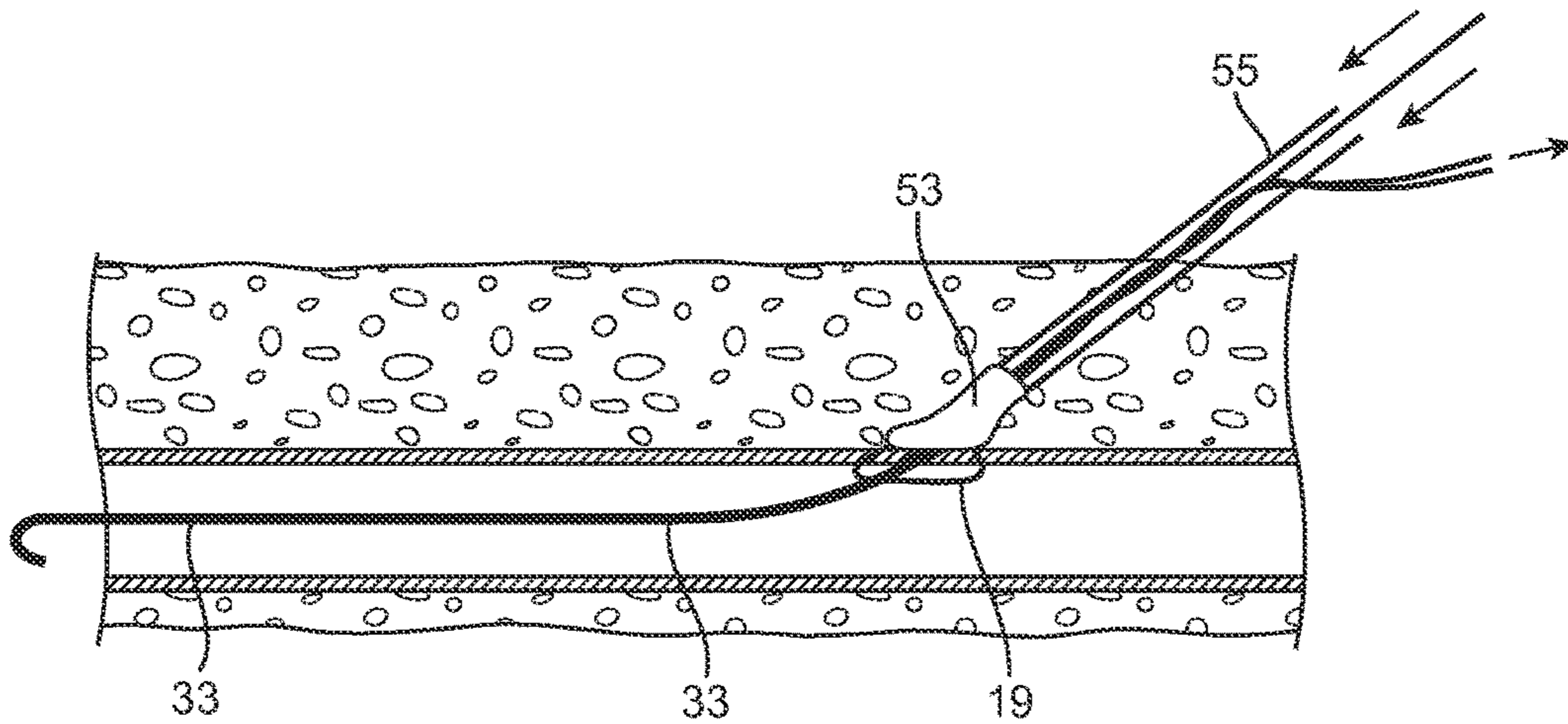
FIG. 18B
