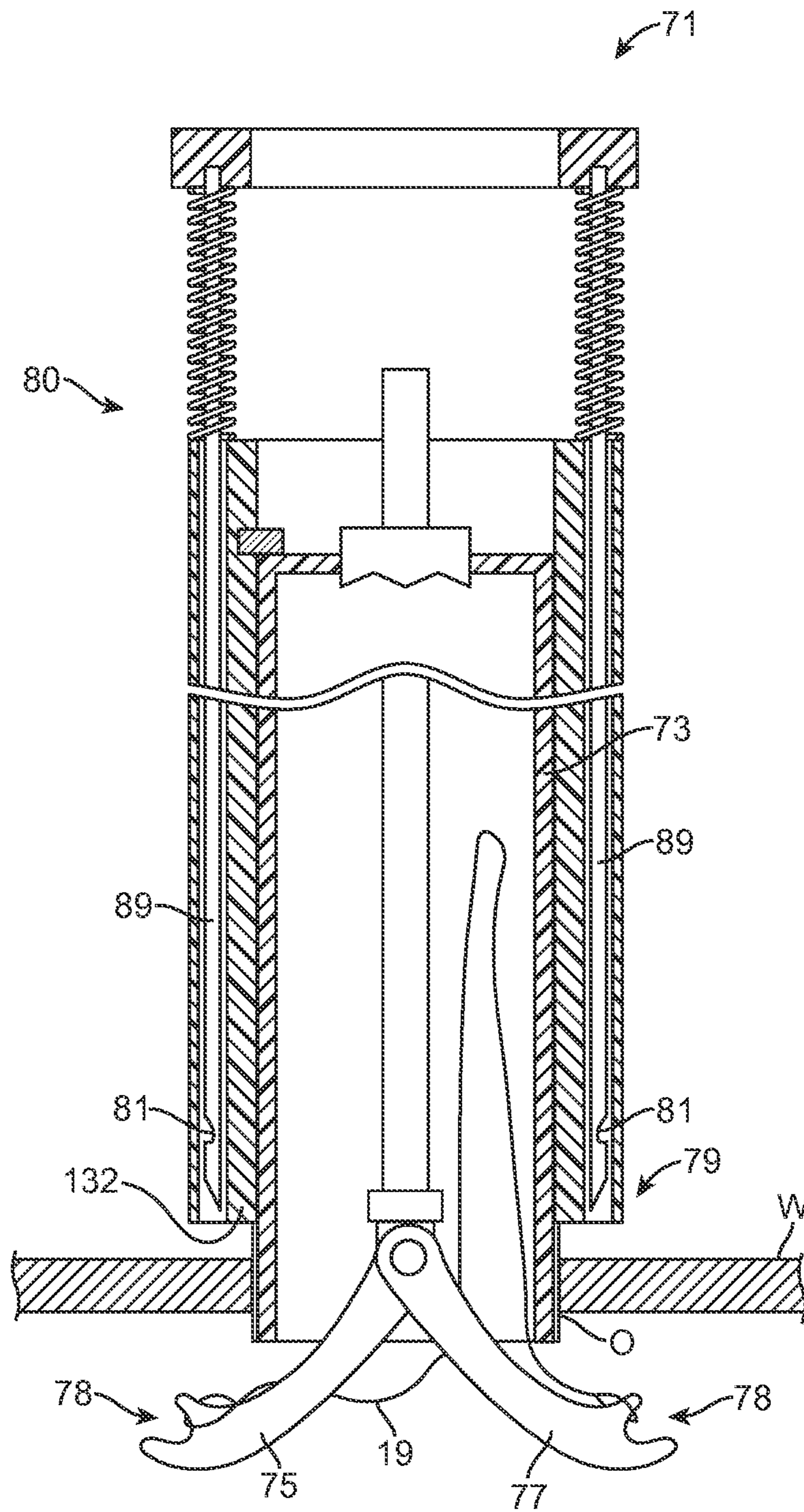
FIG. 8
