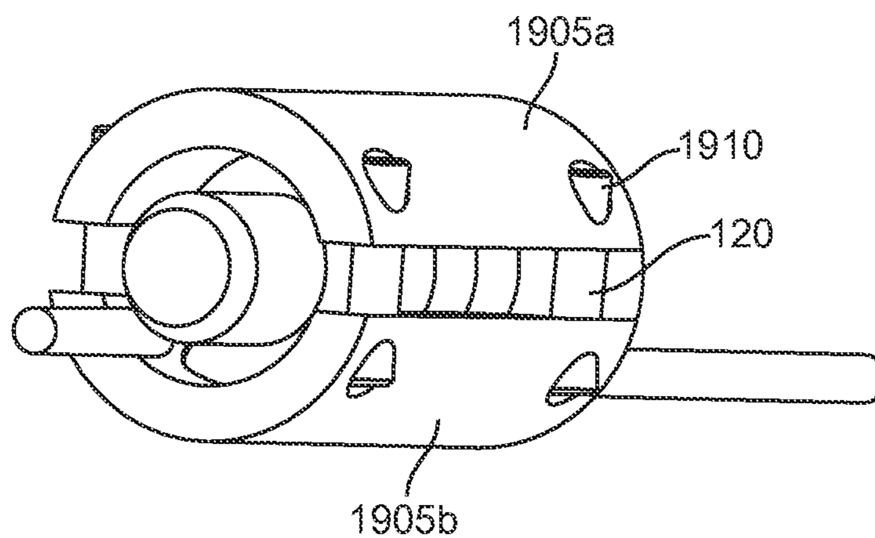
FIG. 35A
