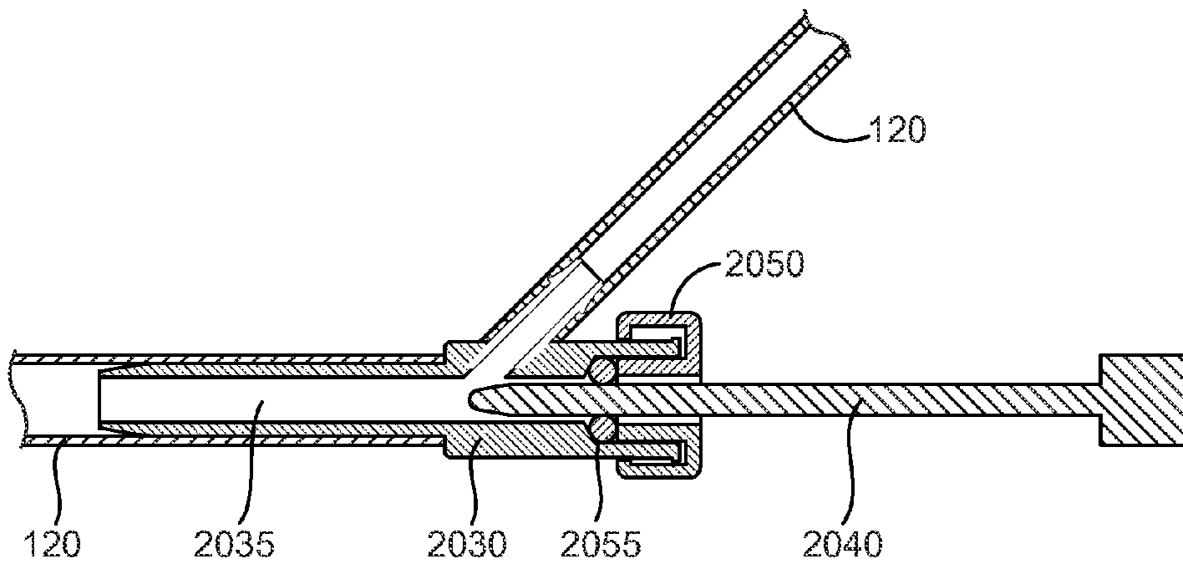
FIG. 37B
