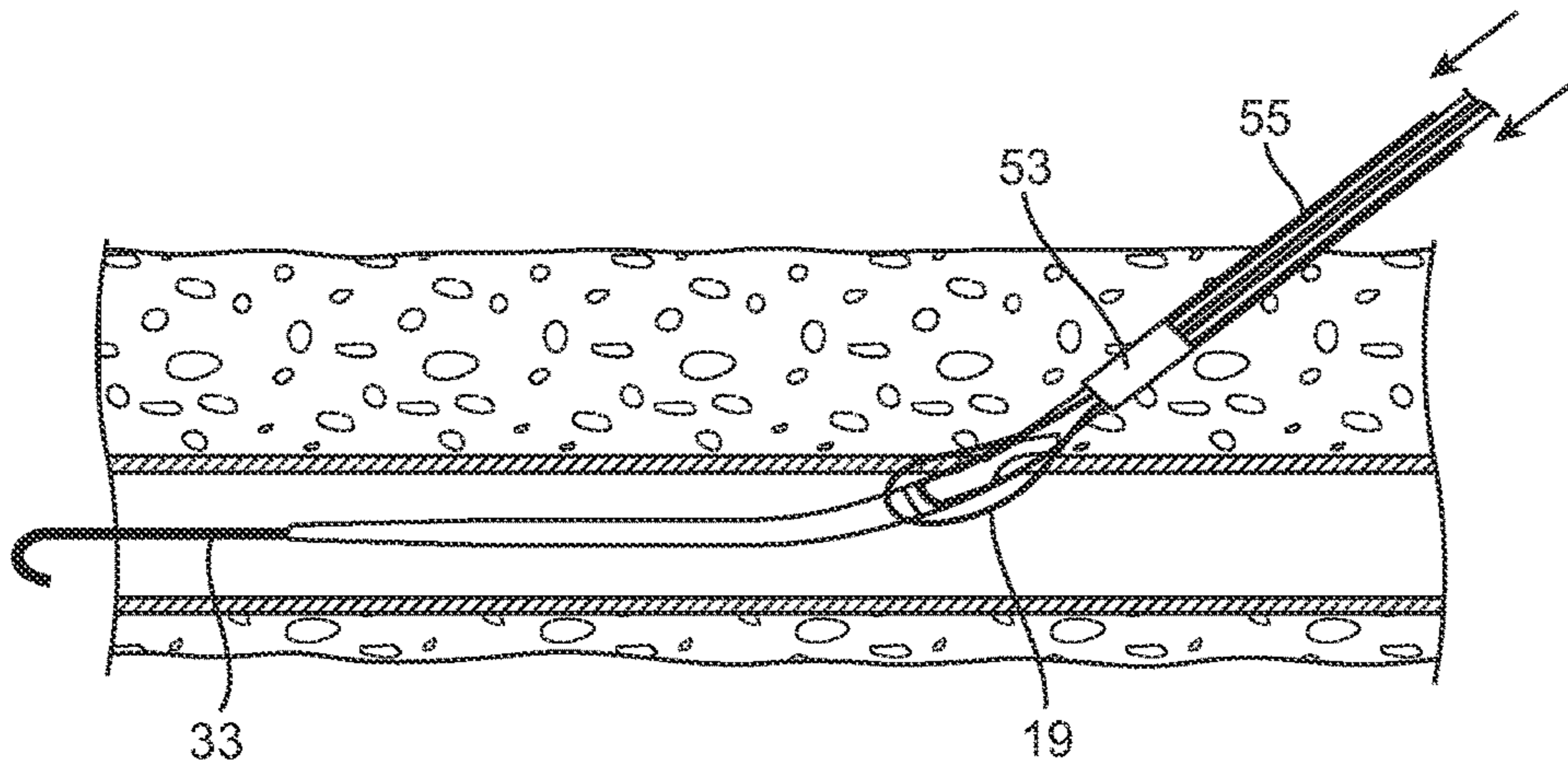
FIG. 18A
