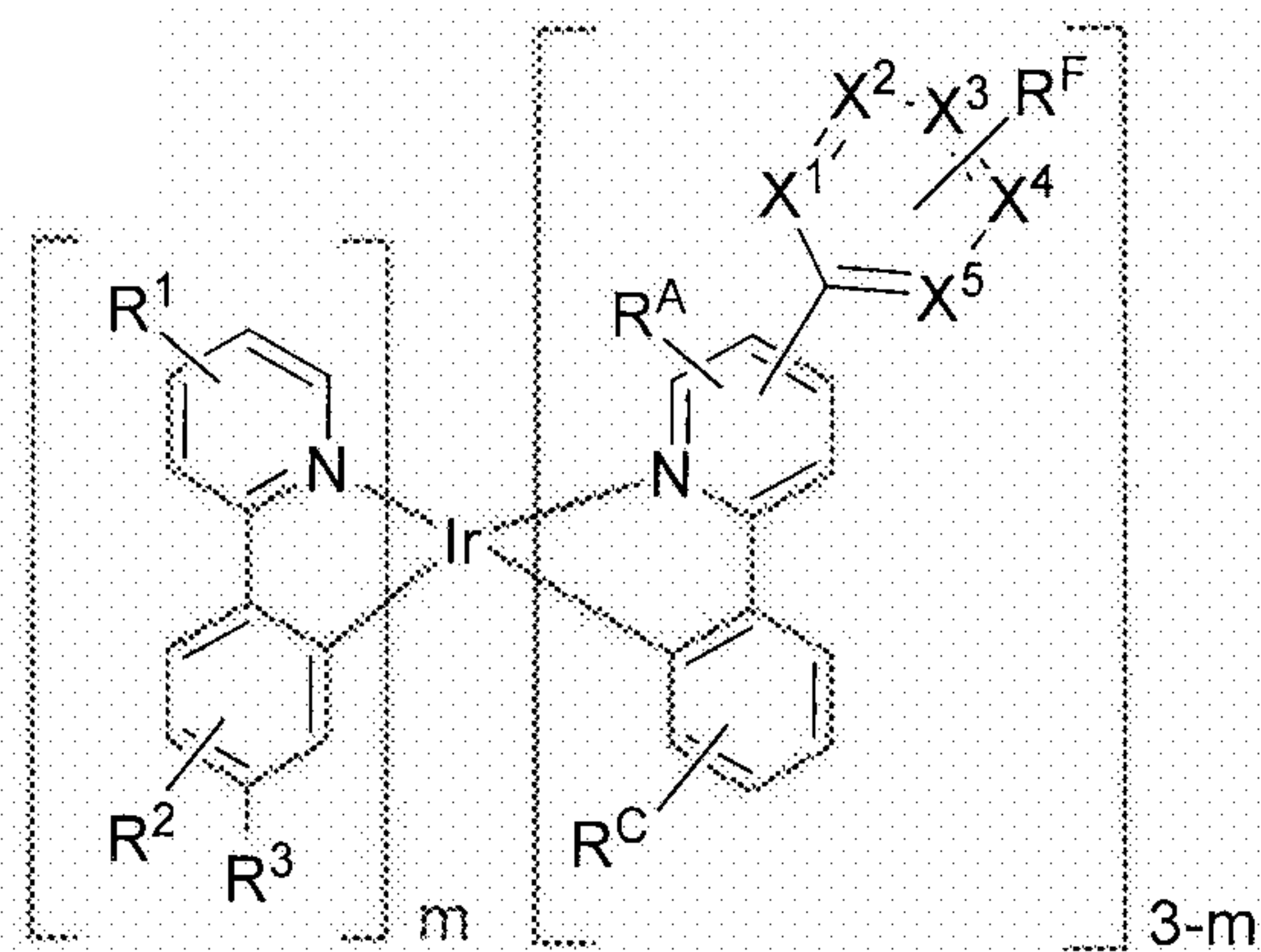
Formula I-A
