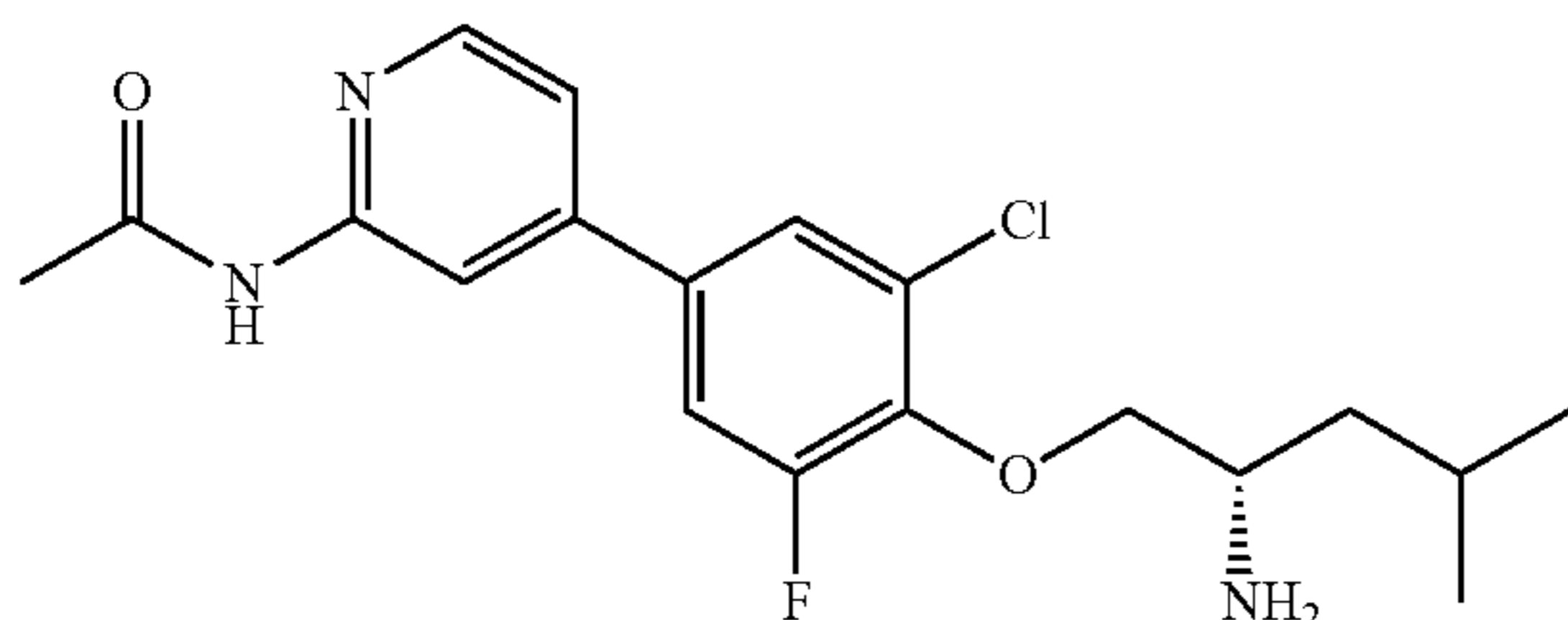
Part C: (S)-N-(4-(4-((2-amino-4-methylpentyl)oxy)-3-chloro-5-fluorophenyl)pyridin-2-yl)acetamide
