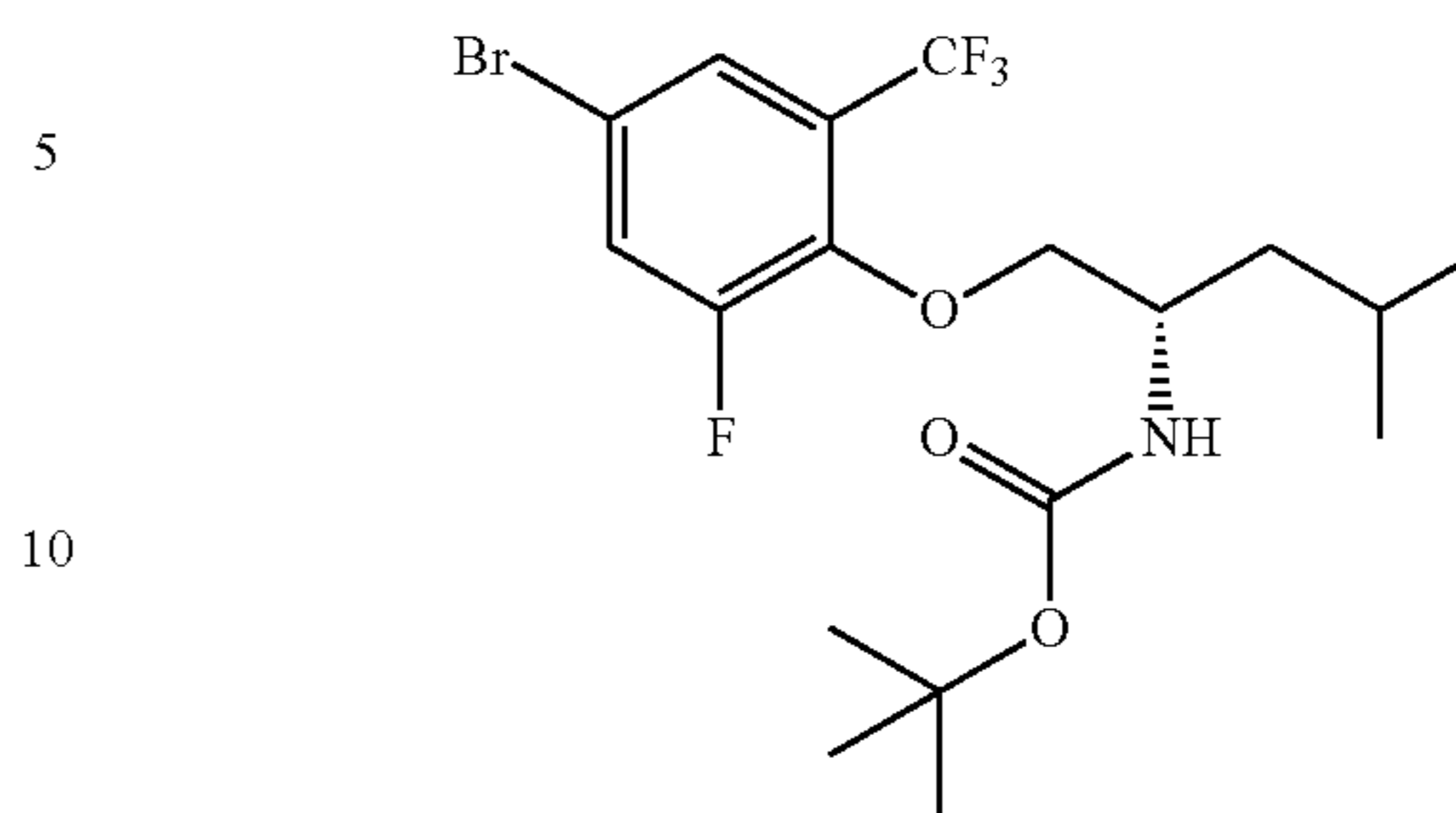
Part A: (S)-tert-butyl (1-(4-(2-amino-4-methylpentyl)oxy)-3-bromo-6-(trifluoromethyl)phenyl)pyridin-2-yl)acetamide
