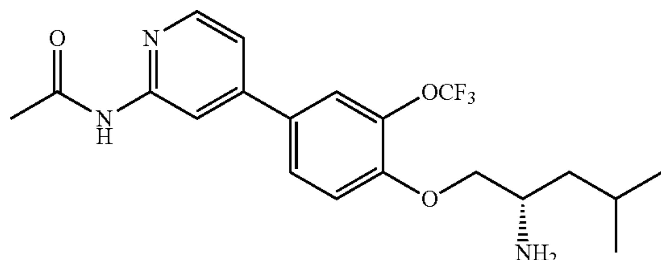
Part C: (S)-N-(4-(4-((2-amino-4-methylpentyl)oxy)-3-(trifluoromethoxy)phenyl)pyridin-2-yl)acetamide
