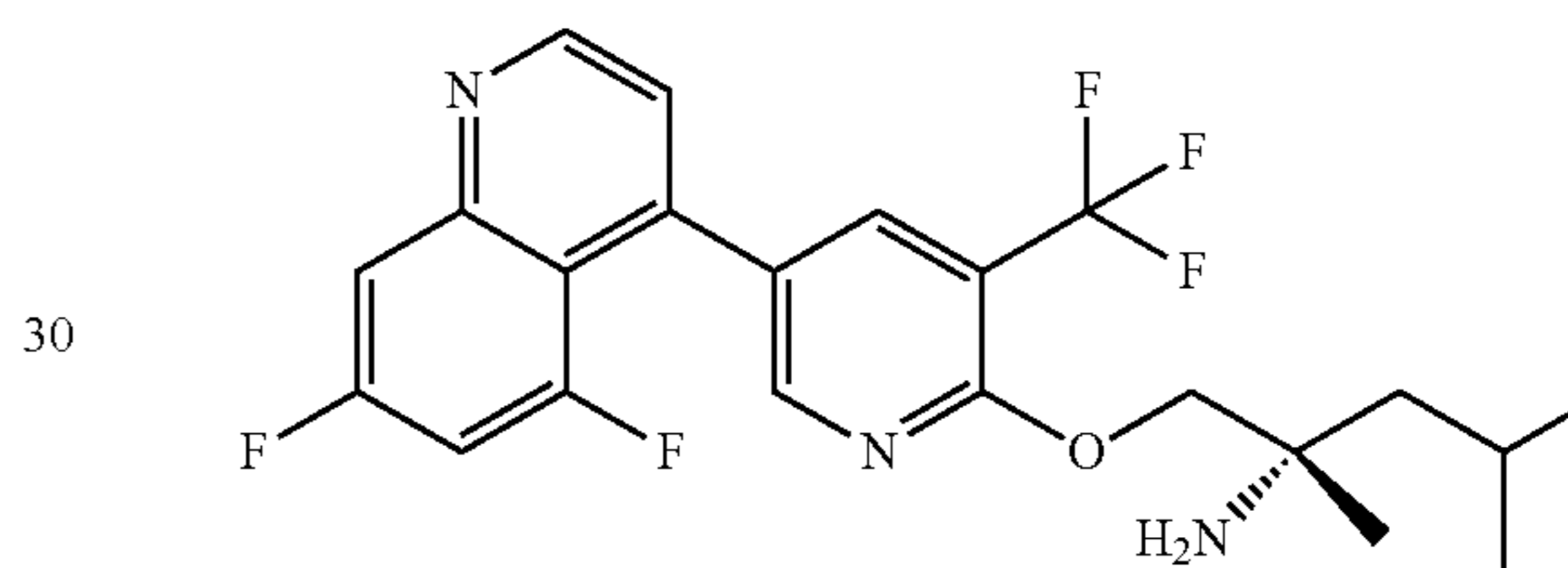
Part D: (S)-1-((5-(5,7-difluoroquinolin-4-yl)-3-(trifluoromethyl)pyridin-2-yl)oxy)-2,4-dimethylpentan-2-amine
