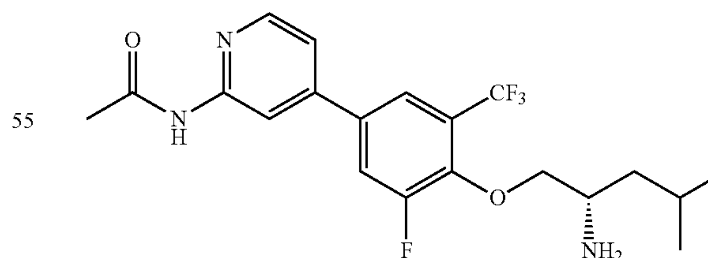
Part C: (S)-N-(4-(4-((2-amino-4-methylpentyl)oxy)-3-fluoro-5-(trifluoromethyl)phenyl)pyridin-2-yl)acetamide
