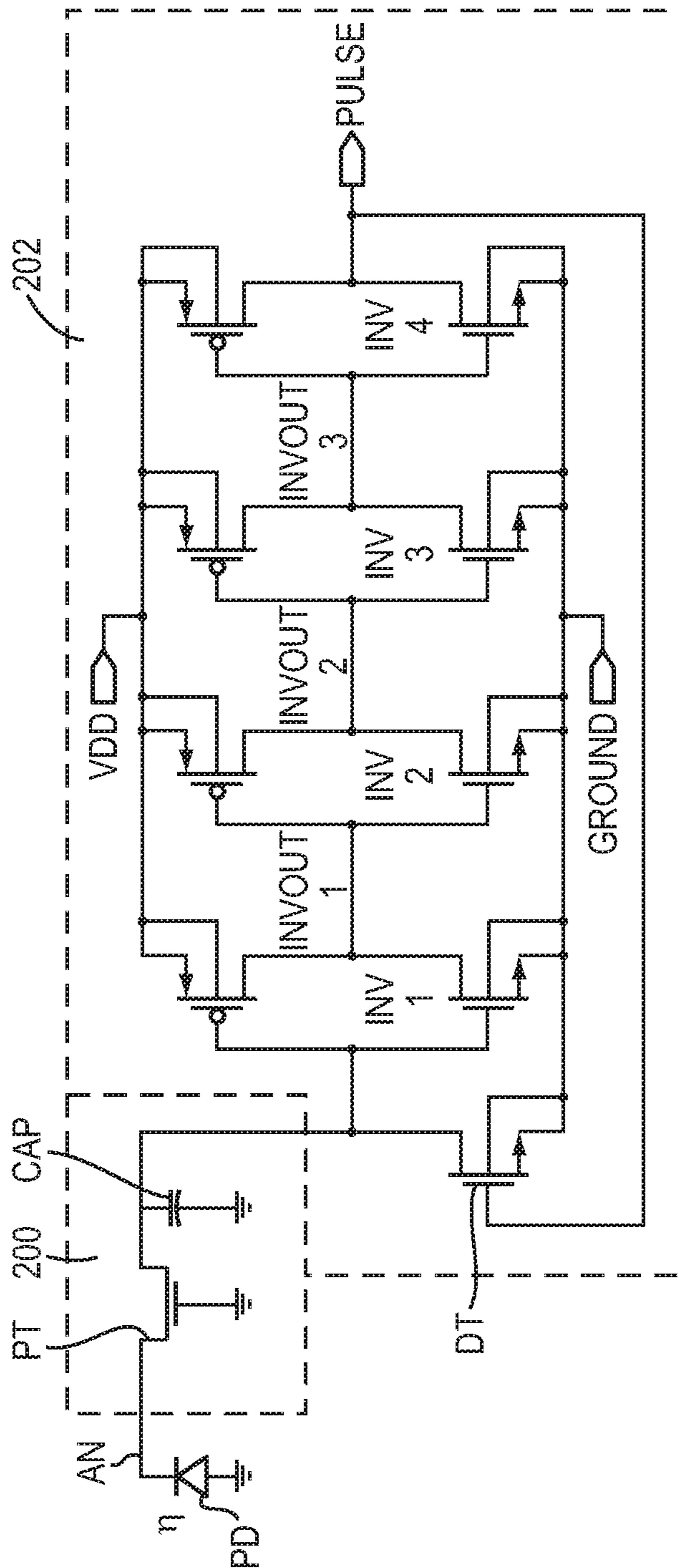
FIG. 3
