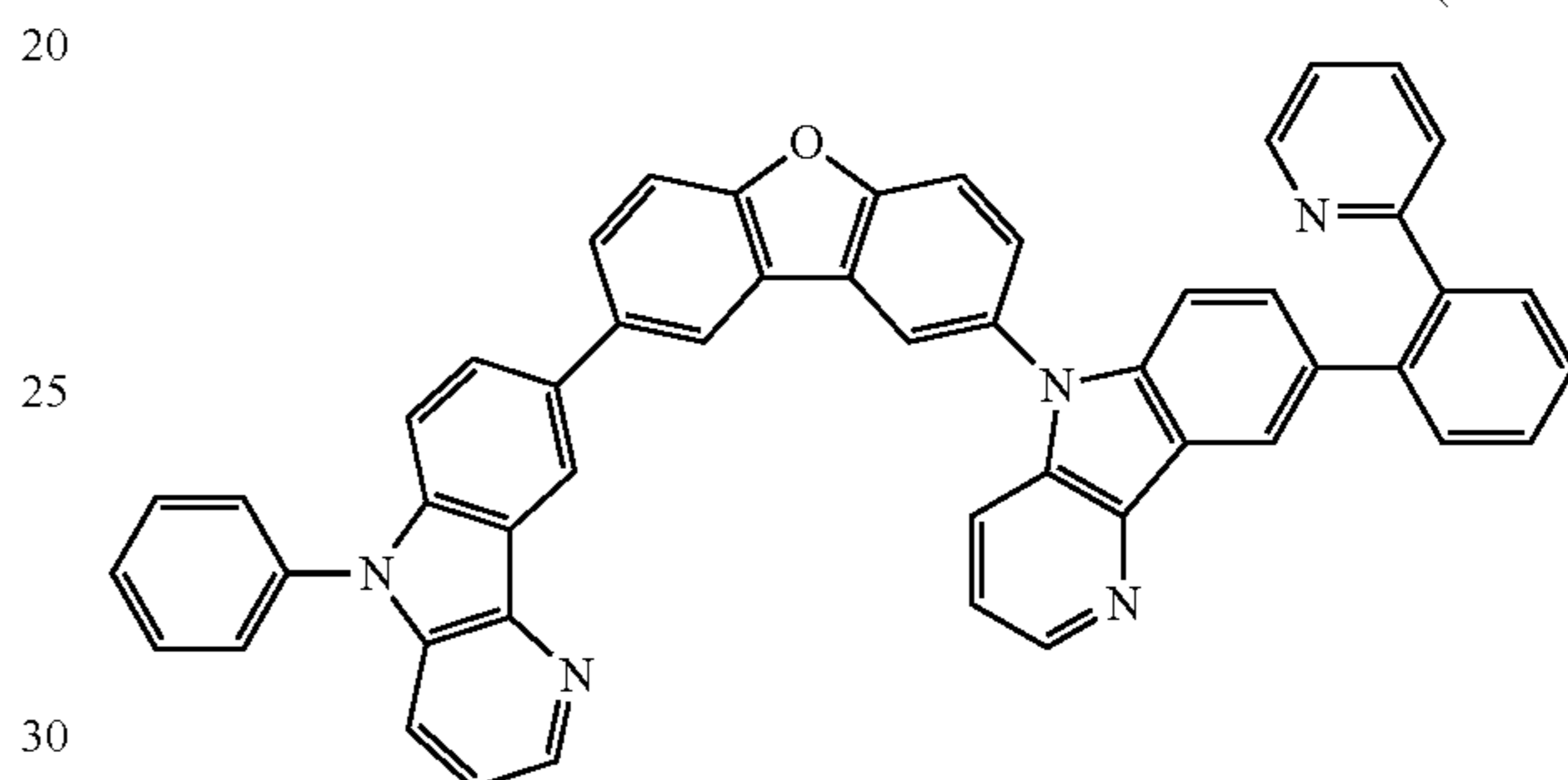
(ETM-5)
