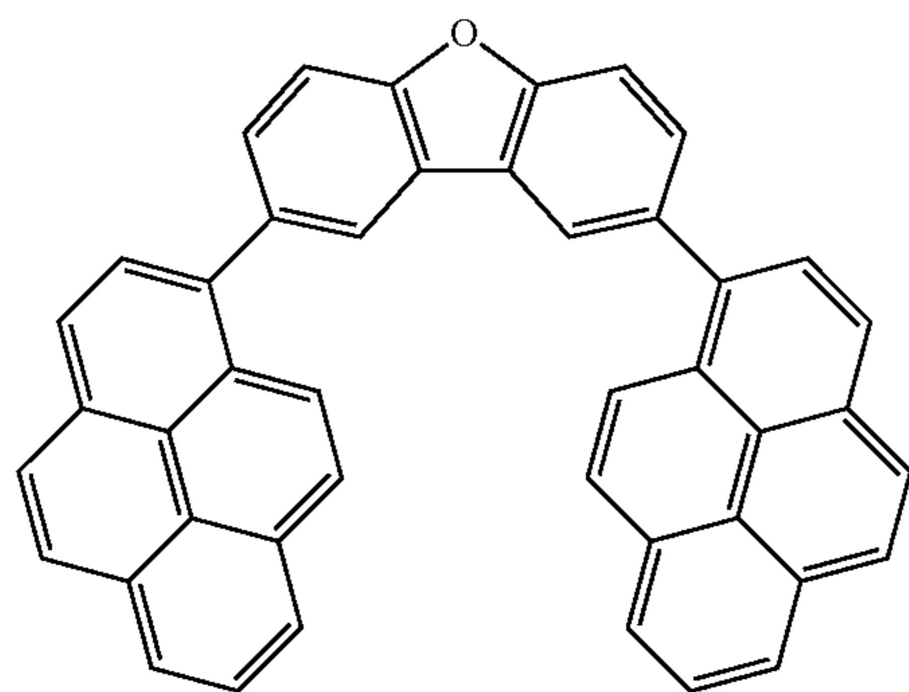
(A-10; = ETM-1)
