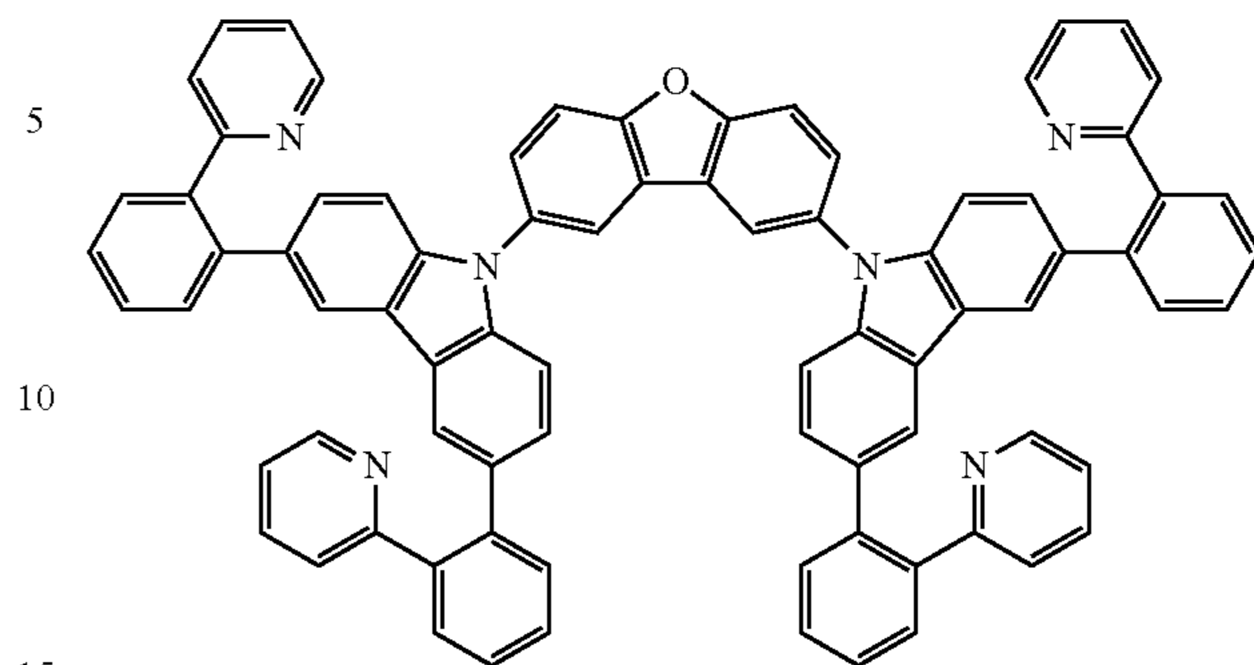
(ETM-4)
