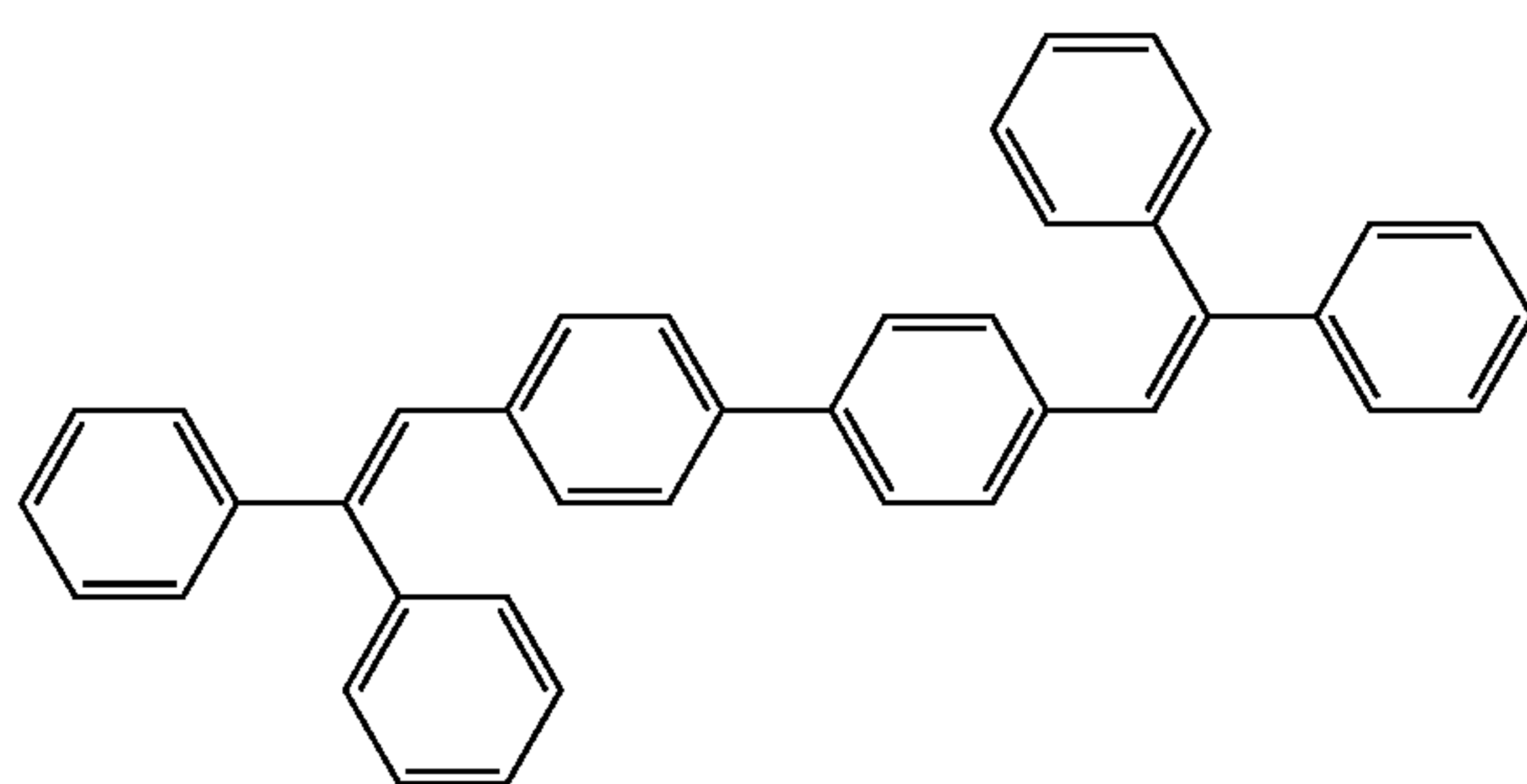
(DPVBi)
