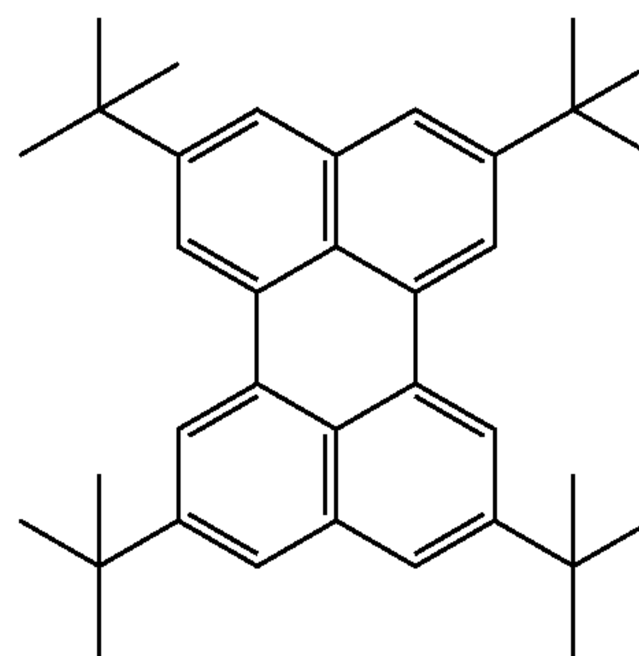
(Tetra-tert-butyl perylene)
