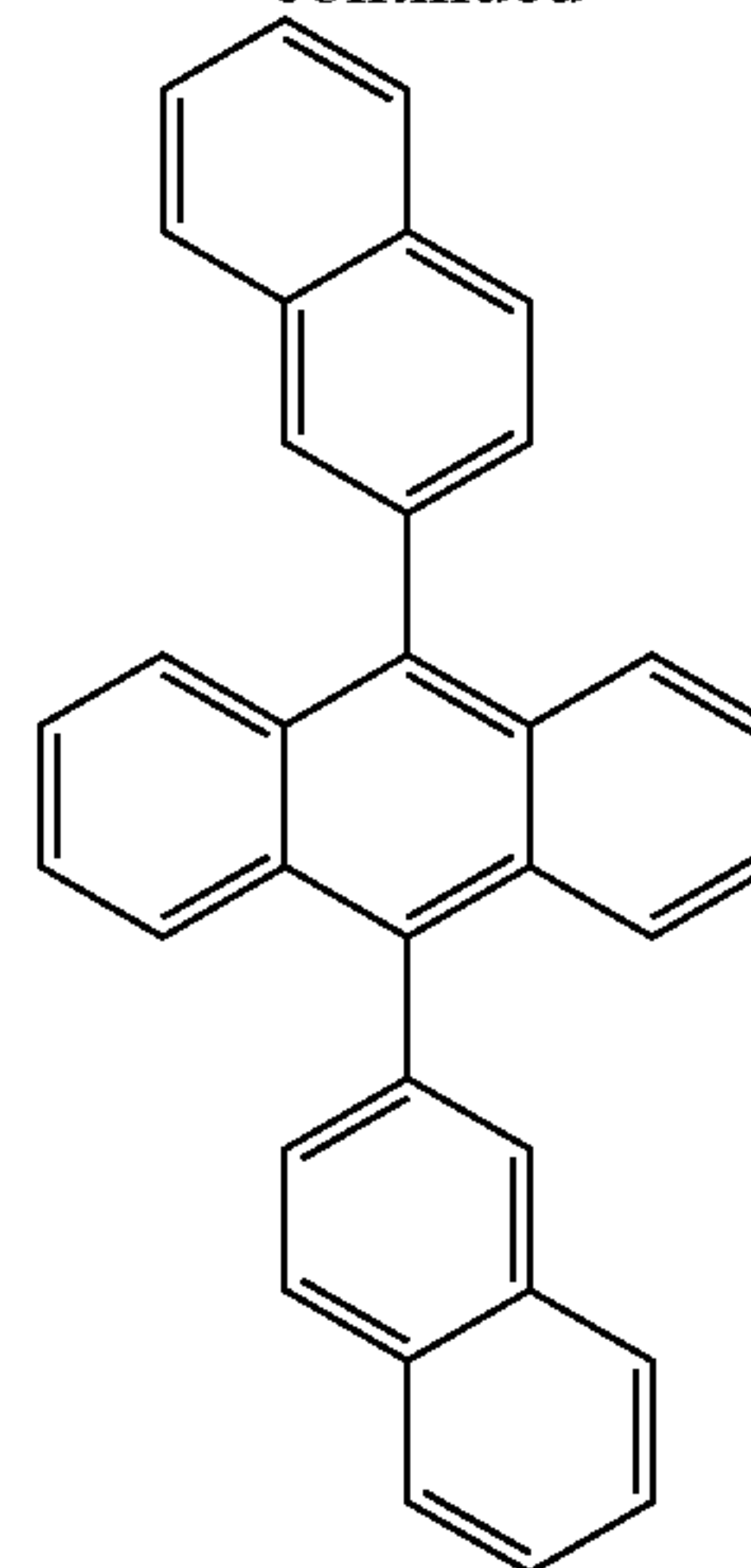
(ADN)
