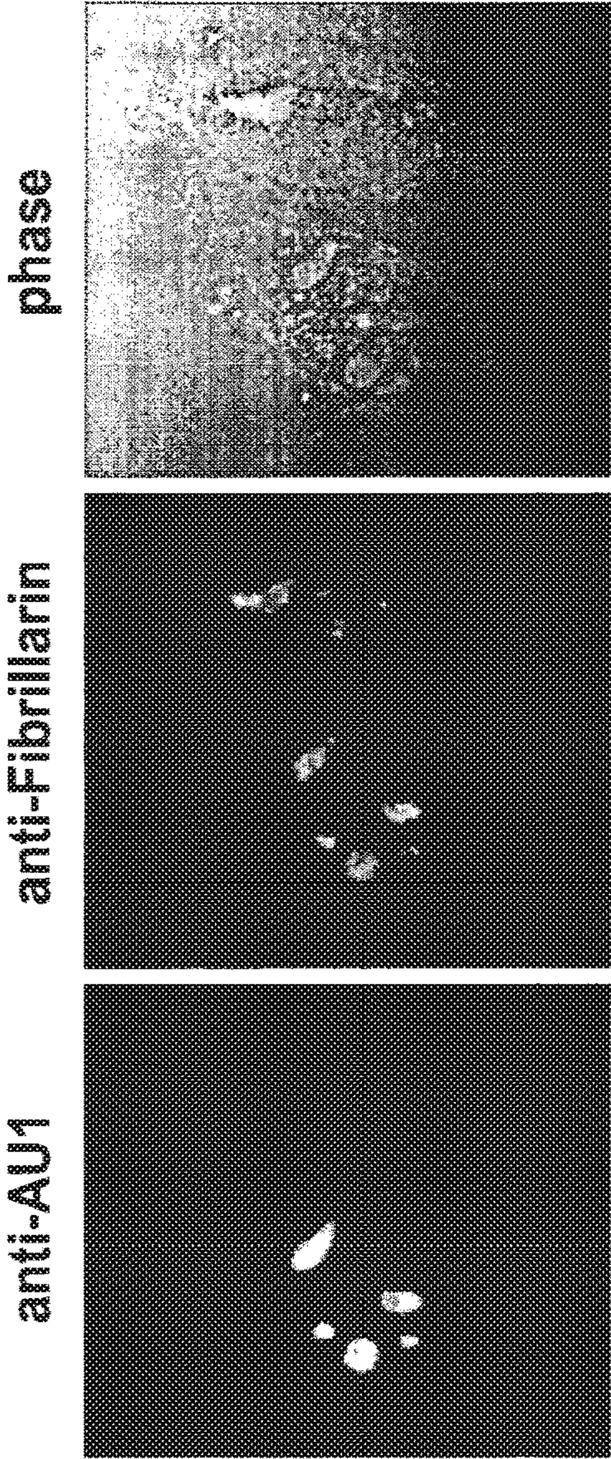
Fig. 25C pCMV-VP3/2809 + pORF2/ATG-AU1
