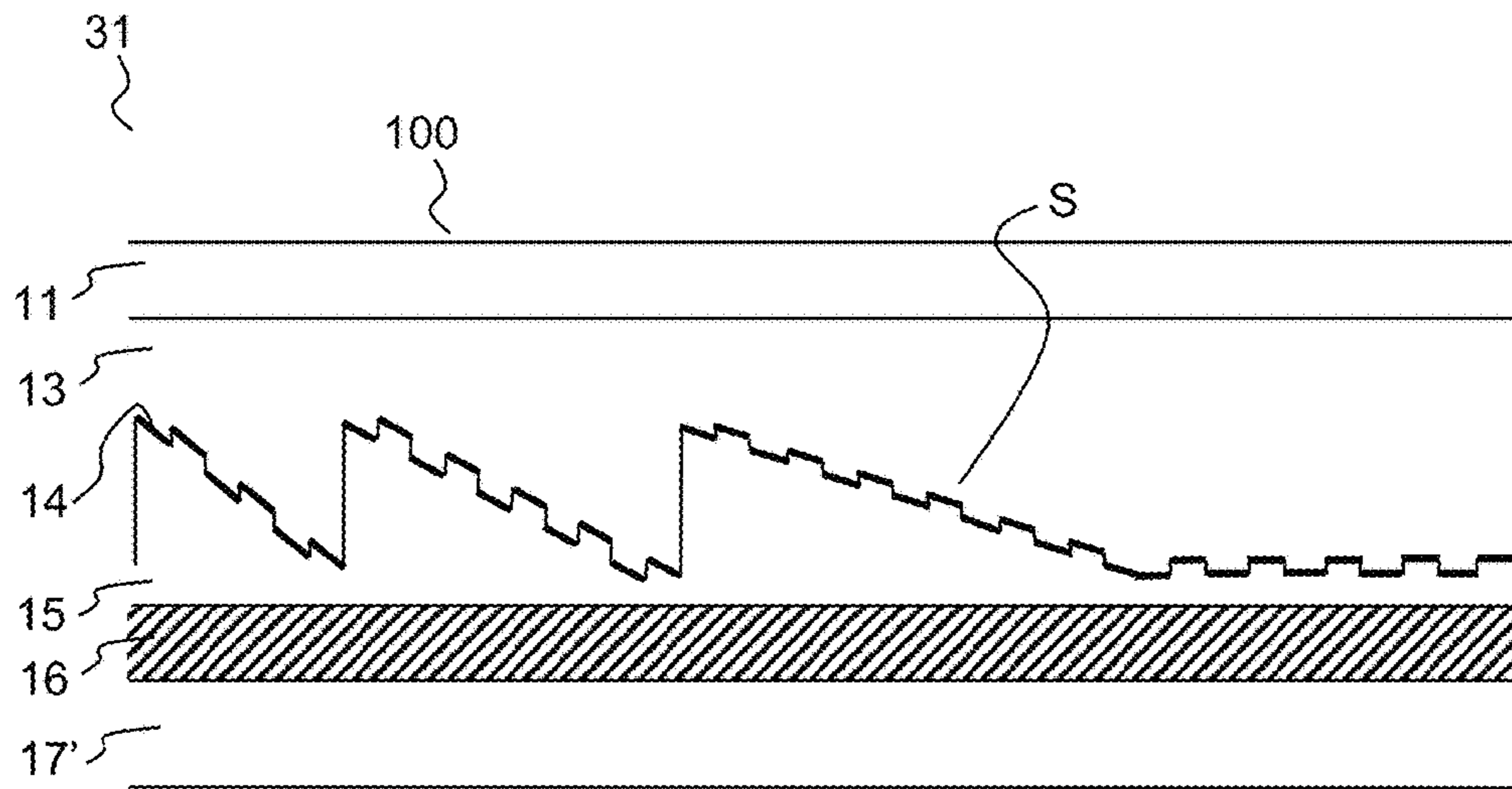
FIG.3B
