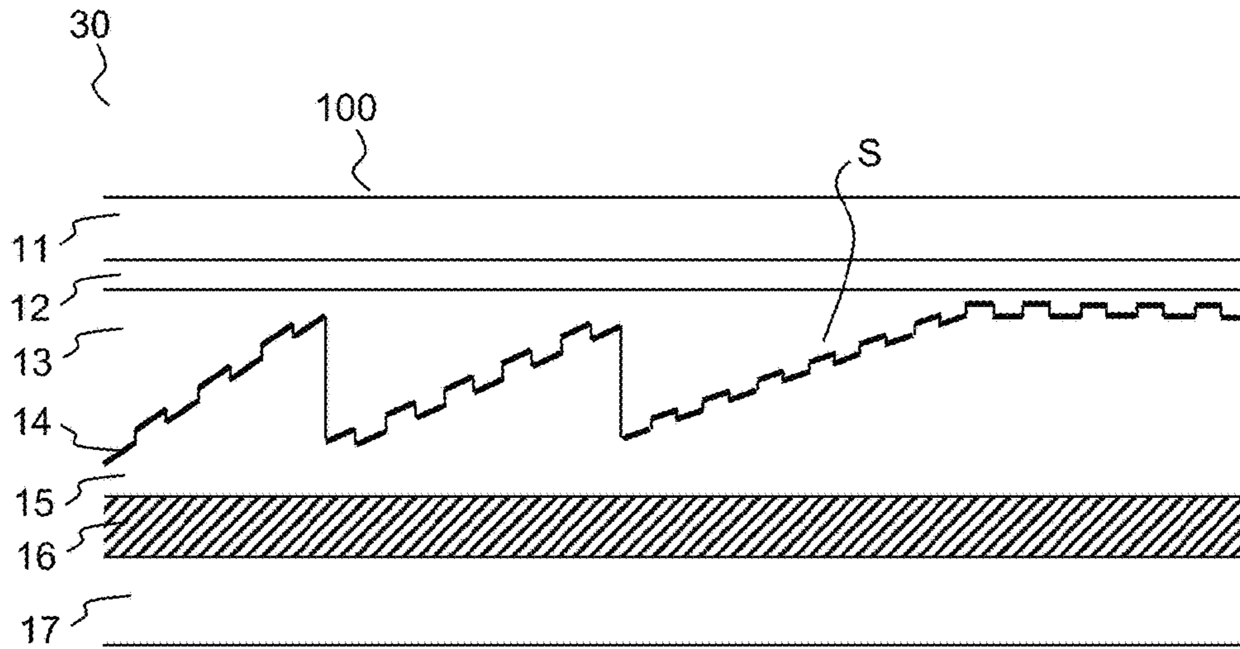
FIG.3A
