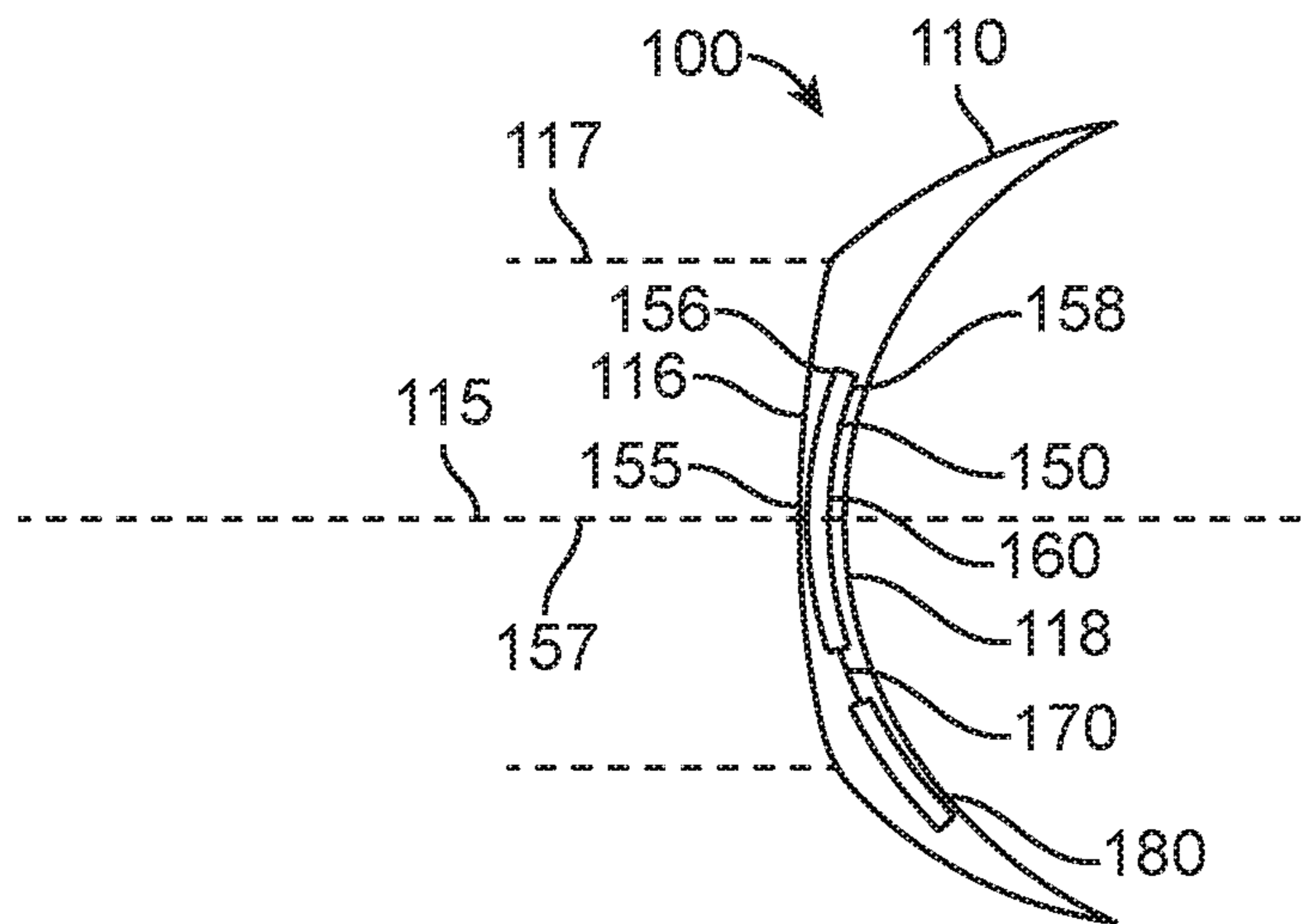
FIG. 4D
