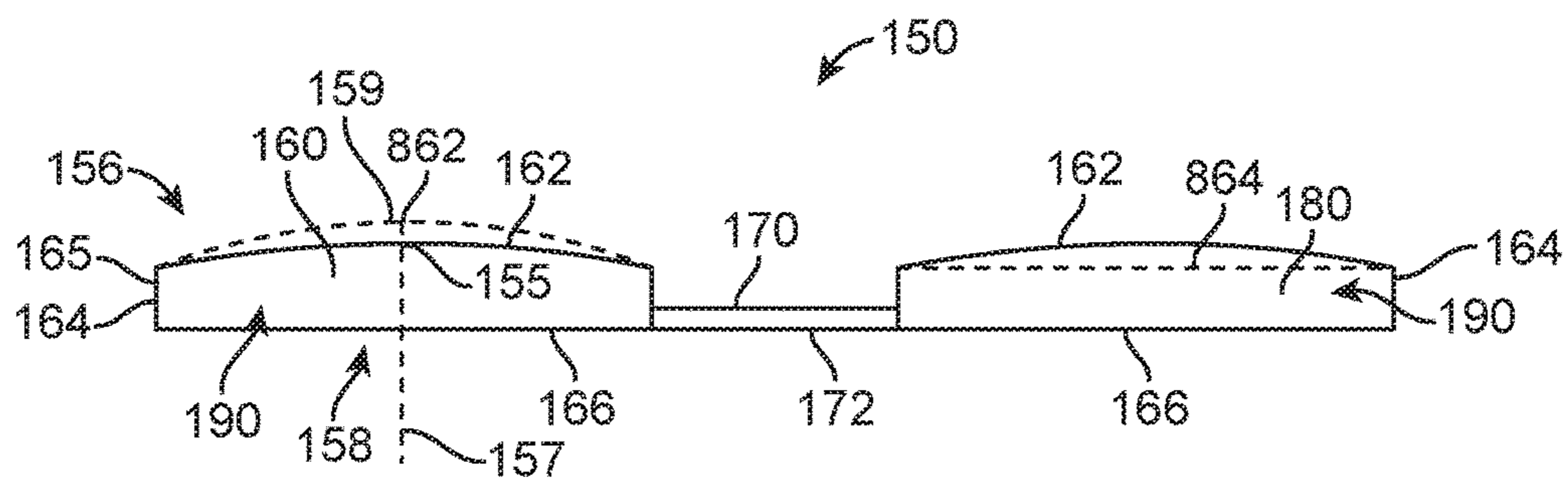
FIG. 8
