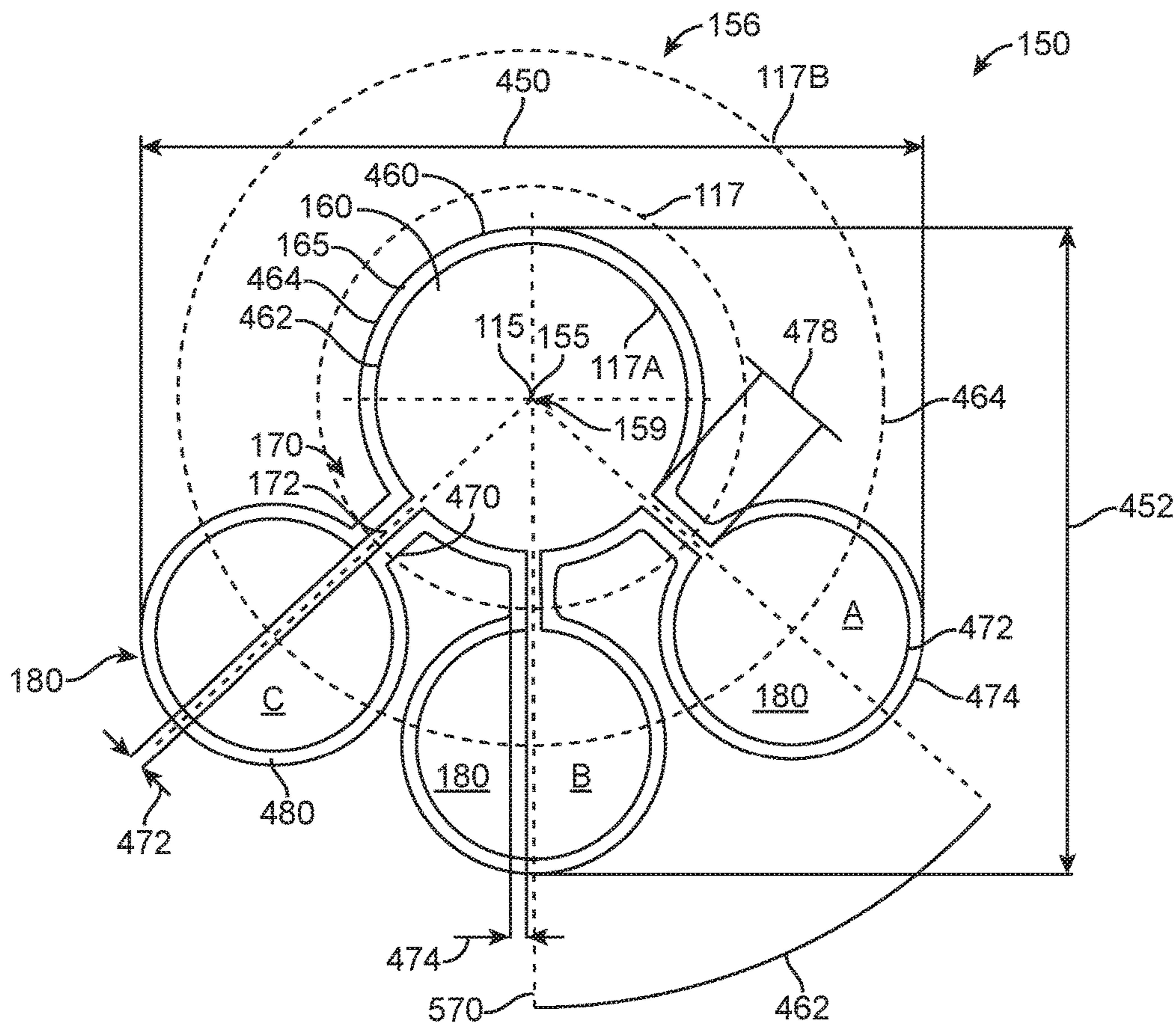
FIG. 4A
