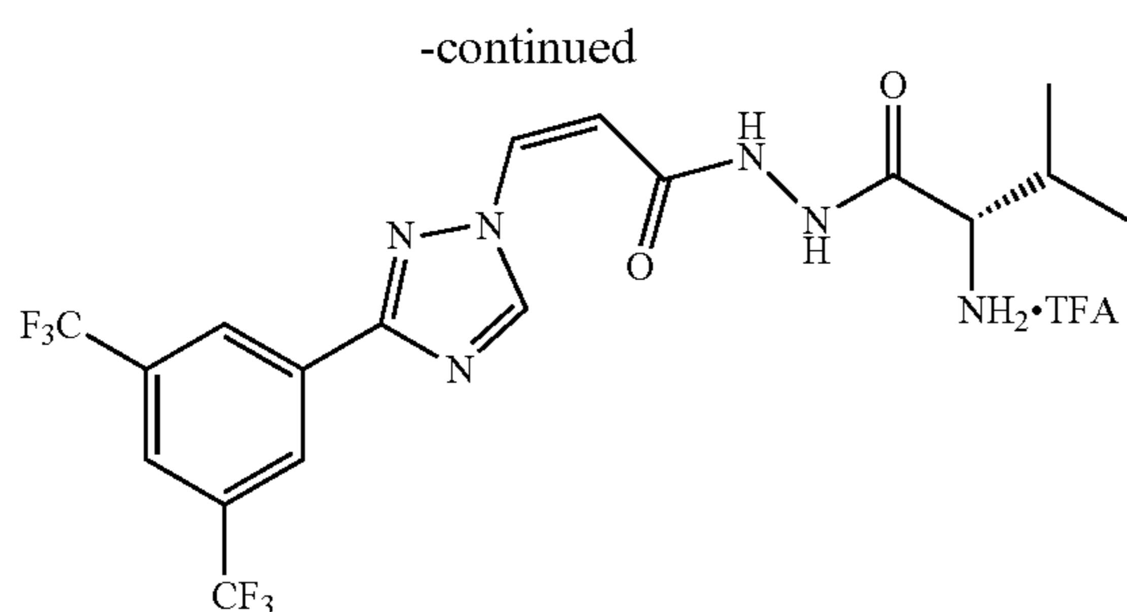
(Z)-3-(3-(3,5-bis(trifluoromethyl)phenyl)-1H-1,2,4-triazol-1-yl)acrylohydrazide (Step 1)
