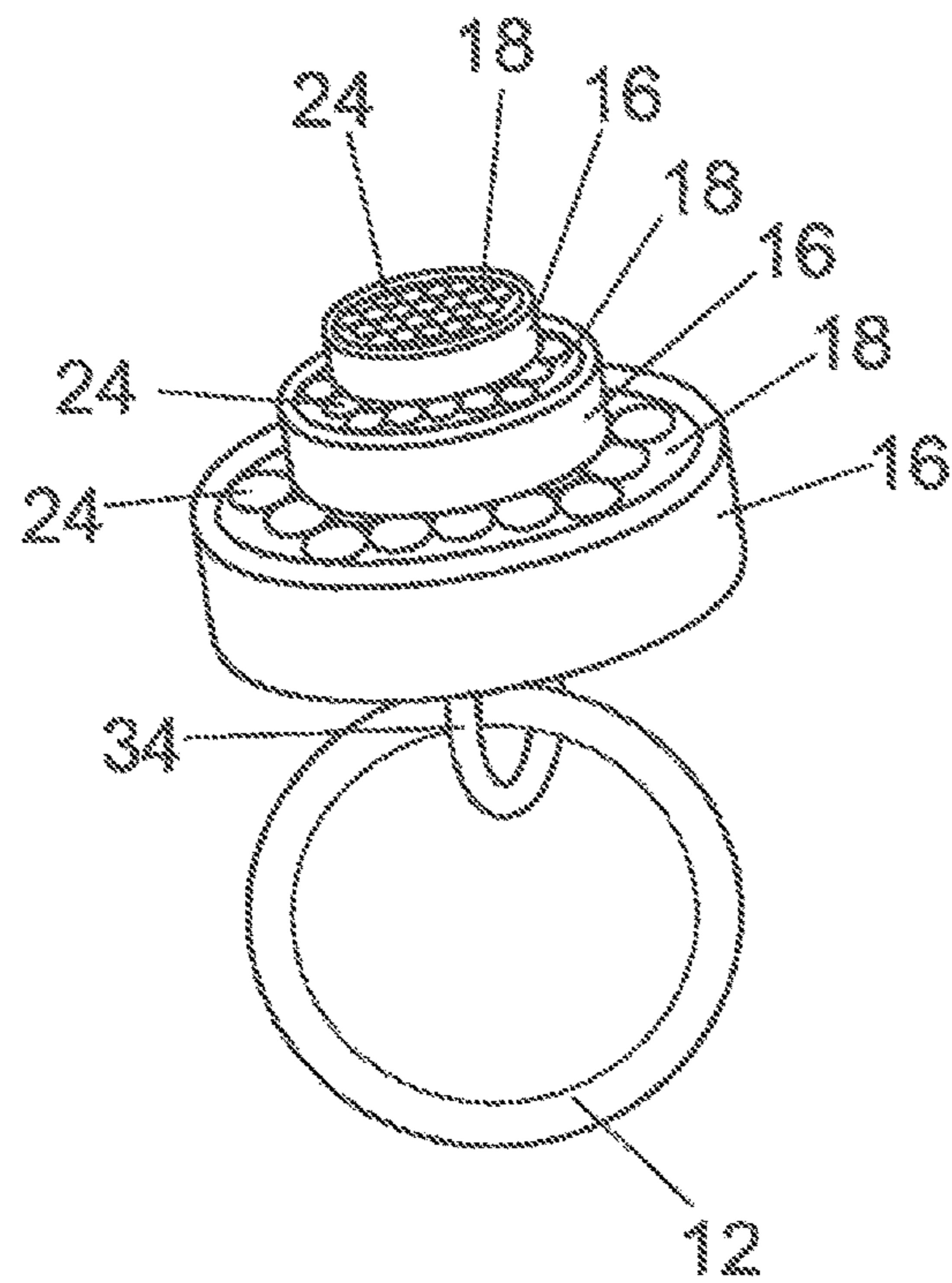
FIG. 12
