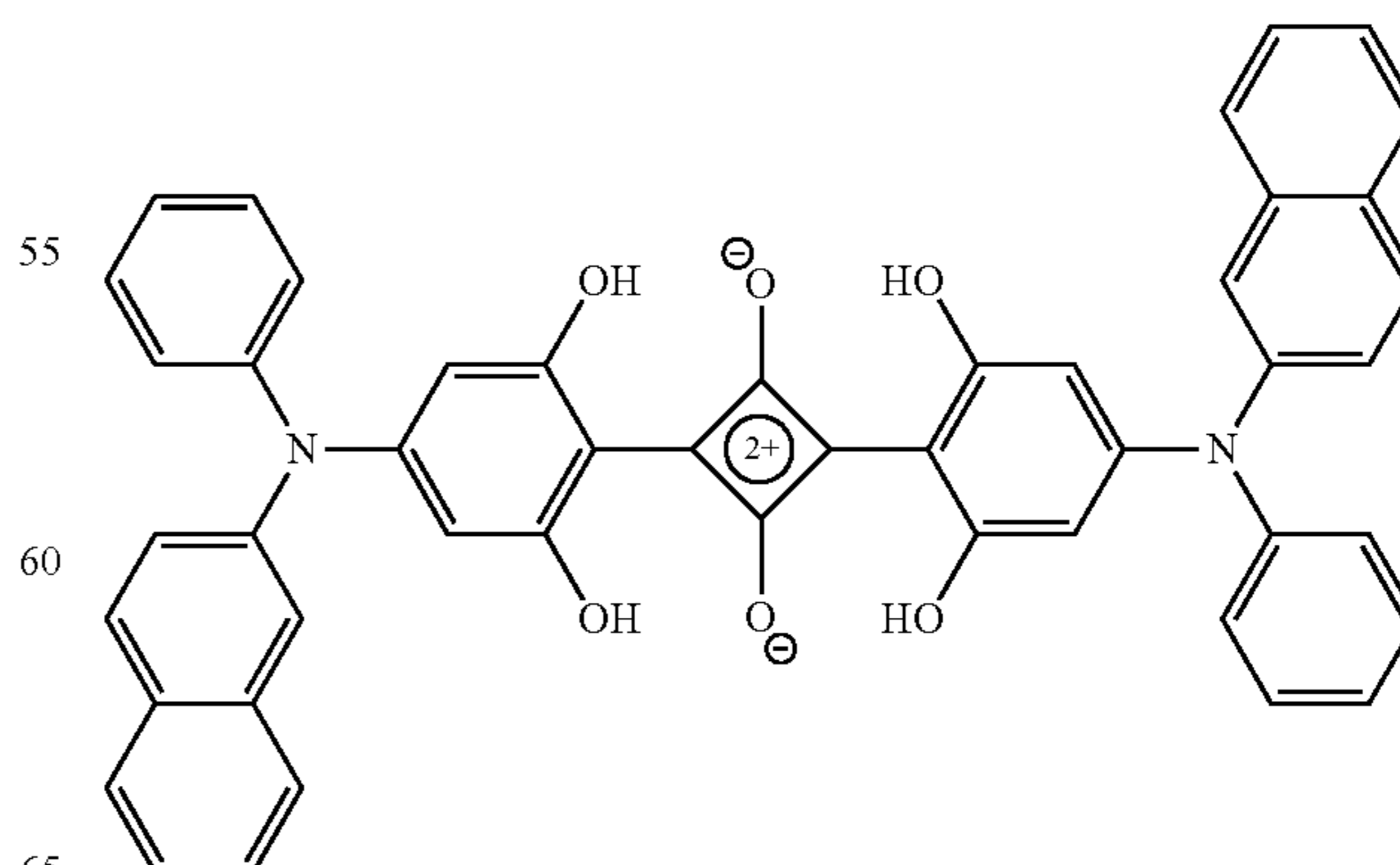
2NPSQ
