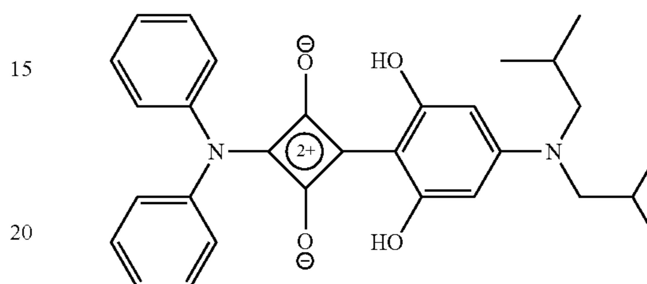
USSQ
