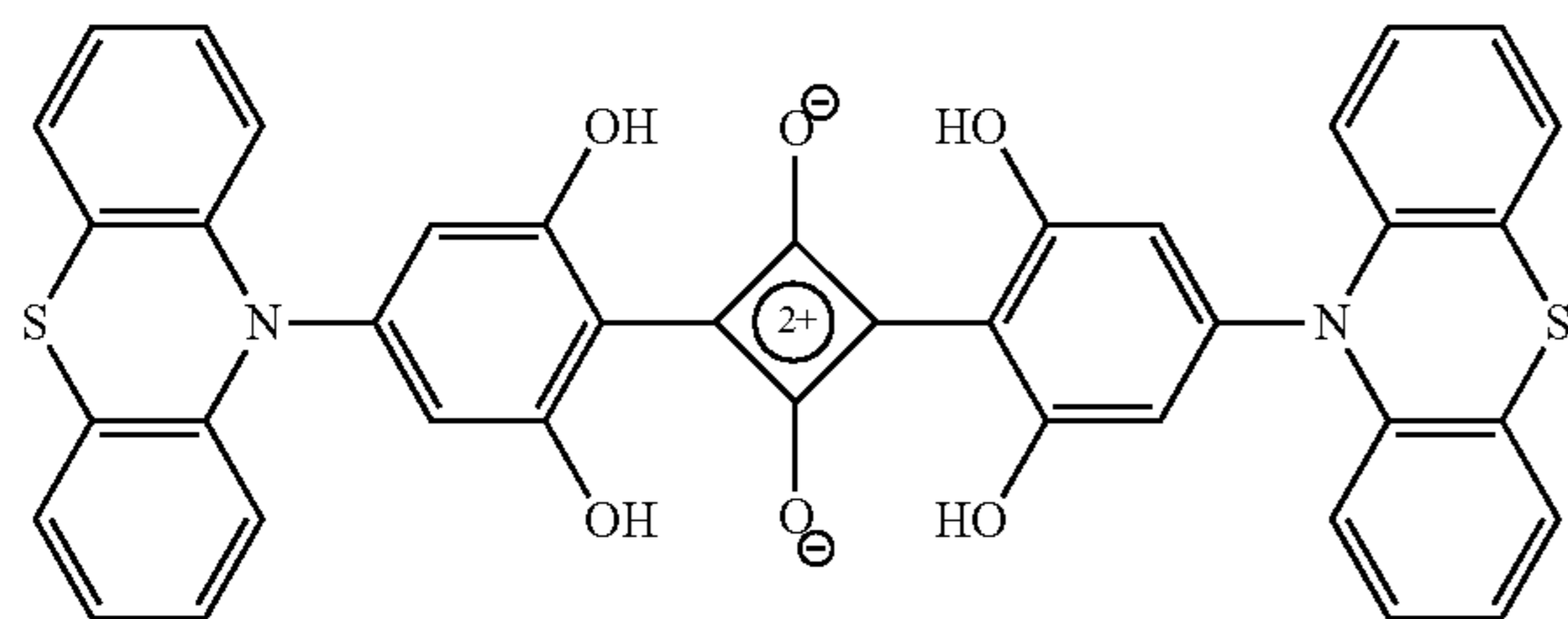
PTSQ
