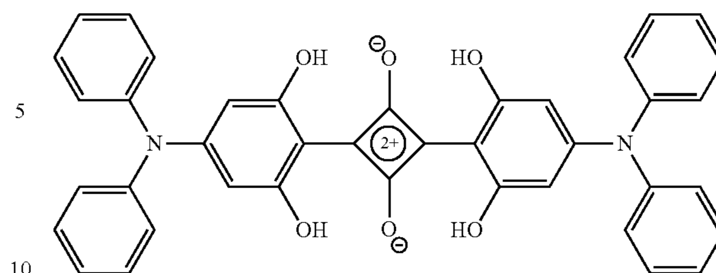
DPSQ
