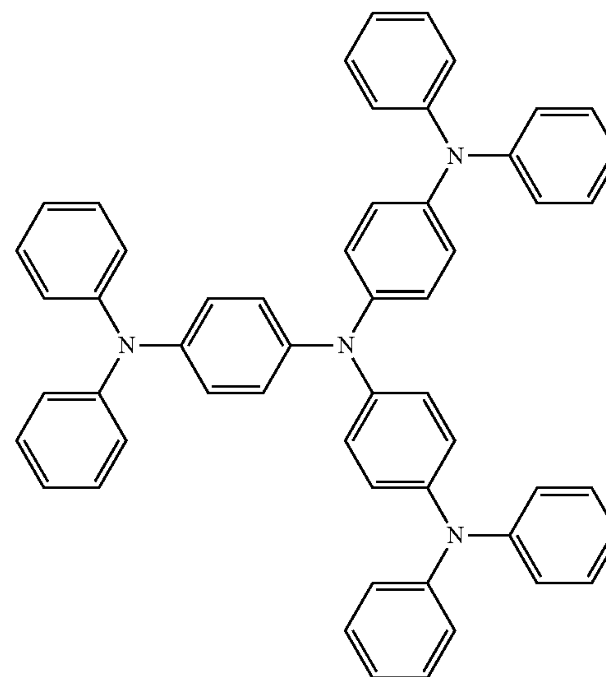
m-MTDATA
