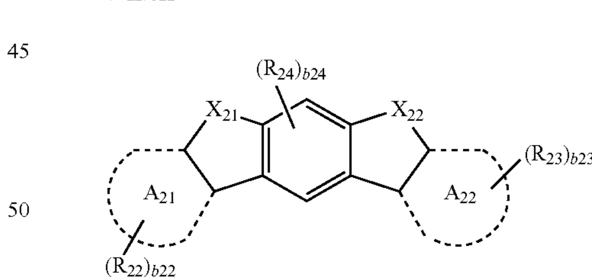
Formula 10E
