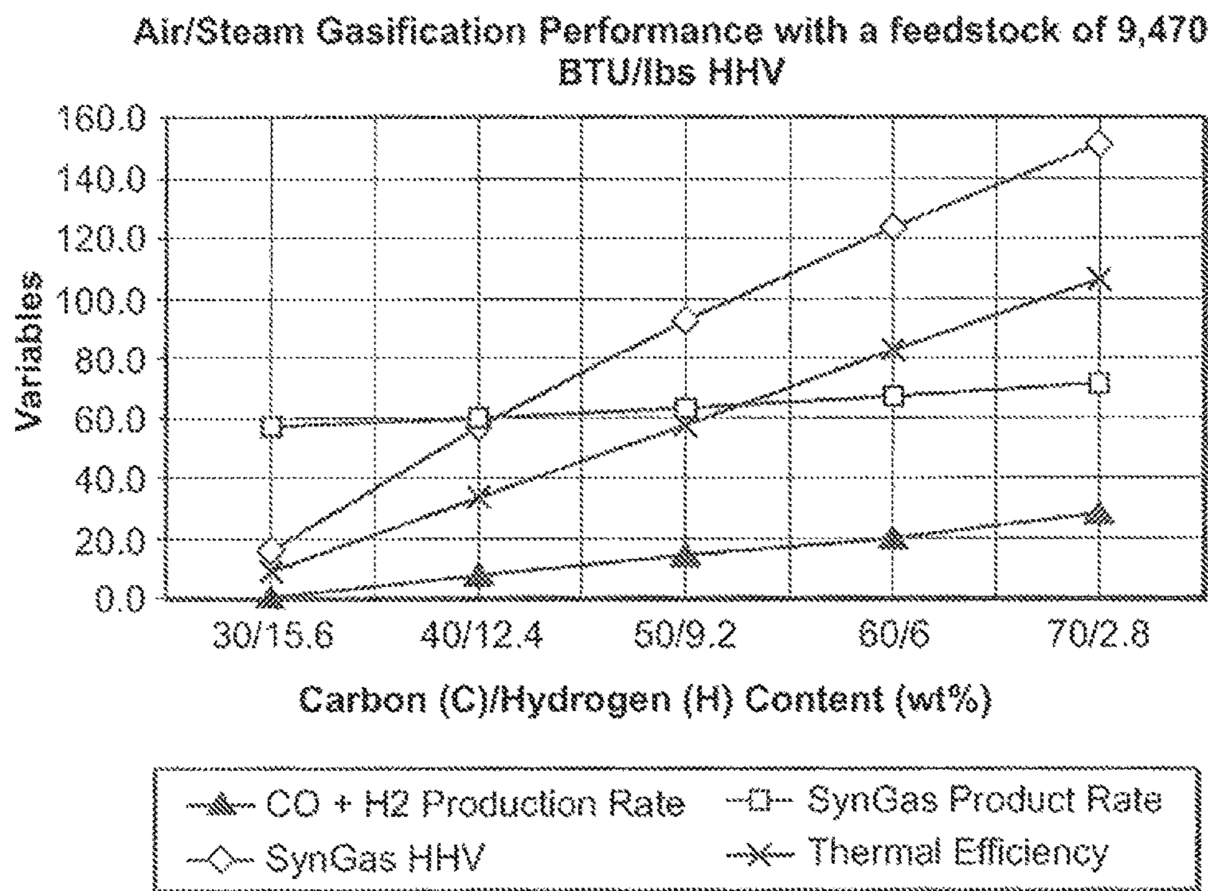
FIG. 15
