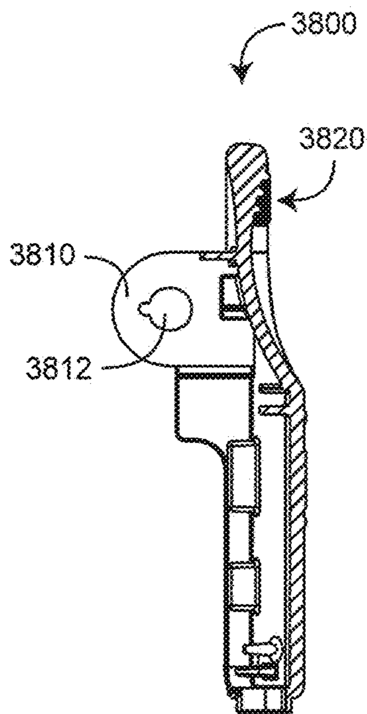
SECTION A-A FIG. 38D
