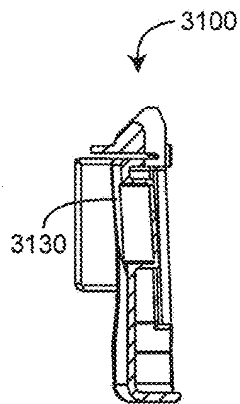
SECTION A-A FIG. 31F
