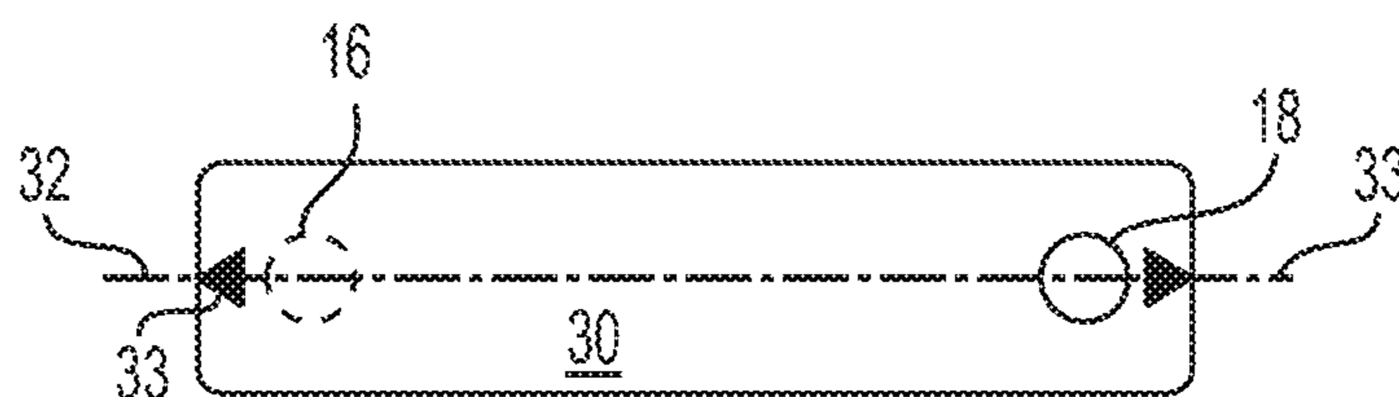
FIG. 4B
