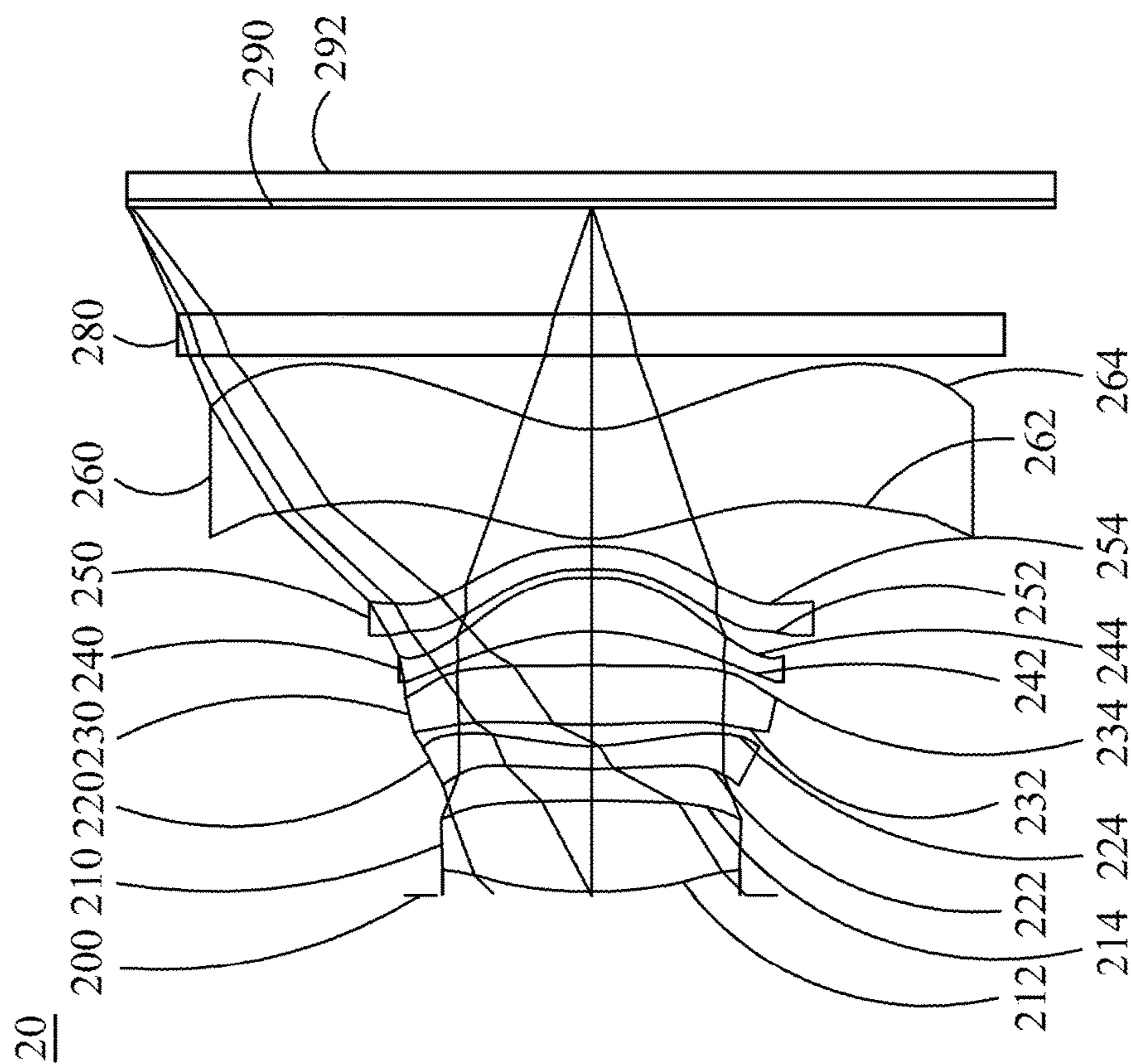
FIG. 2A
