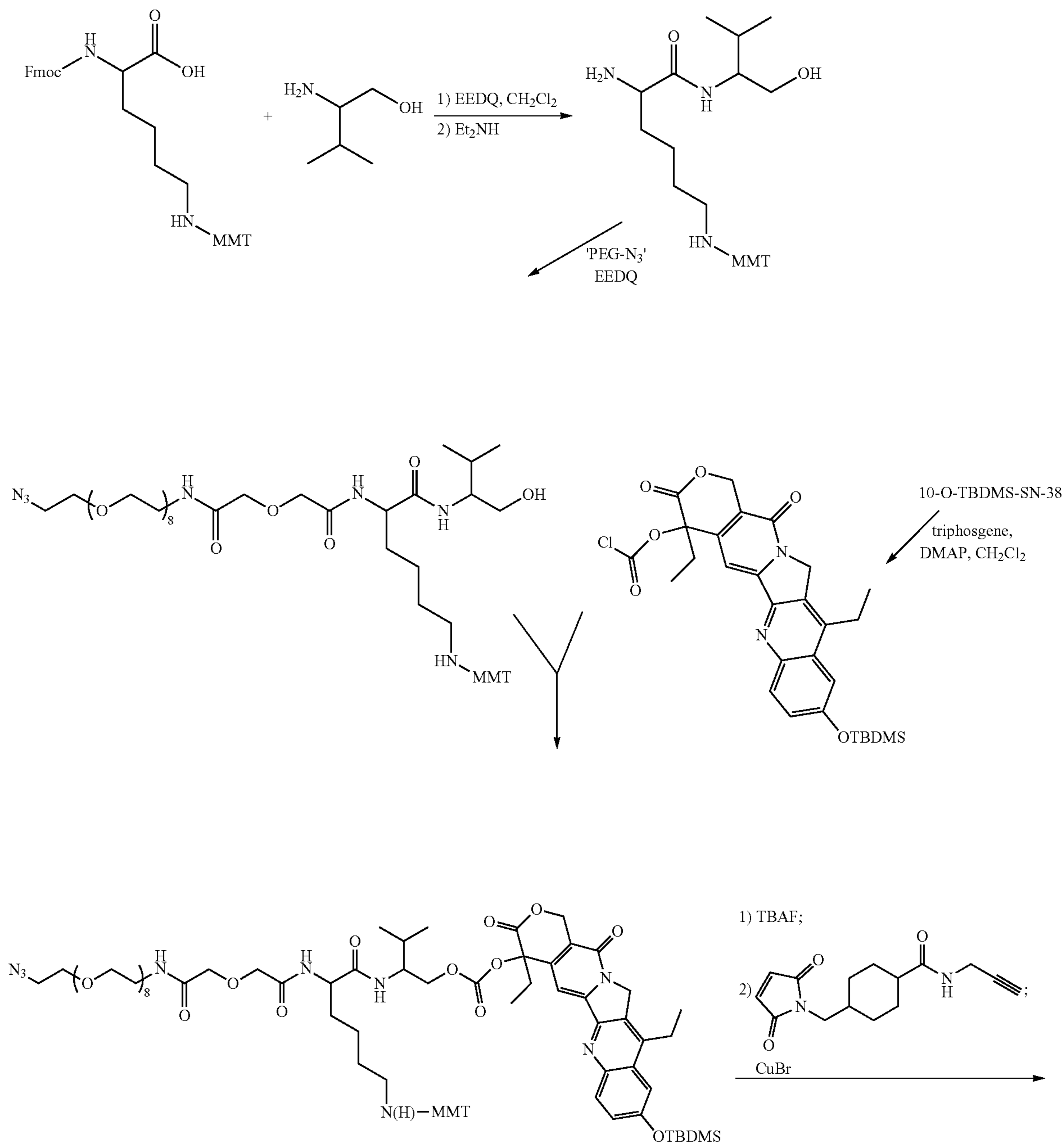
Scheme-2
