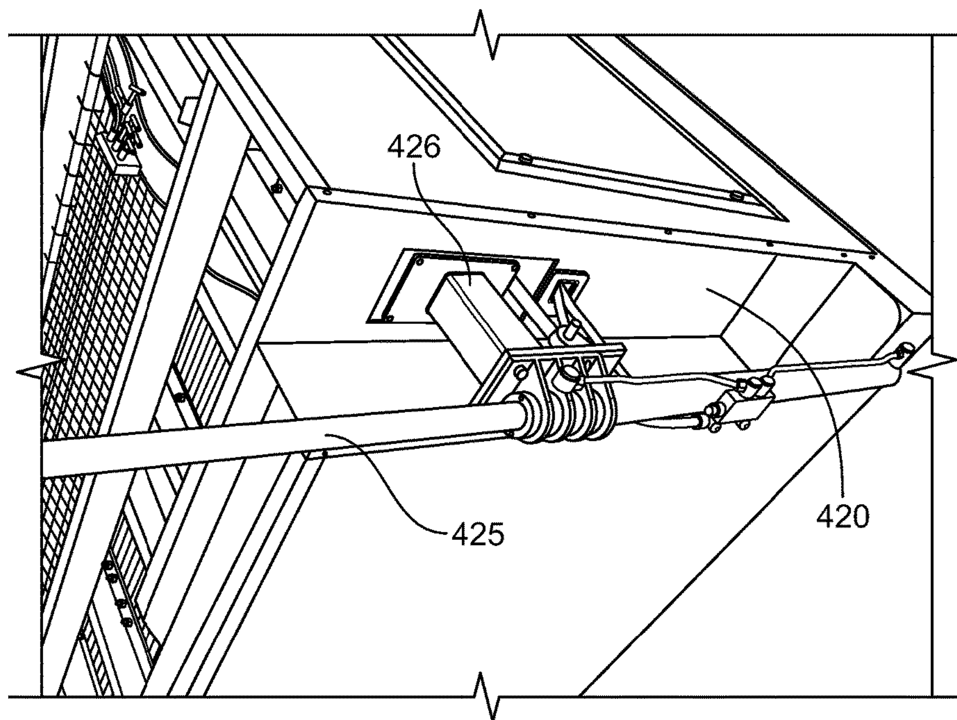
FIG. 4E
