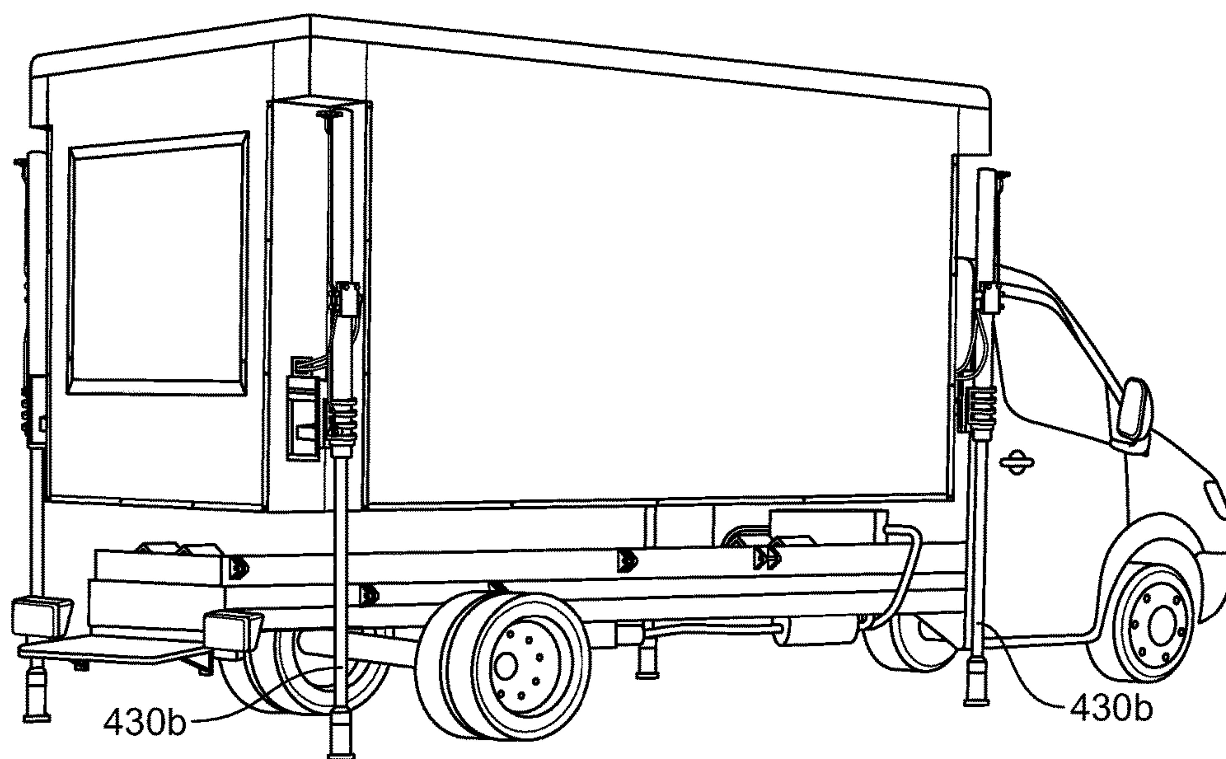
FIG. 4C
