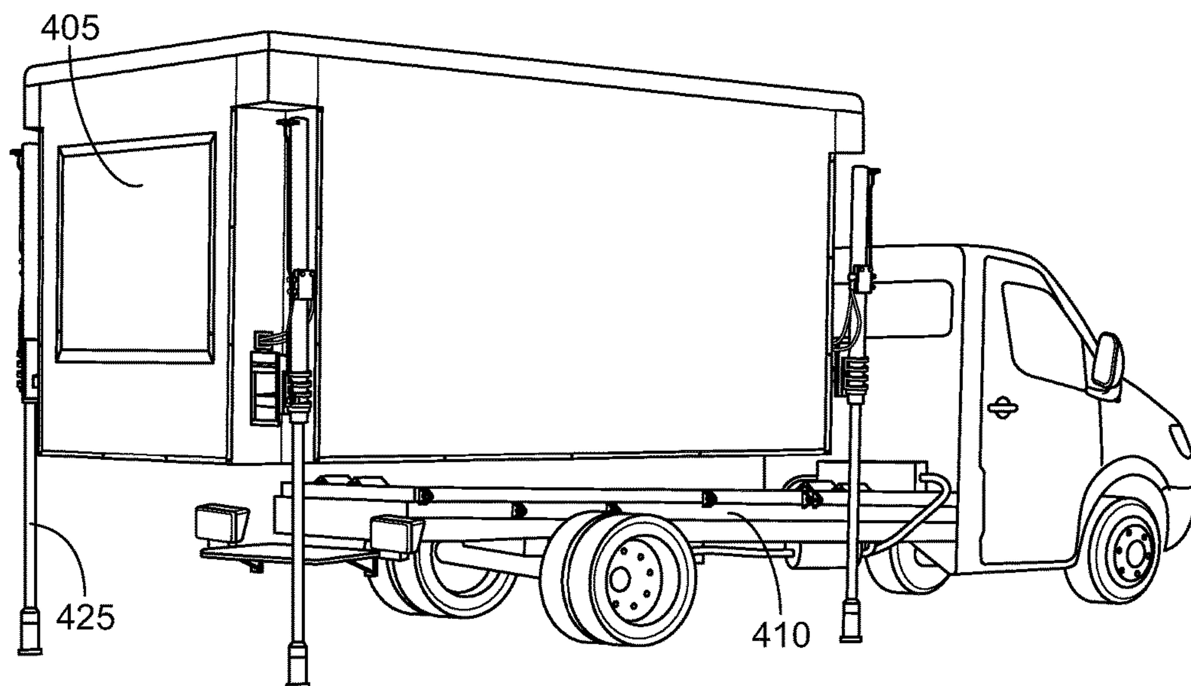
FIG. 4F
