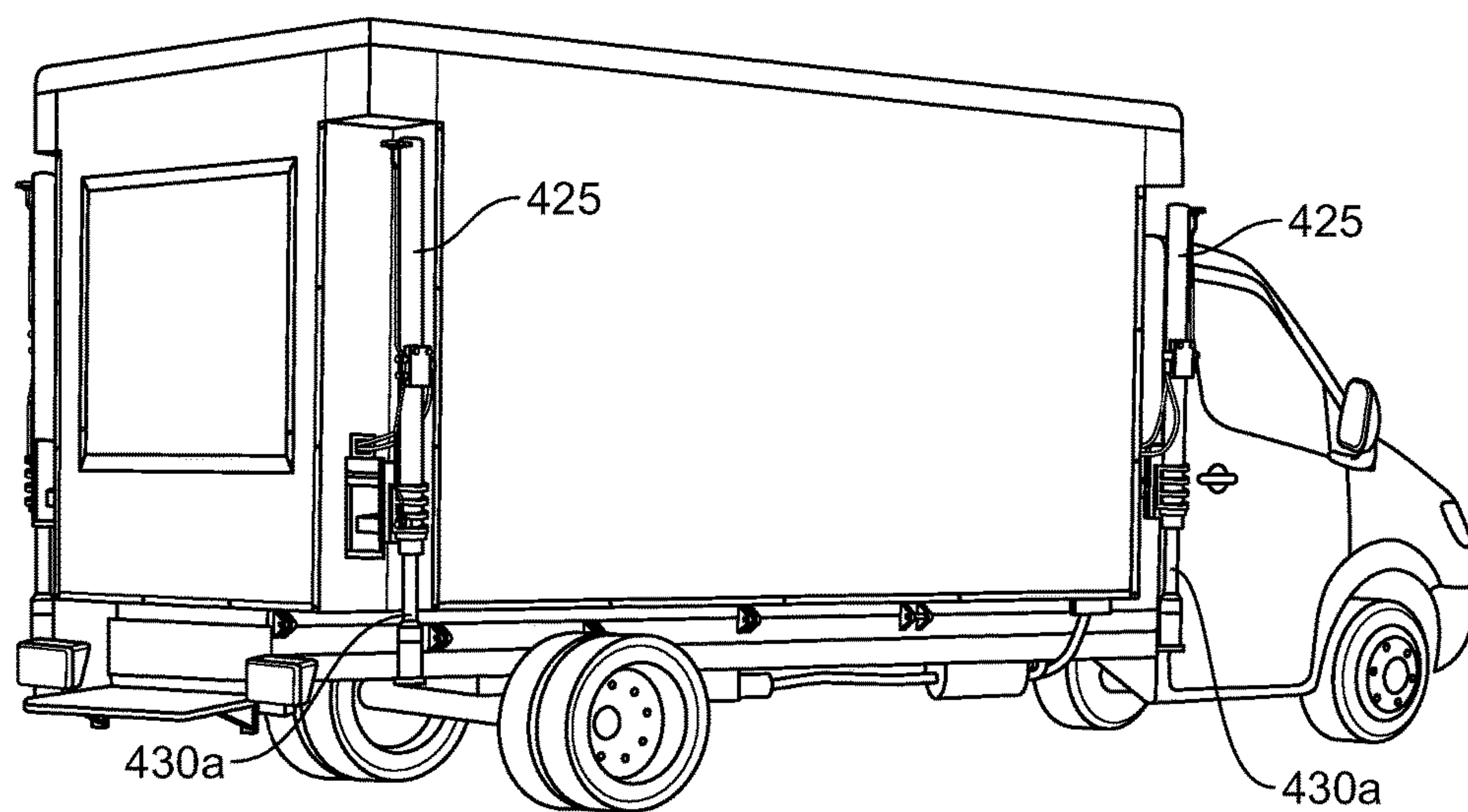
FIG. 4C
