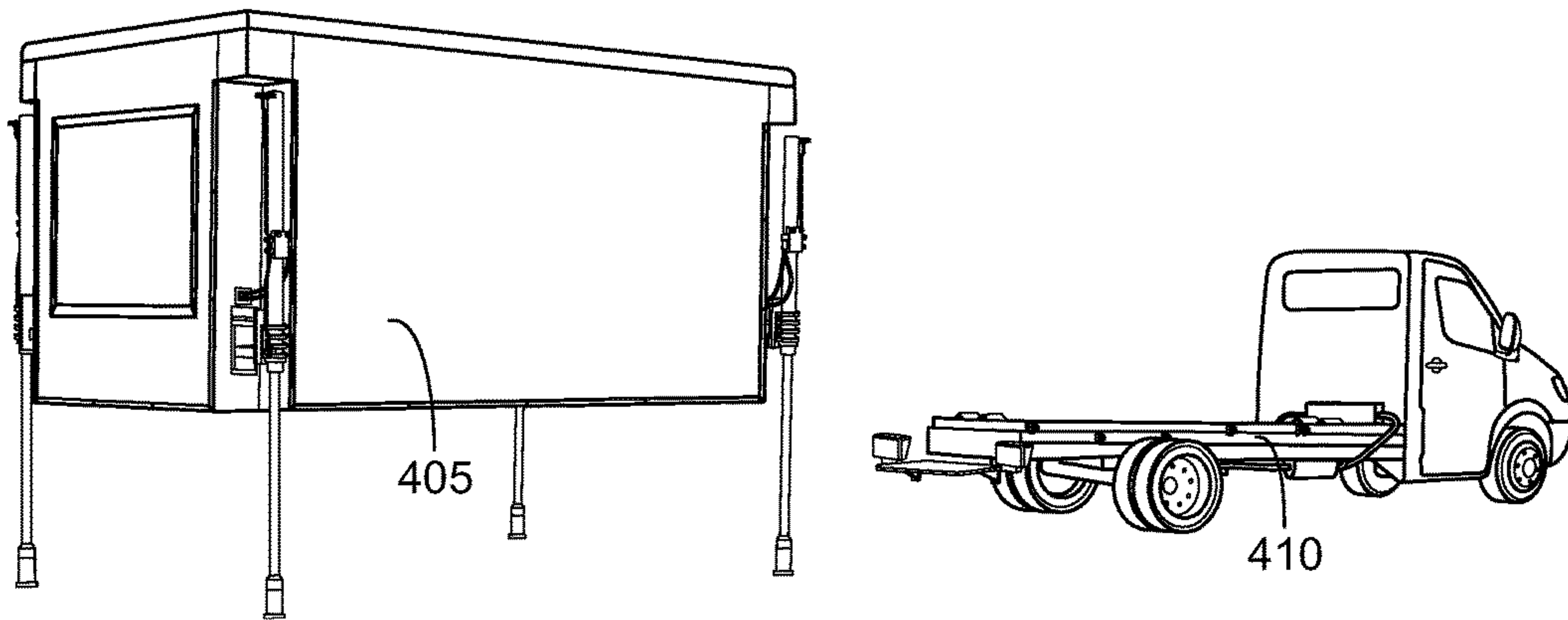
FIG. 4G
