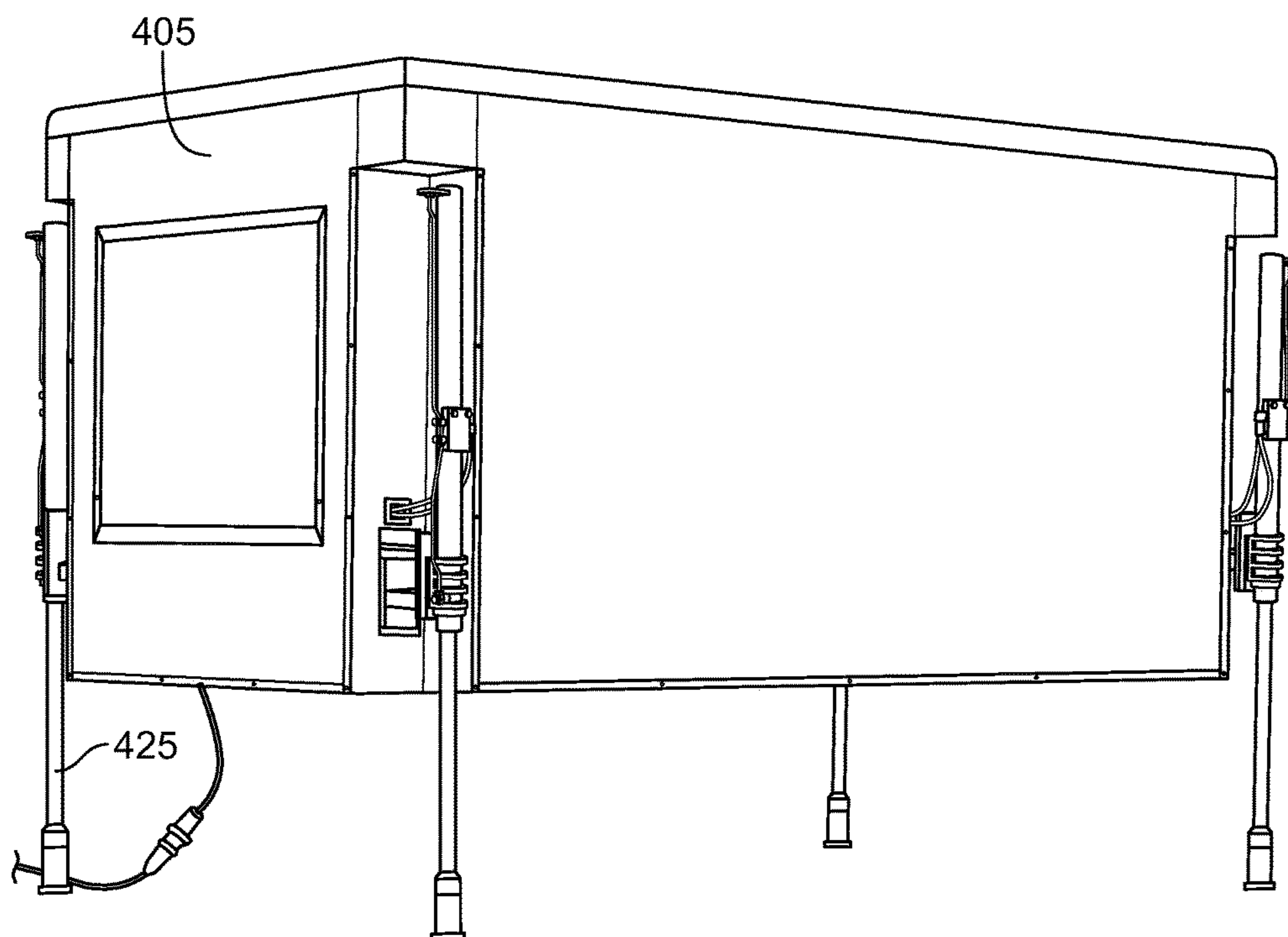
FIG. 4I
