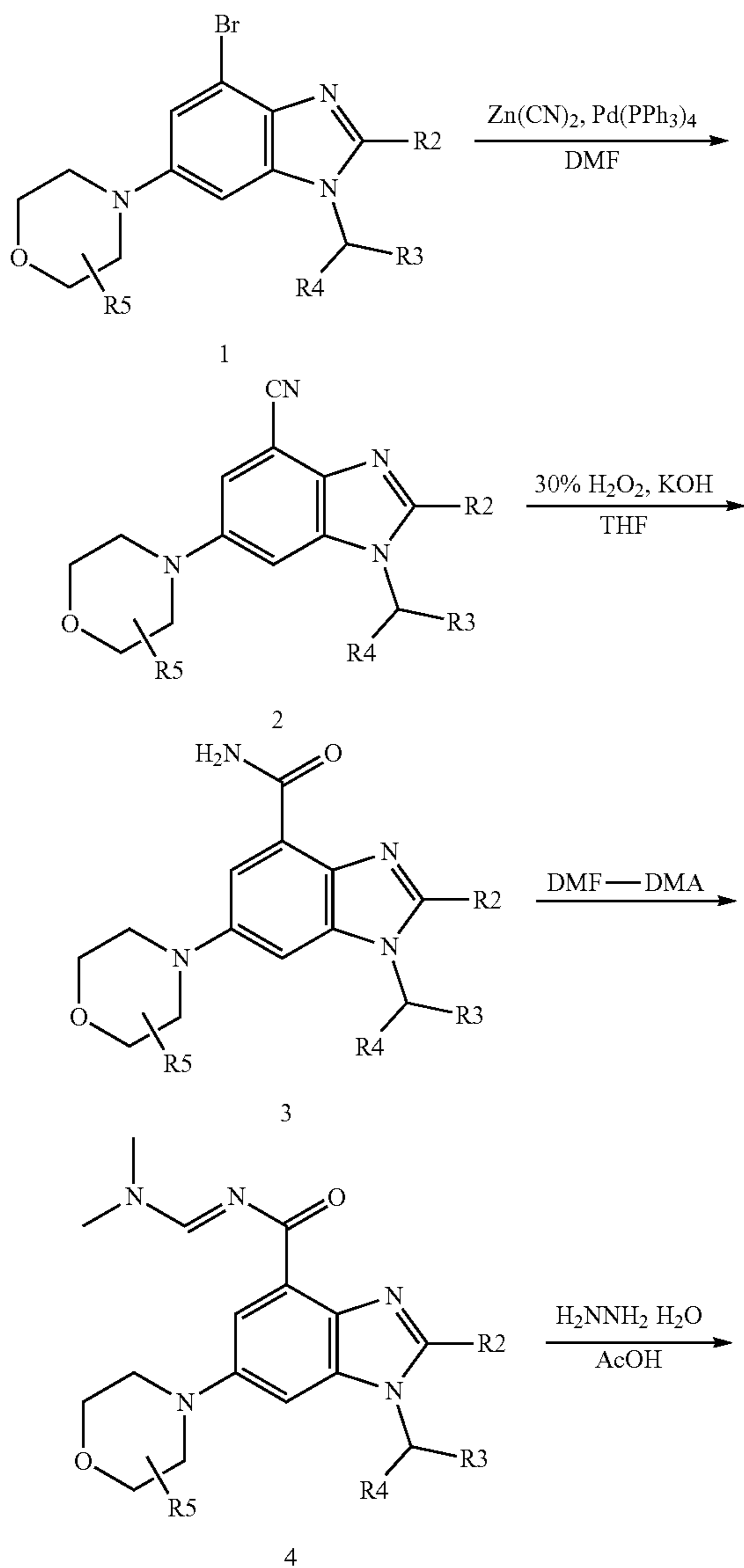
Scheme VI
