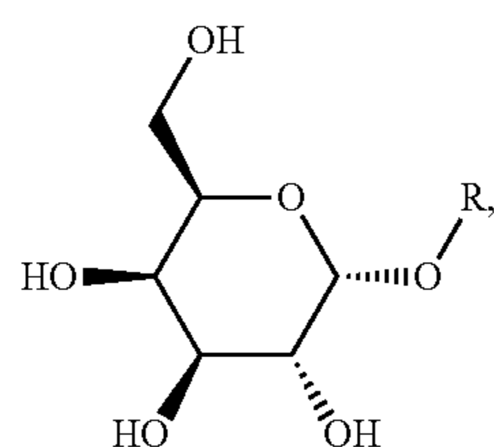
\alpha -GalCer
