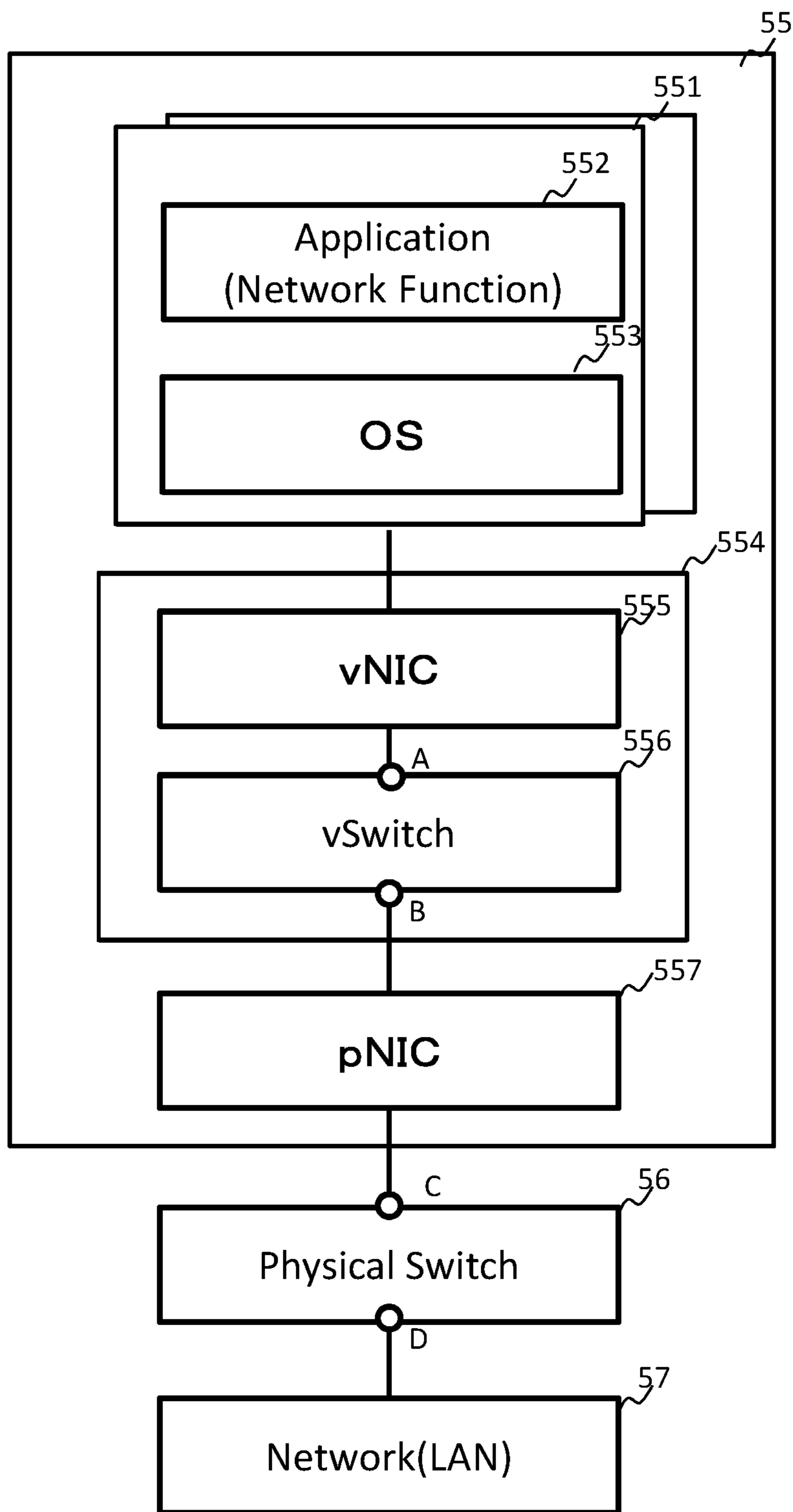
FIG. 9
