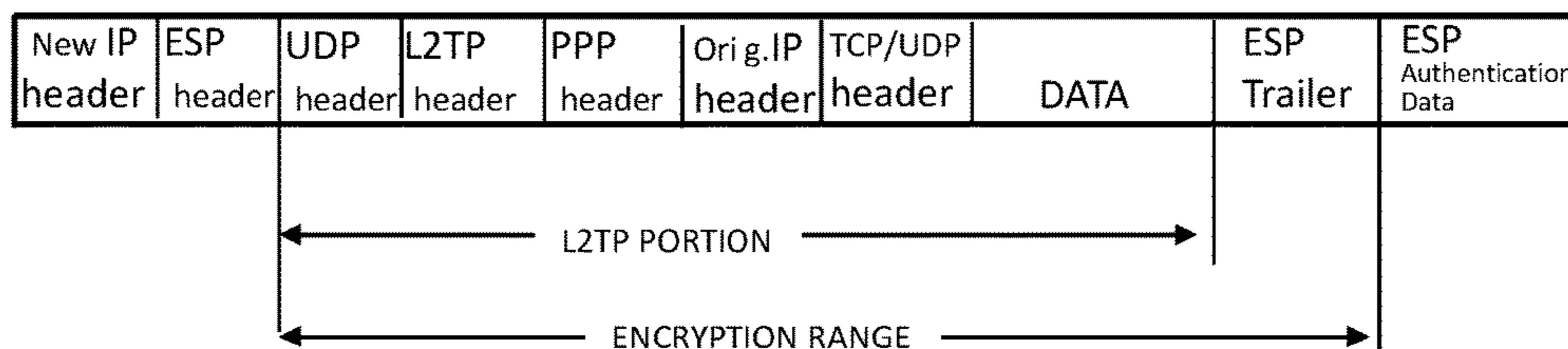
FIG. 10E
