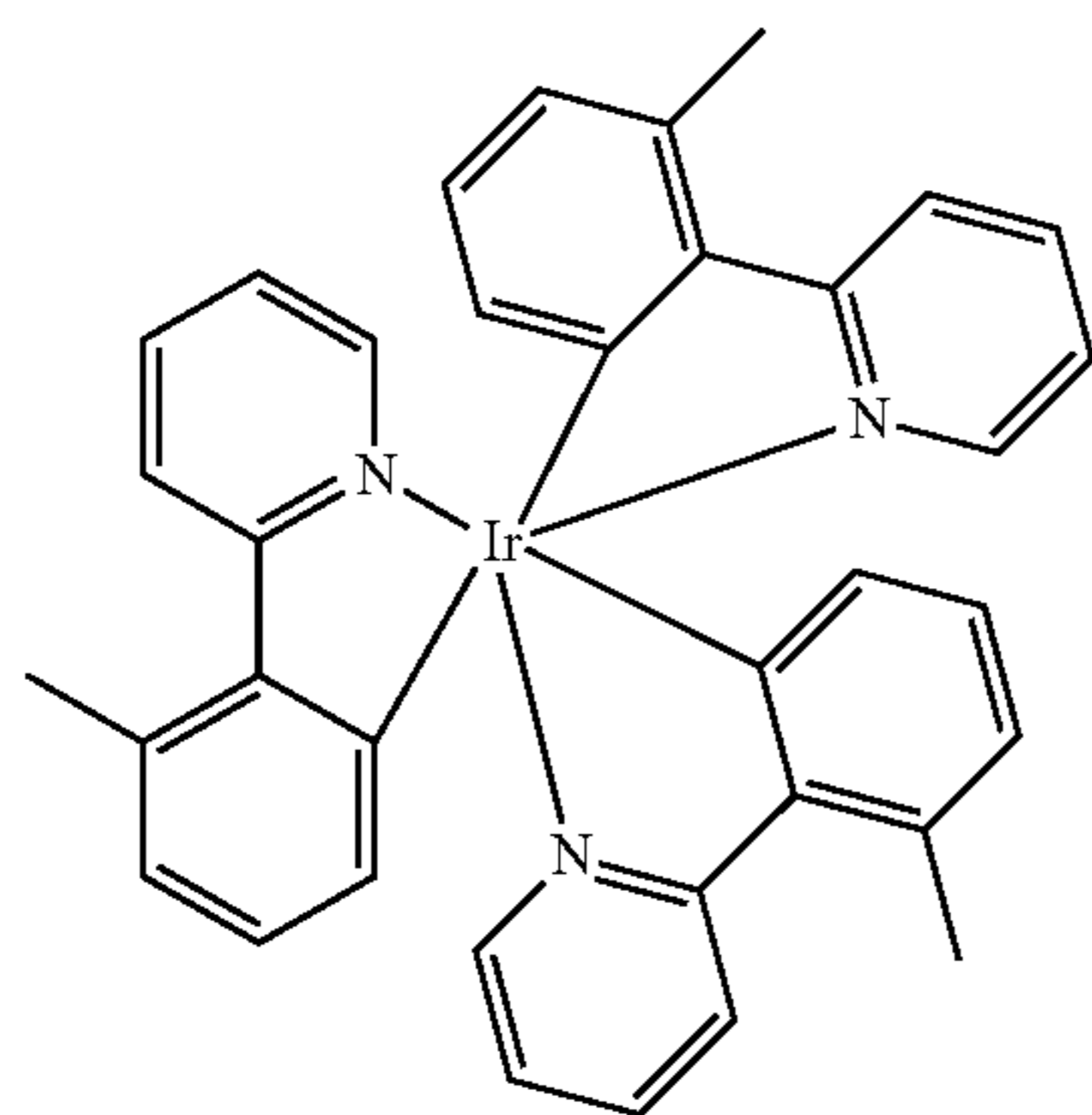
Dopant 1
