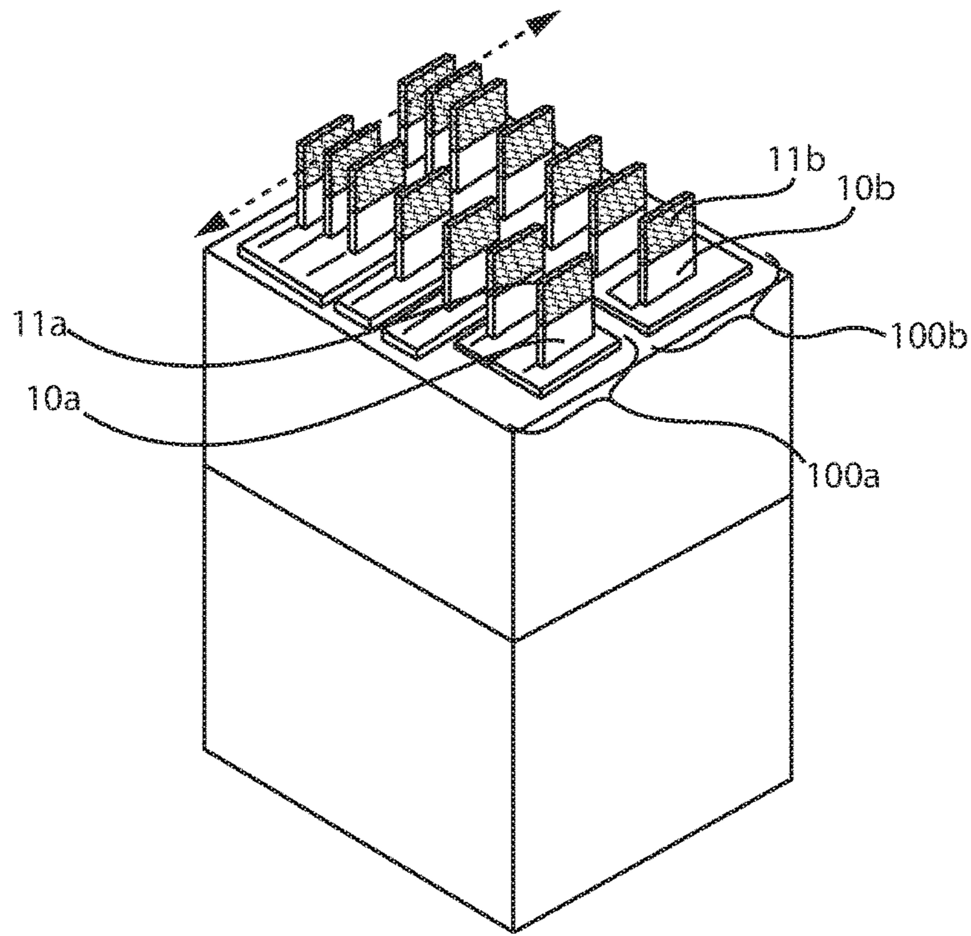
FIG. 2A
