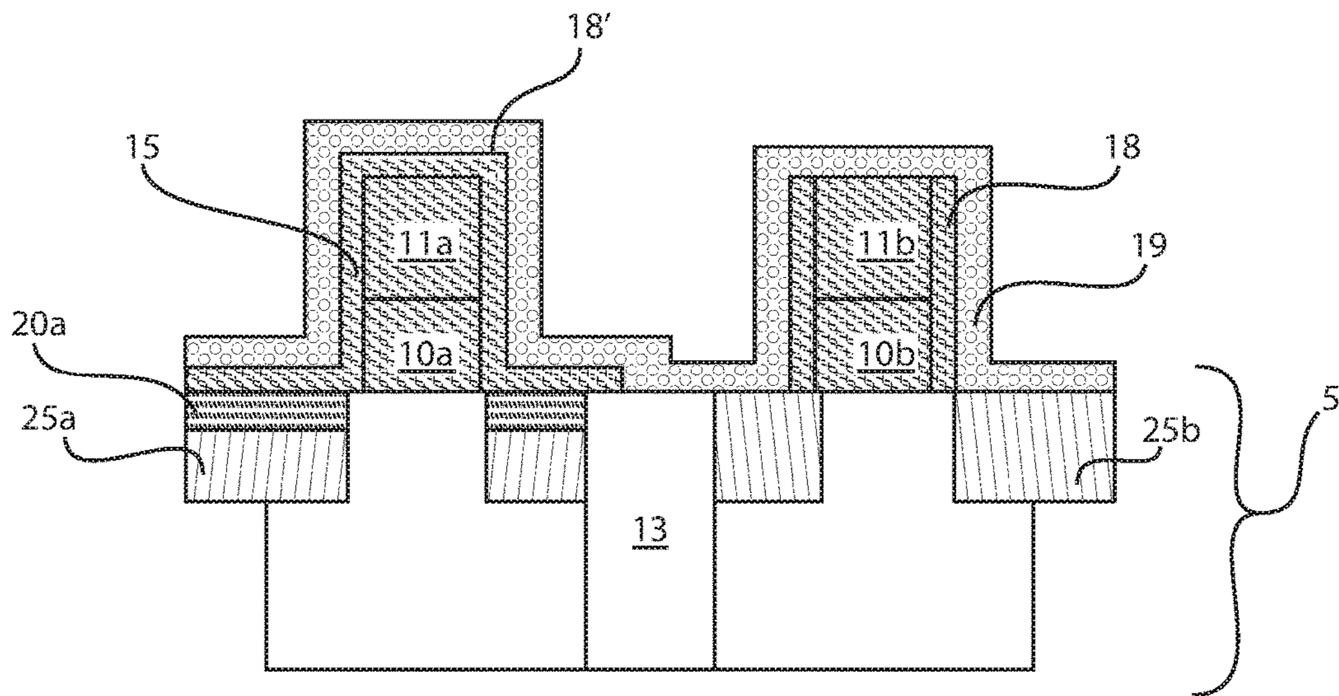
FIG. 7
