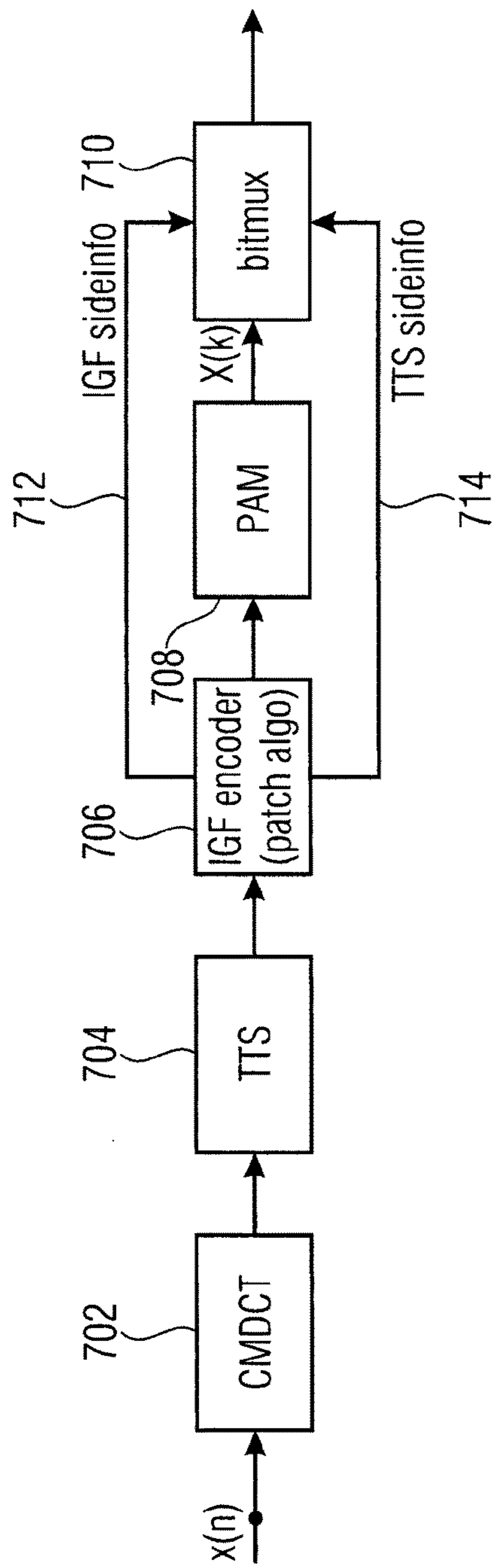
FIG 7A (ENCODER)
