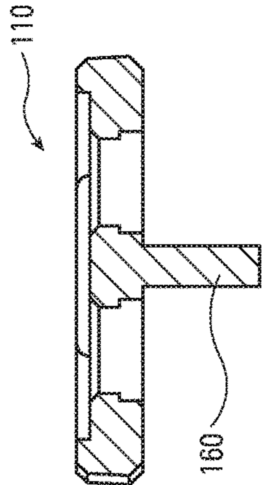
Fig. 1I
