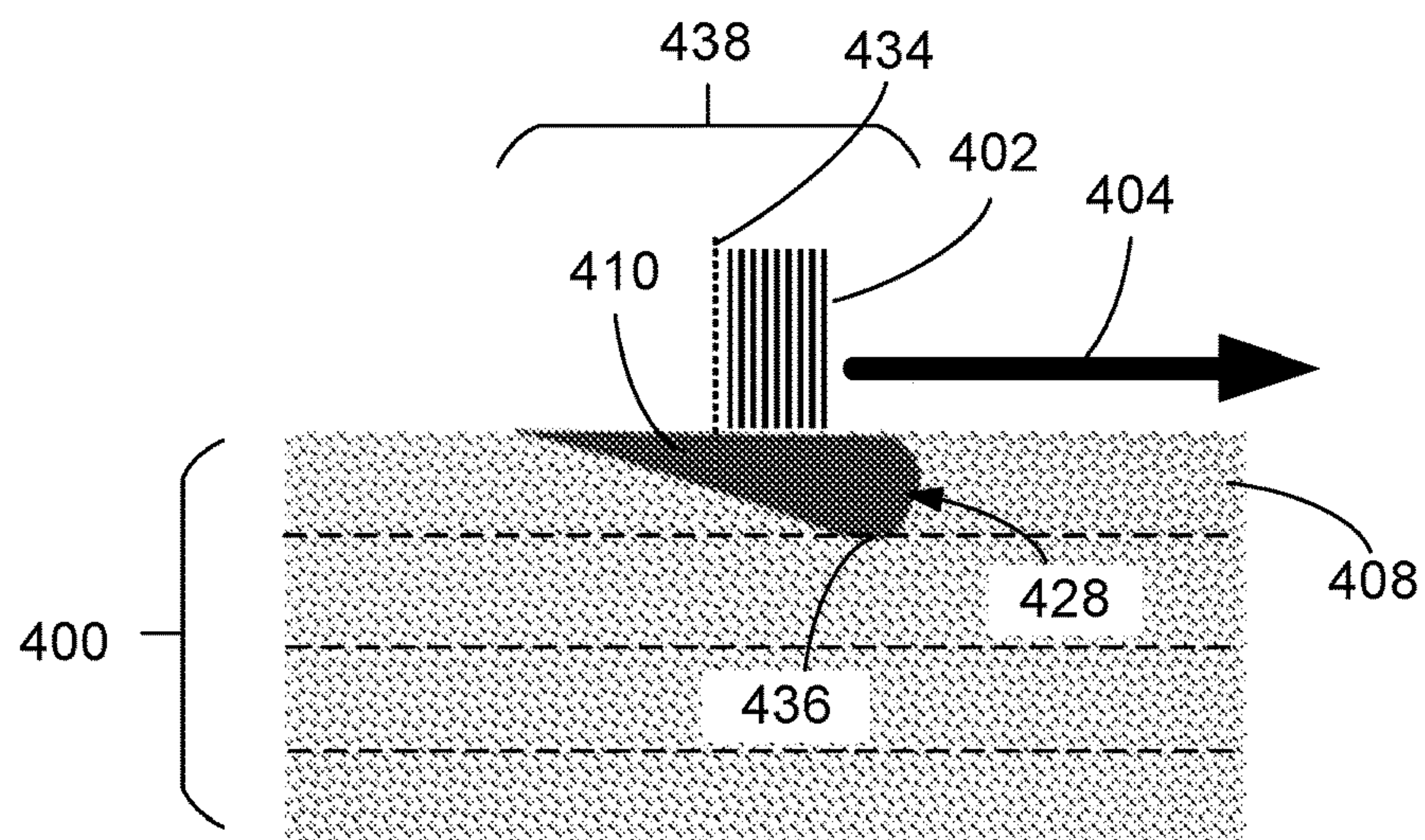
FIG. 4A
