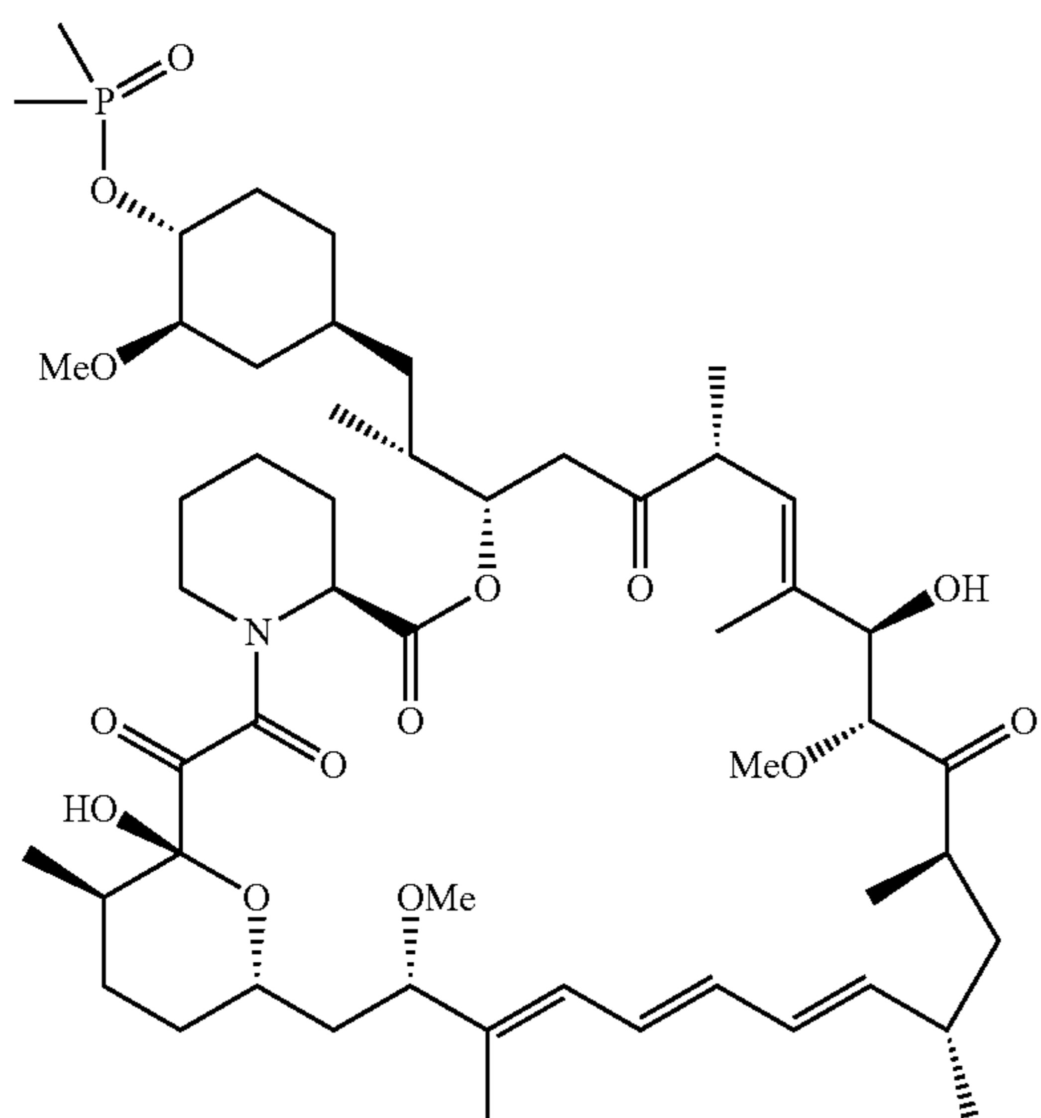
Ridaforolimus (MK-8669)
