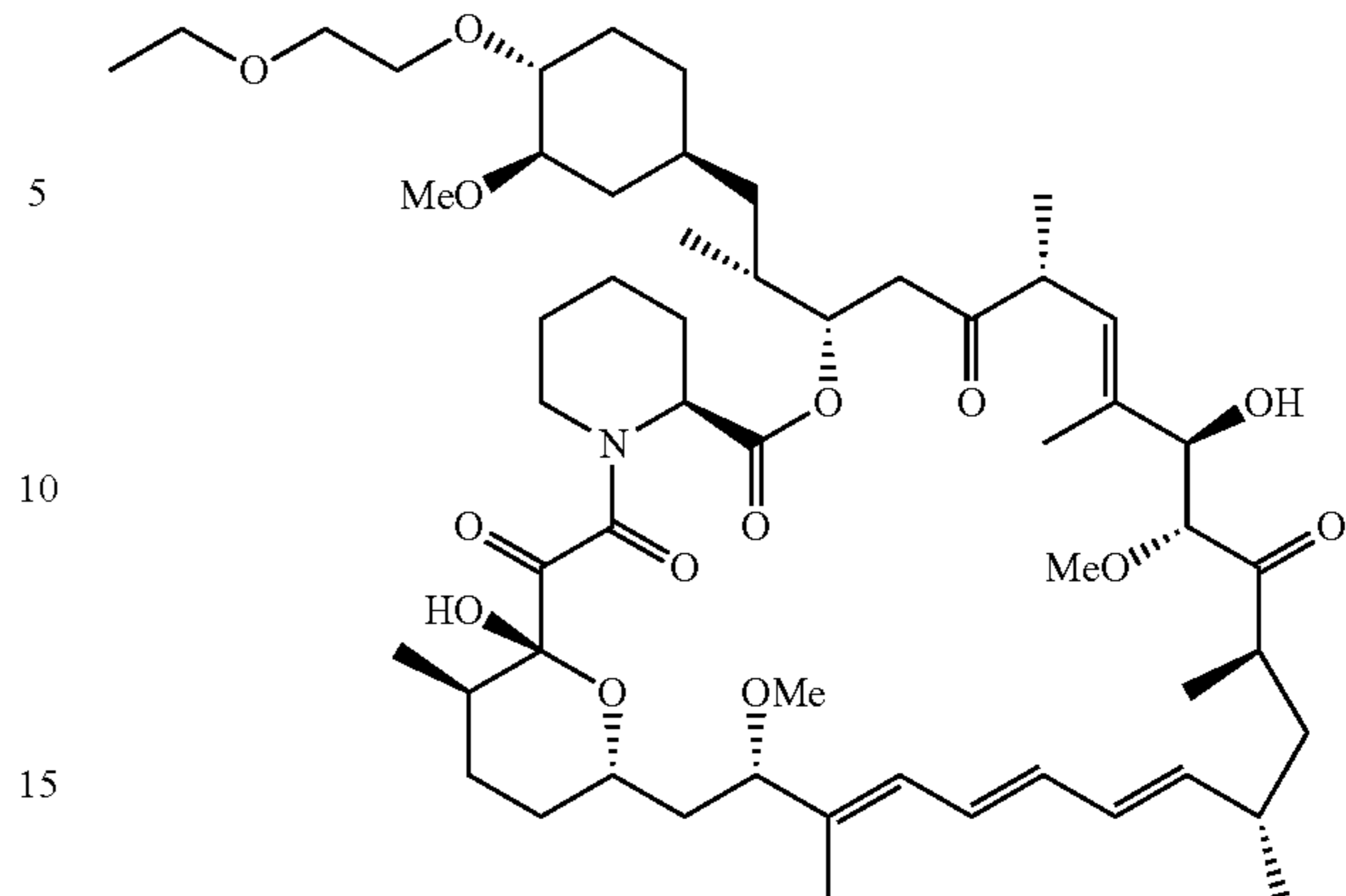
Umirolimus
