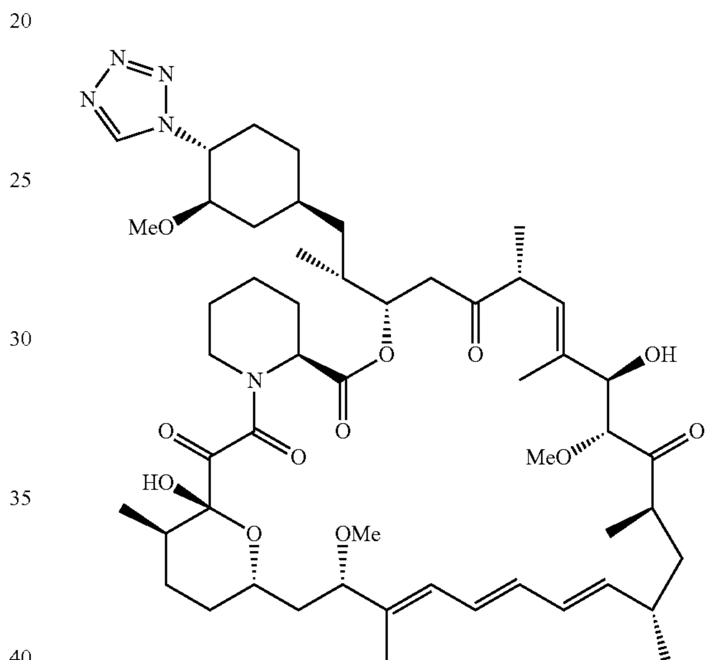
Zotarolimus (ABT-578)
