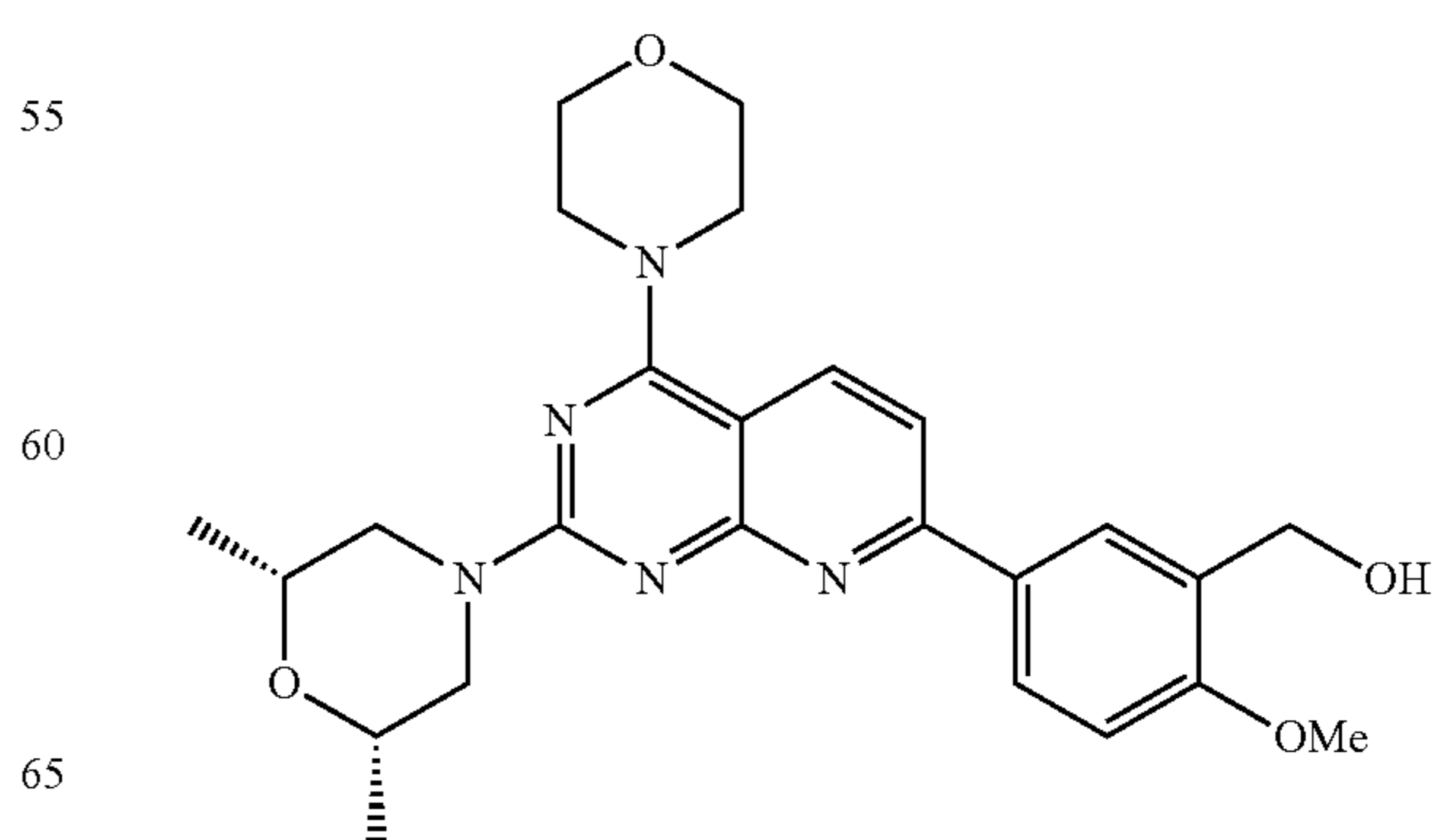
KU-0063794
