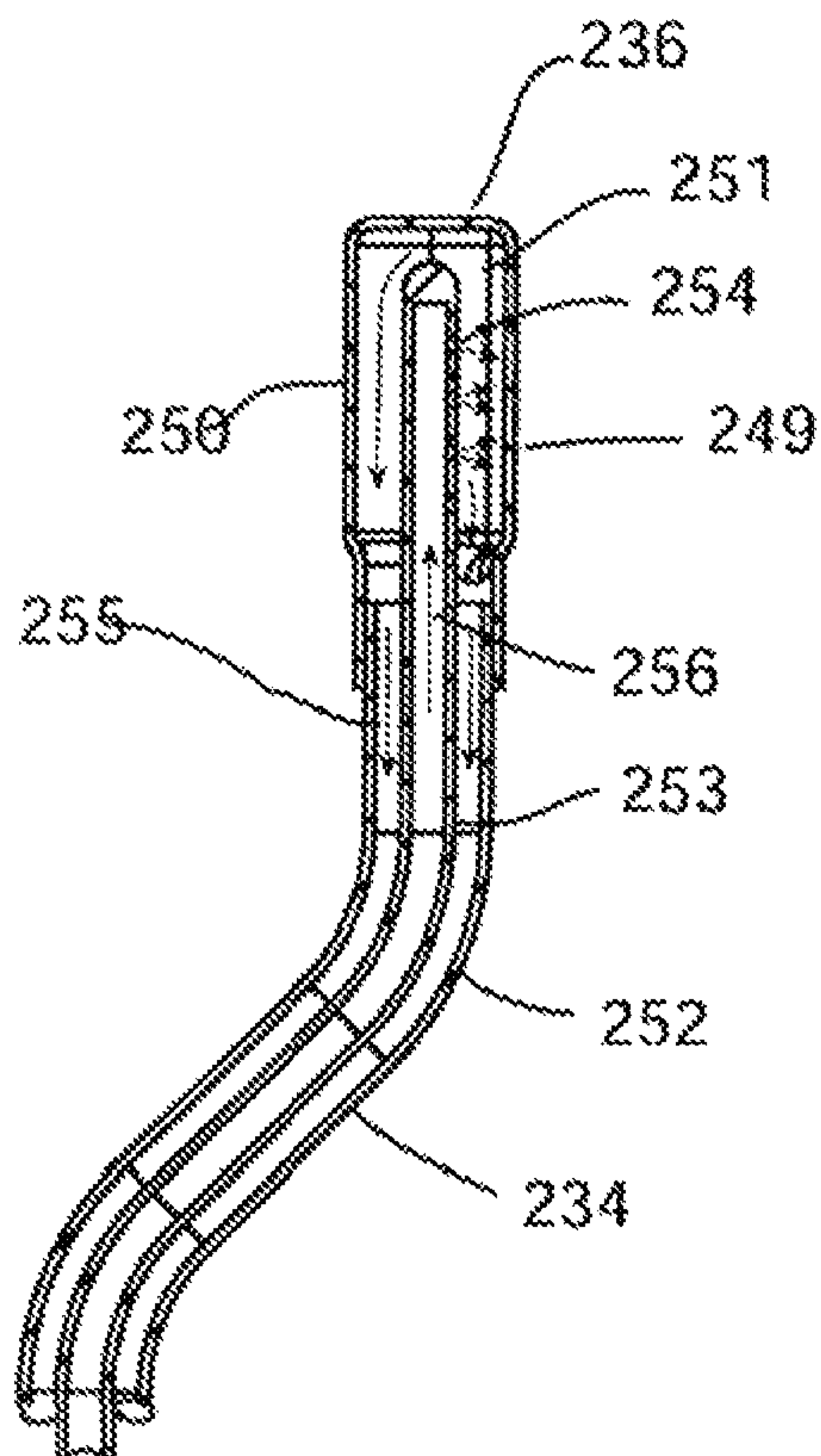
Section A-A
