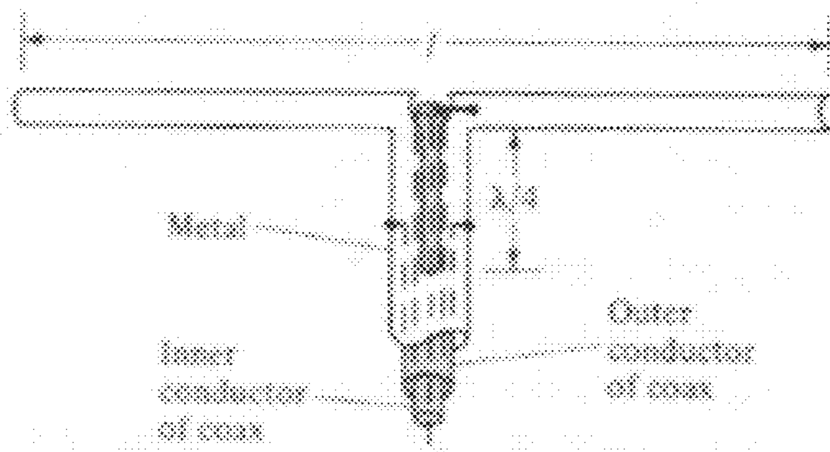
(d) Coaxial balun (1 : 1)
