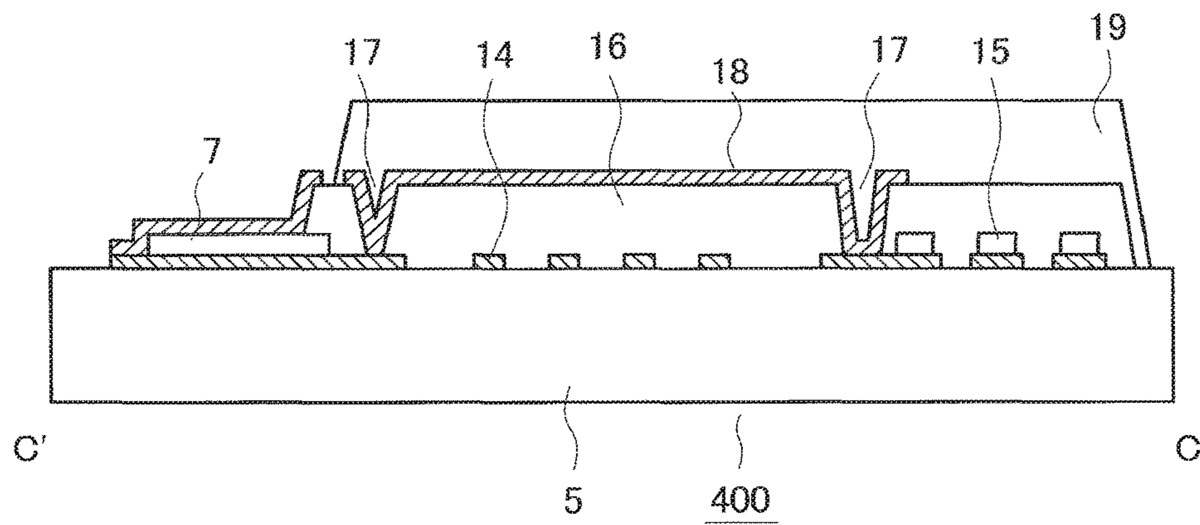
FIG. 9B
