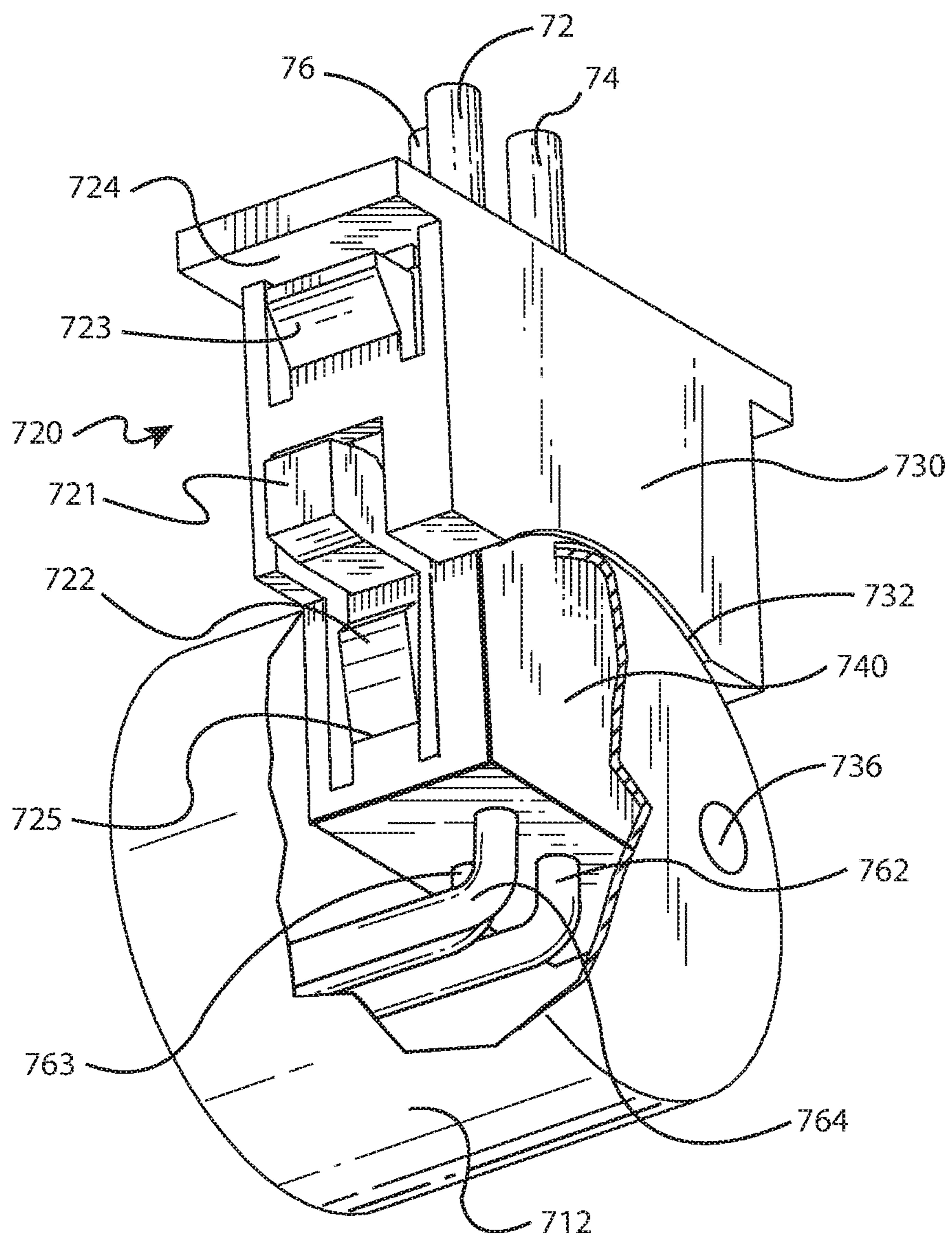
FIG. 18
