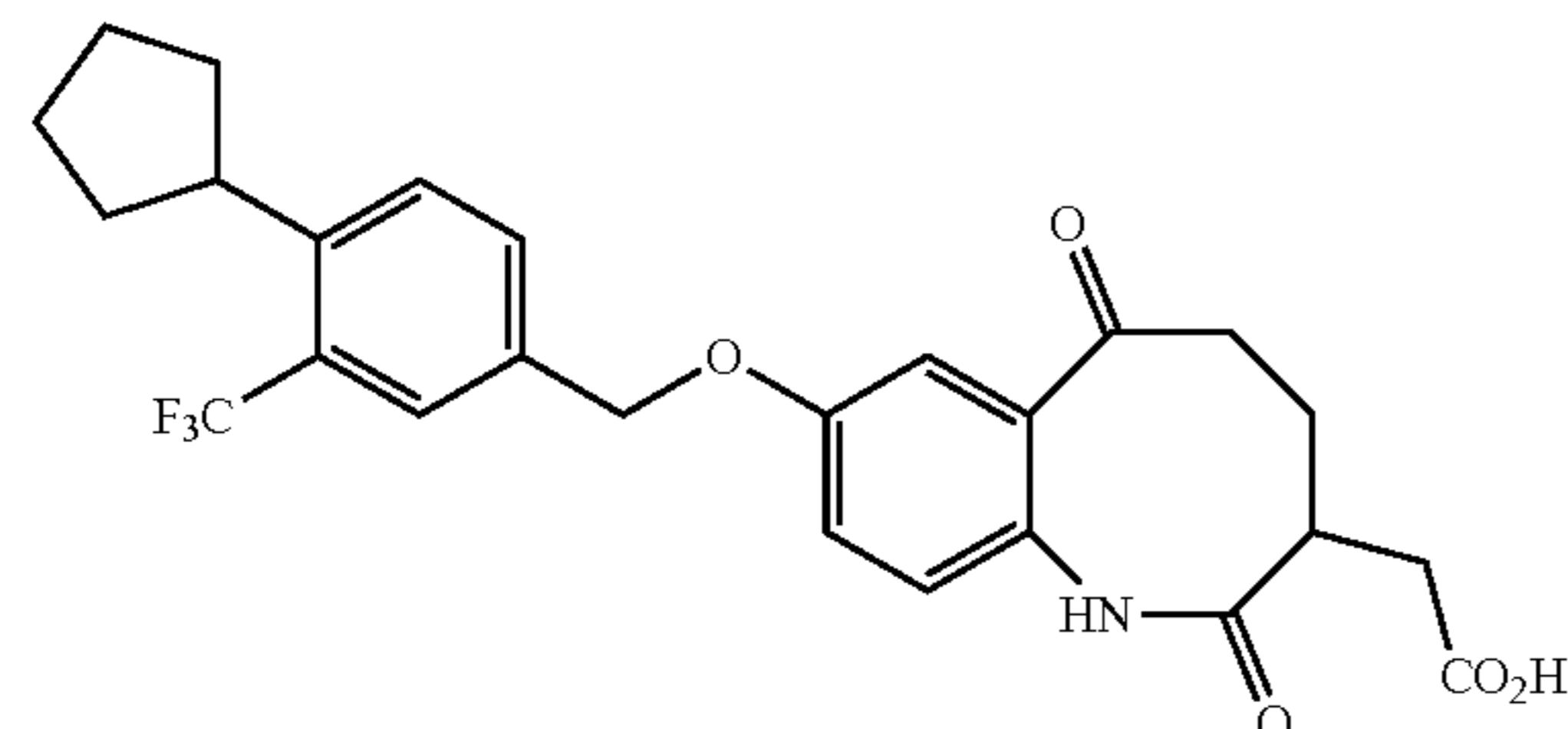
Cmpd A
