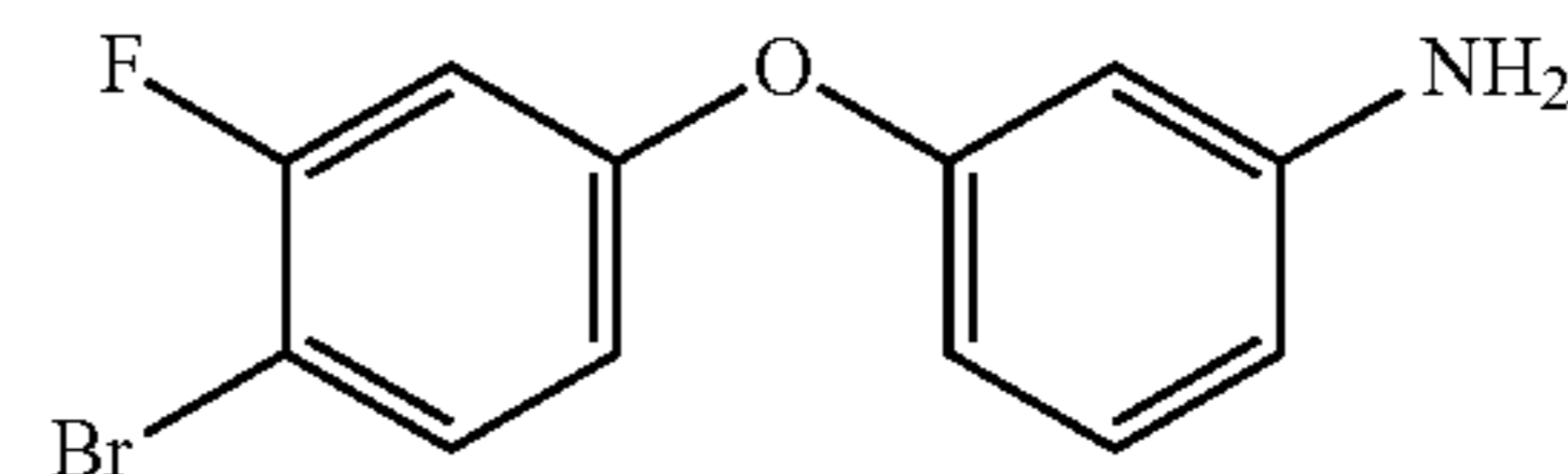
3-(4-bromo-3-fluorophenoxy)benzenamine
