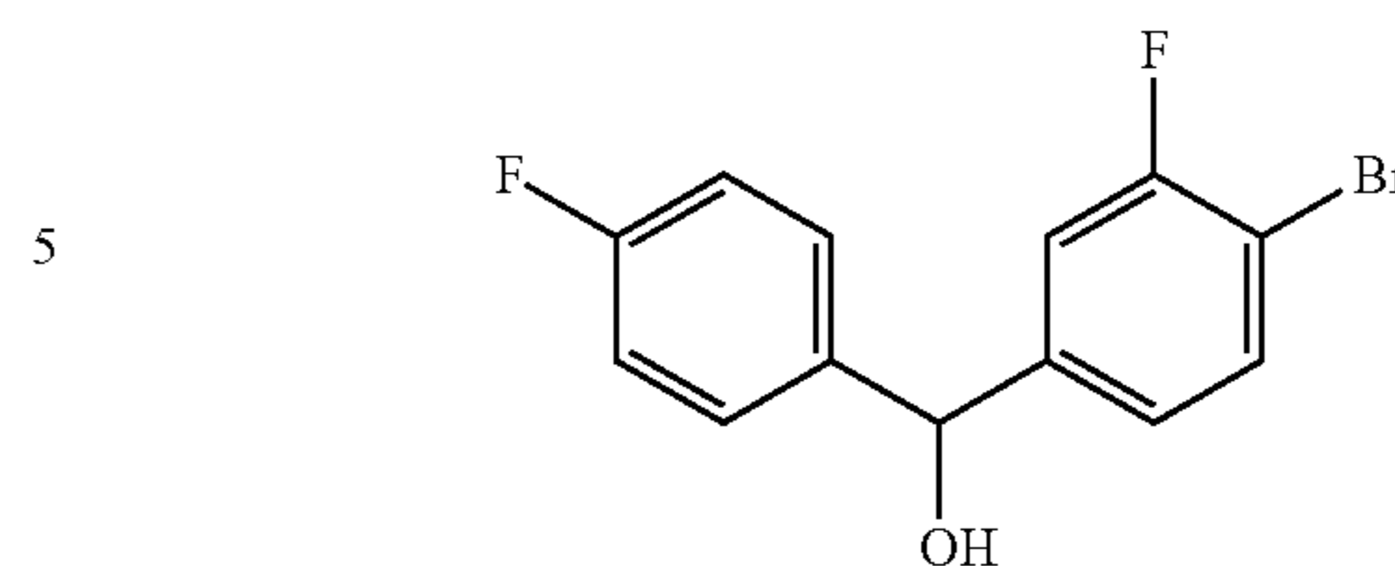
(4-bromo-3-fluorophenyl)(4-fluorophenyl)methanol
