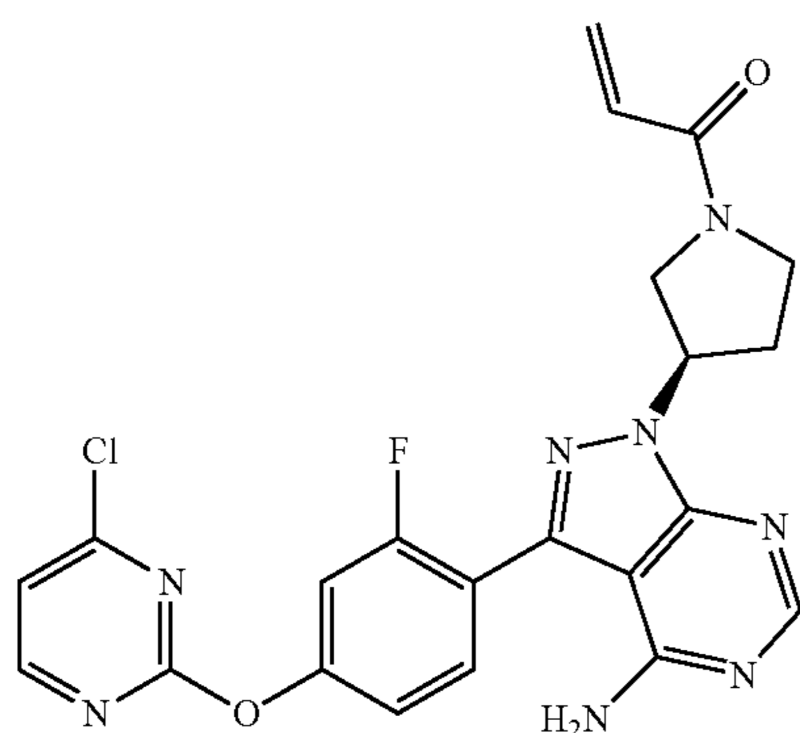
1-((R)-3-(4-amino-3-(4-(4-chloropyrimidin-2-yloxy)-2-fluorophenyl)-1H-pyrazolo[3,4-d]pyrimidin-1-yl)pyrrolidin-1-yl)prop-2-en-1-one
