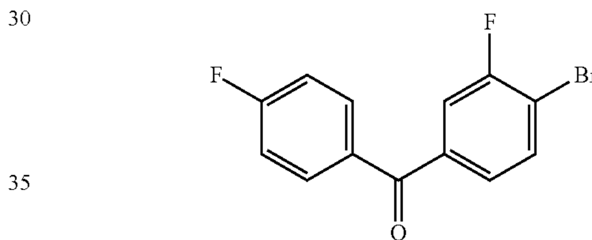
(4-bromo-3-fluorophenyl)(4-fluorophenyl)methanone
