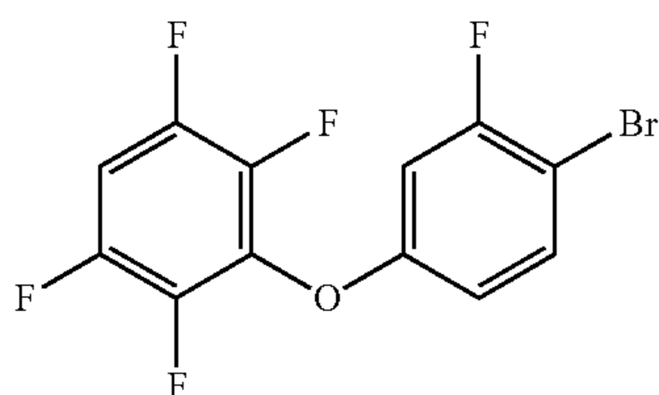
3-(4-bromo-3-fluorophenoxy)-1,2,4,5-tetrafluorobenzene
