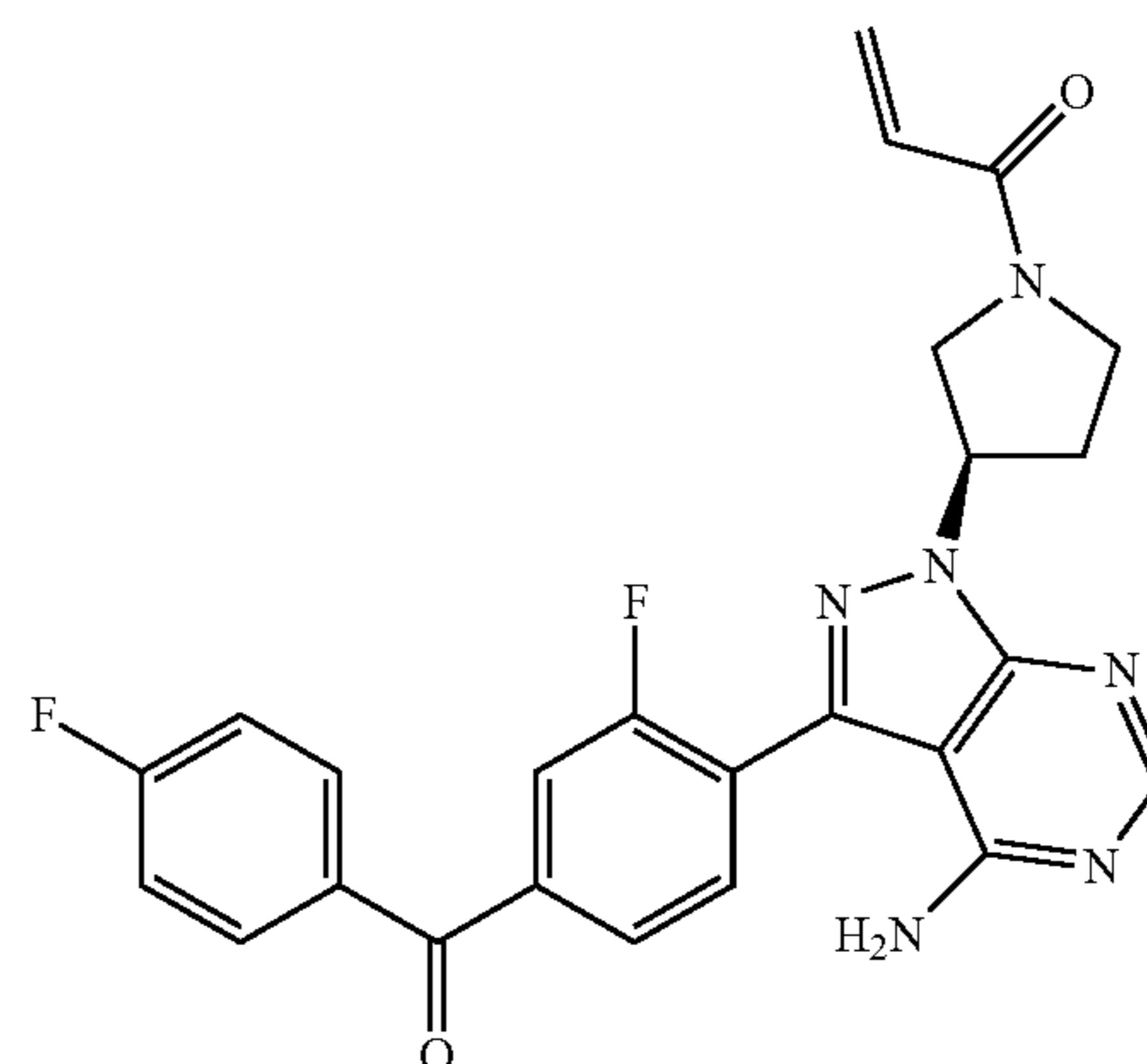
1-((R)-3-(4-amino-3-(2-fluoro-4-(4-fluorobenzoyl)phenyl)-1H-pyrazolo[3,4-d]pyrimidin-1-yl)pyrrolidin-1-yl)prop-2-en-1-one
