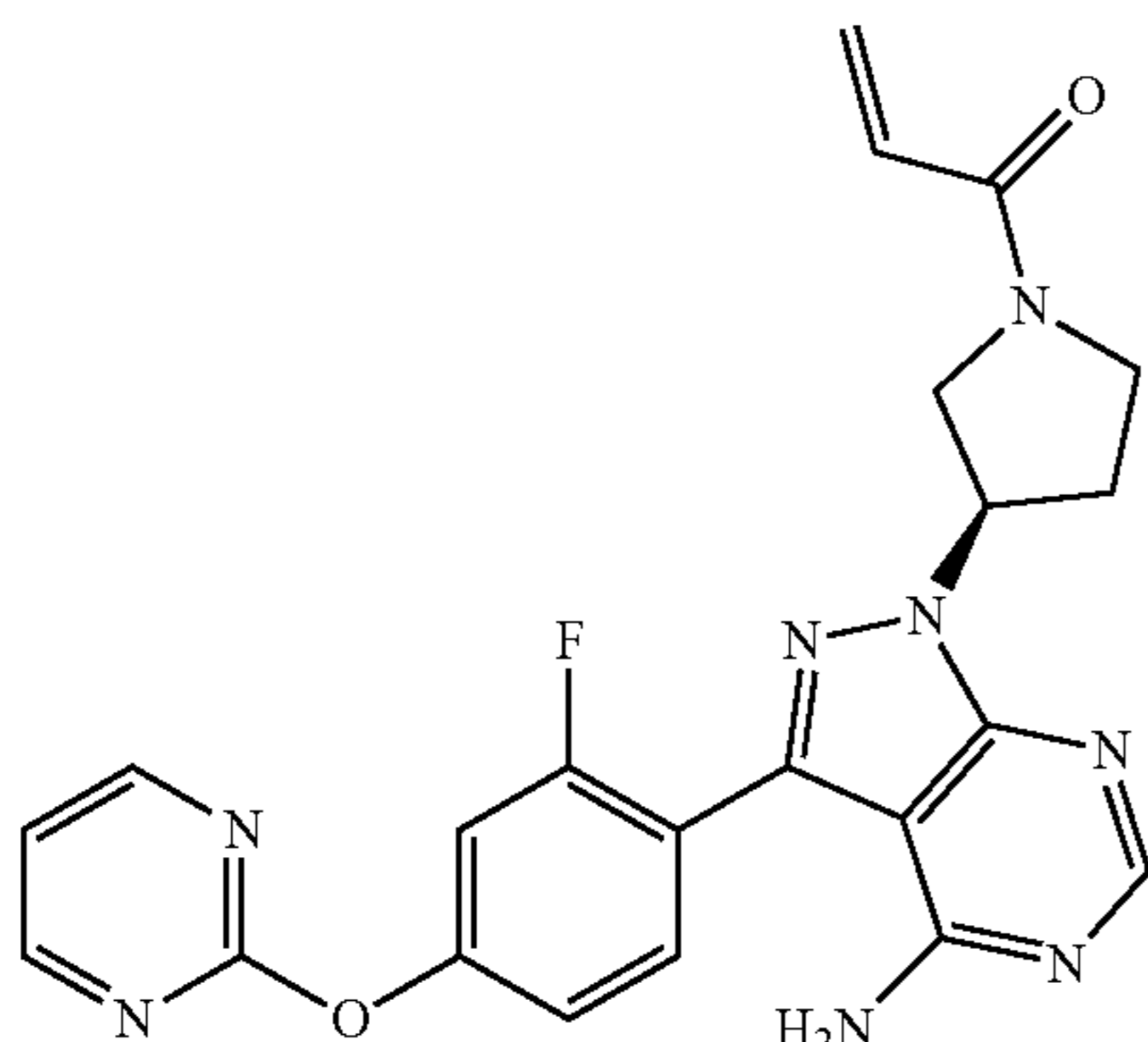
1-((R)-3-(4-amino-3-(2-fluoro-4-(pyrimidin-2-yloxy)phenyl)-1H-pyrazolo[3,4-d]pyrimidin-1-yl)pyrrolidin-1-yl)prop-2-en-1-one
