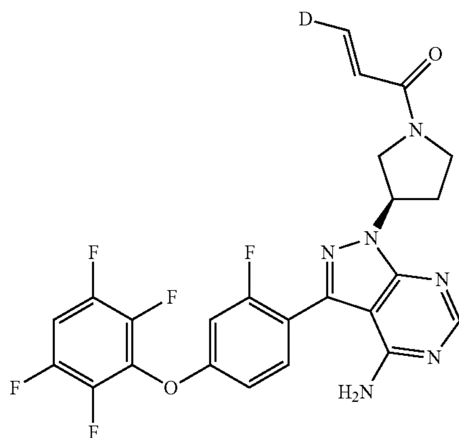
(E)-1-((R)-3-(4-amino-3-(2-fluoro-4-(2,3,5,6-tetrafluorophenoxy)phenyl)-1H-pyrrolo[2,3-d]pyrimidin-1-yl)pyrrolidin-1-yl)-3-deuterium-prop-2-en-1-one
