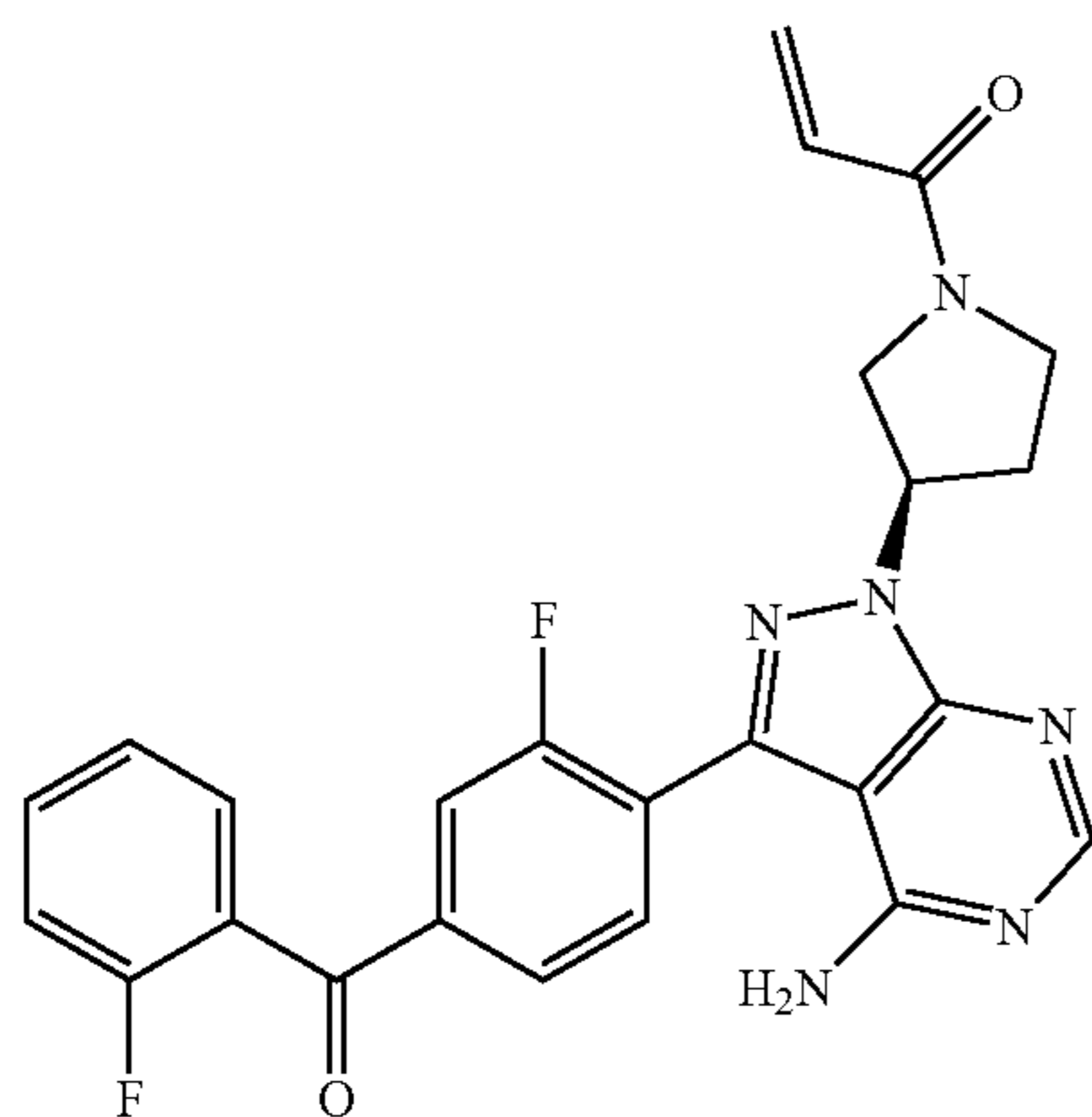
1-((R)-3-(4-amino-3-(2-fluoro-4-(2-fluorobenzoyl)phenyl)-1H-pyrazolo[3,4-d]pyrimidin-1-yl)pyrrolidin-1-yl)prop-2-en-1-one
