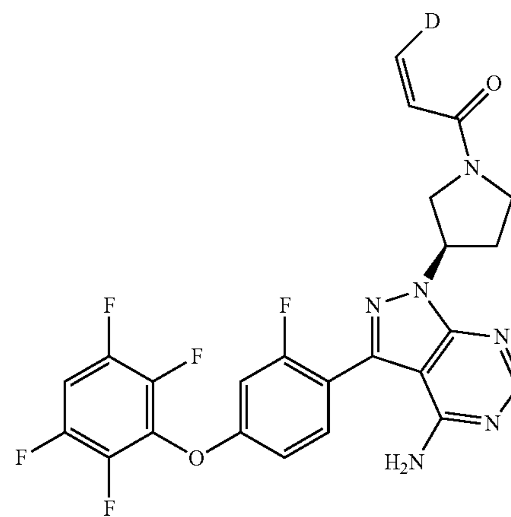
(Z)-1-((R)-3-(4-amino-3-(2-fluoro-4-(2,3,5,6-tetrafluorophenoxy)phenyl)-1H-pyrrolo[2,3-d]pyrimidin-1-yl)pyrrolidin-1-yl)-3-deuterium-prop-2-en-1-one
