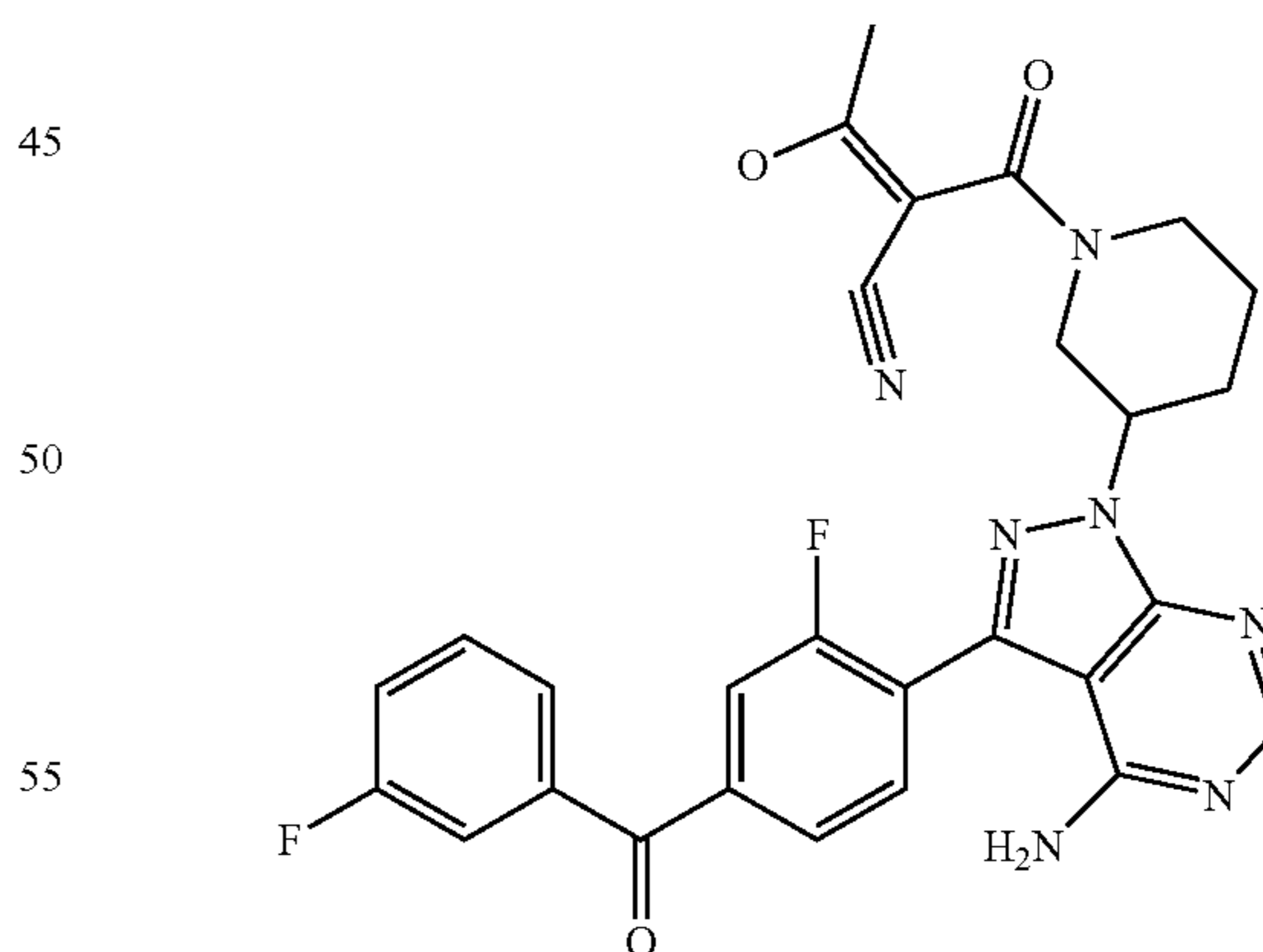
(E)-2-(3-(4-amino-3-(2-fluoro-4-(3-fluorobenzoyl)phenyl)-1H-pyrazolo[3,4-d]pyrimidin-1-yl)piperidine-1-carbonyl)-3-hydroxybut-2-enitrile
