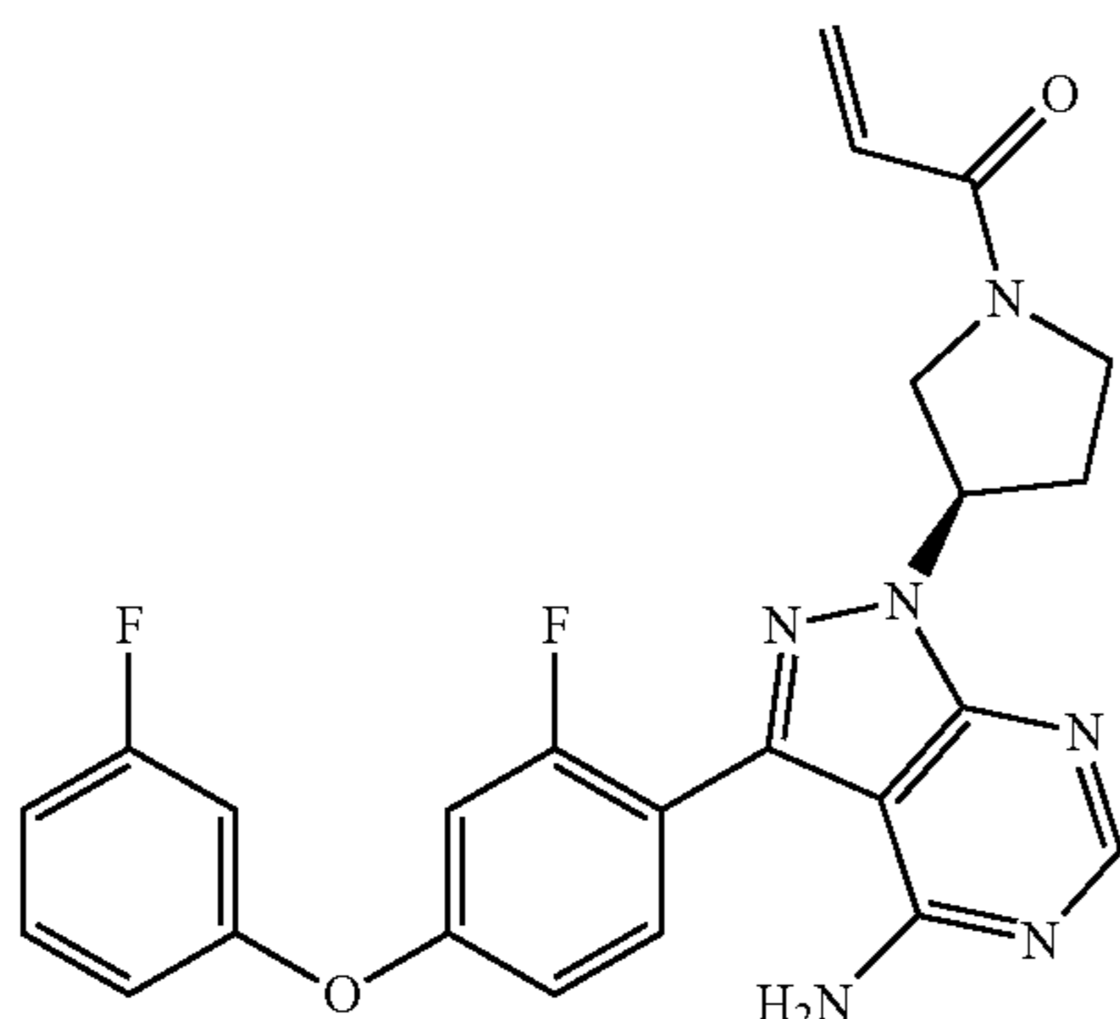
1-((R)-3-(4-amino-3-(2-fluoro-4-(3-fluorophenoxy)phenyl)-1H-pyrazolo[3,4-d]pyrimidin-1-yl)pyrrolidin-1-yl)prop-2-en-1-one
