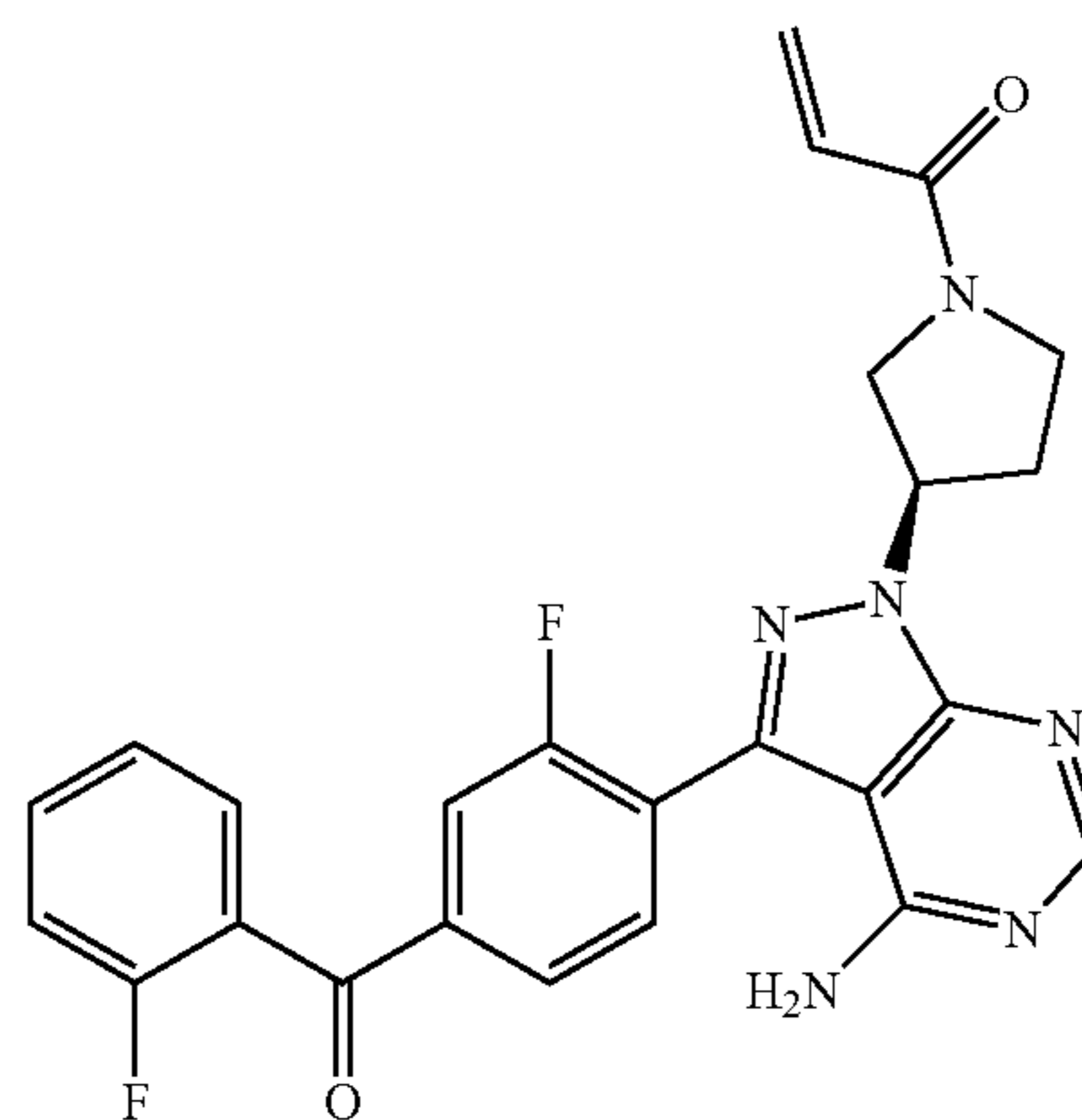
1-((R)-3-(4-amino-3-(2-fluoro-4-(2-fluorobenzoyl)phenyl)-1H-pyrazolo[3,4-d]pyrimidin-1-yl)pyrrolidin-1-yl)prop-2-en-1-one
