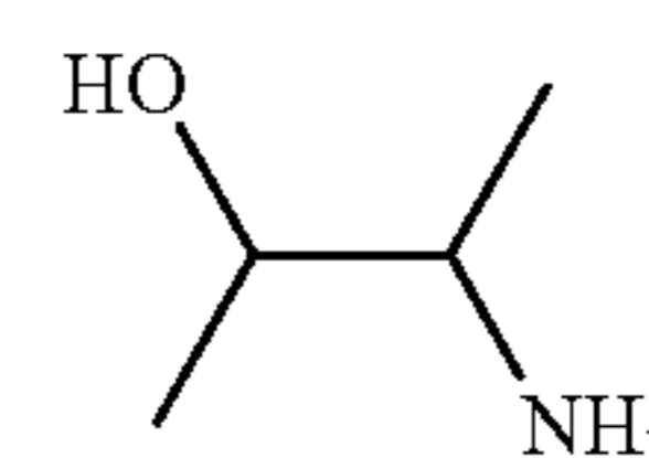
3-aminobutan-2-ol
