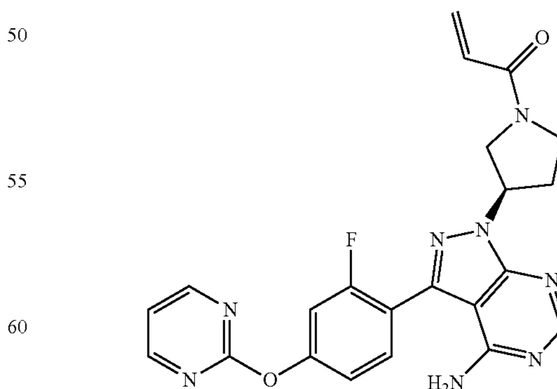
1-((R)-3-(4-amino-3-(2-fluoro-4-(pyrimidin-2-yloxy)phenyl)-1H-pyrazolo[3,4-d]pyrimidin-1-yl)pyrrolidin-1-yl)prop-2-en-1-one
