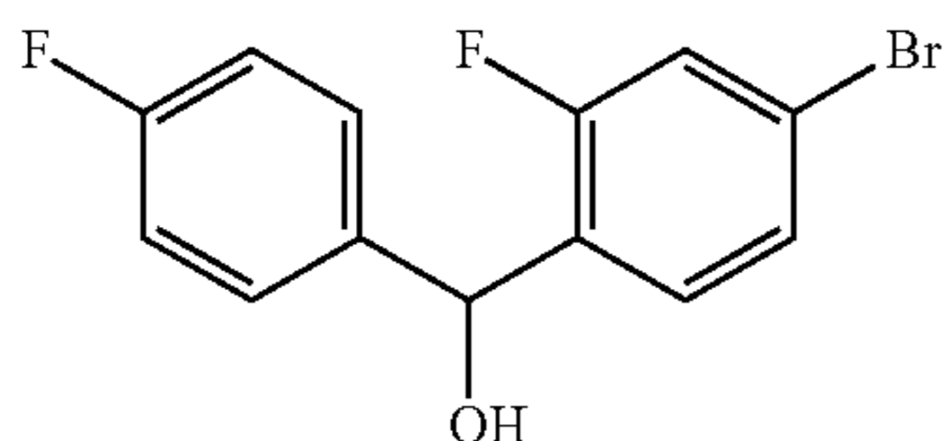
(4-bromo-2-fluorophenyl)(4-fluorophenyl)methanol
