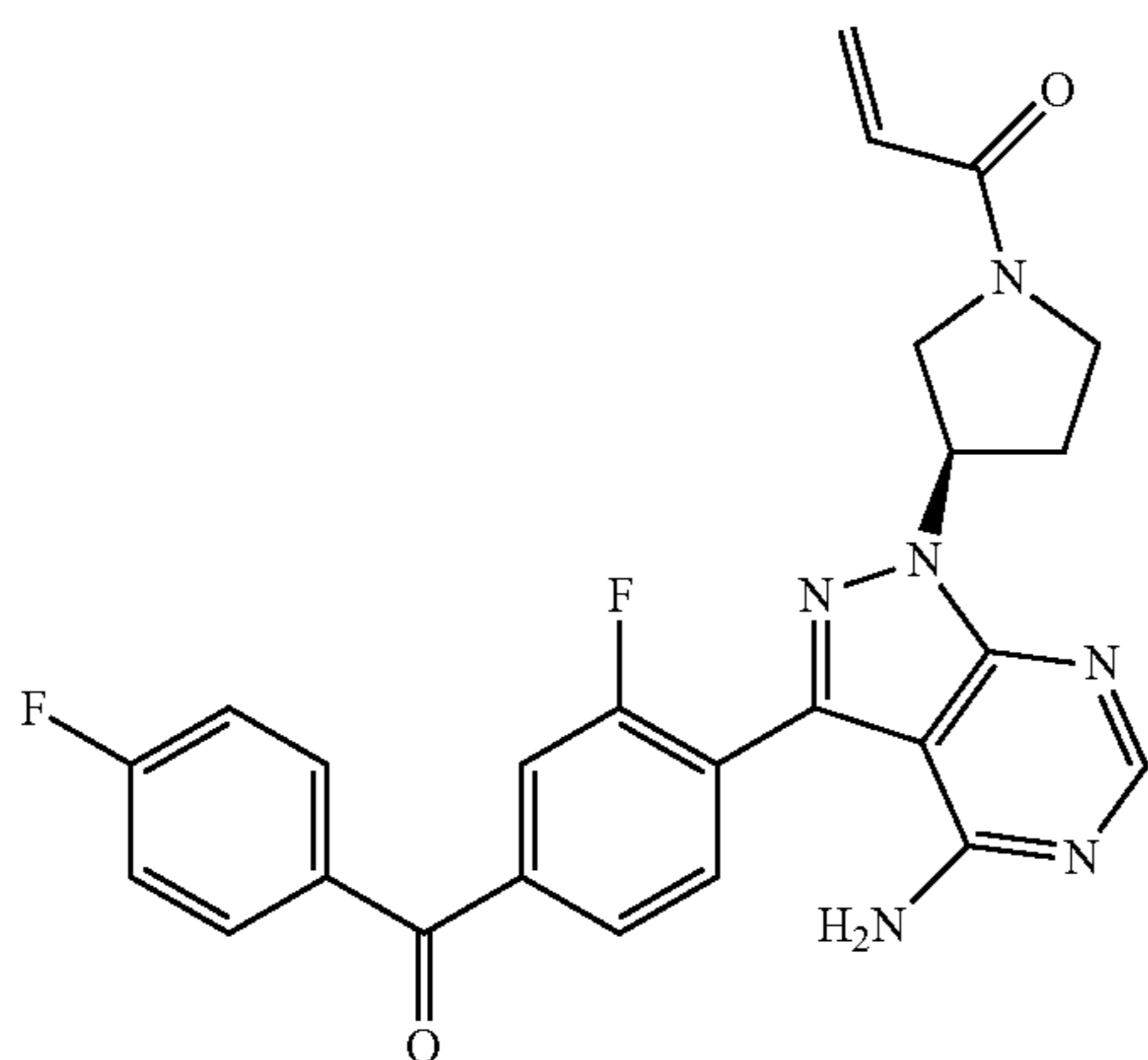
1-((R)-3-(4-amino-3-(2-fluoro-4-(4-fluorobenzoyl)phenyl)-1H-pyrazolo[3,4-d]pyrimidin-1-yl)pyrrolidin-1-yl)prop-2-en-1-one
