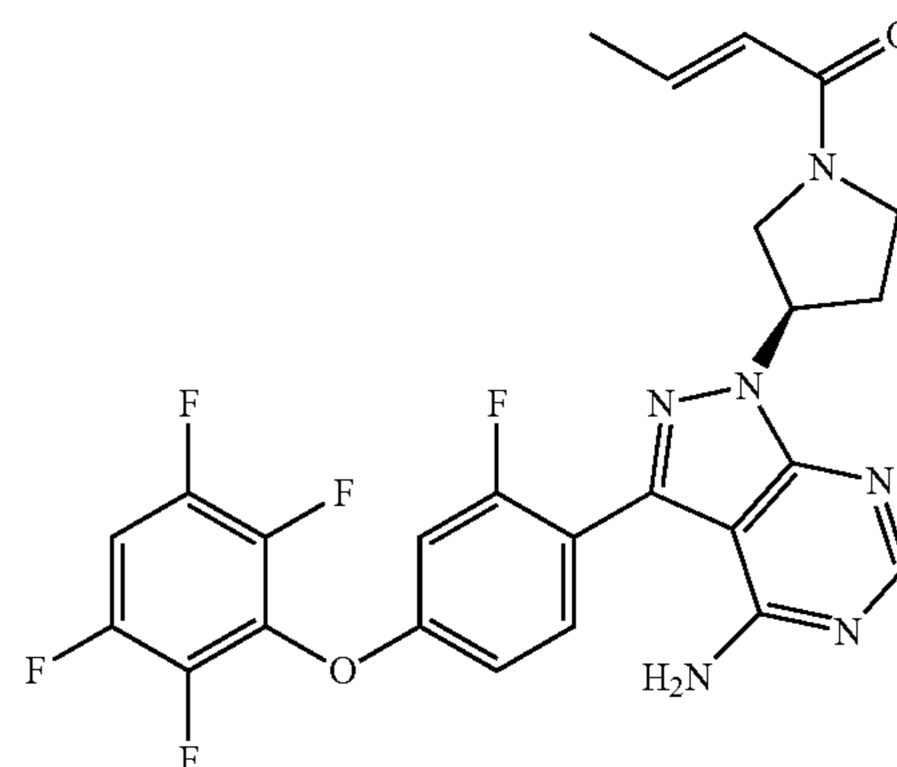
(E)-1-((R)-3-(4-amino-3-(2-fluoro-4-(2,3,5,6-tetrafluorophenoxy)phenyl)-1H-pyrazolo[3,4-d]pyrimidin-1-yl)pyrrolidin-1-yl)but-2-en-1-one
