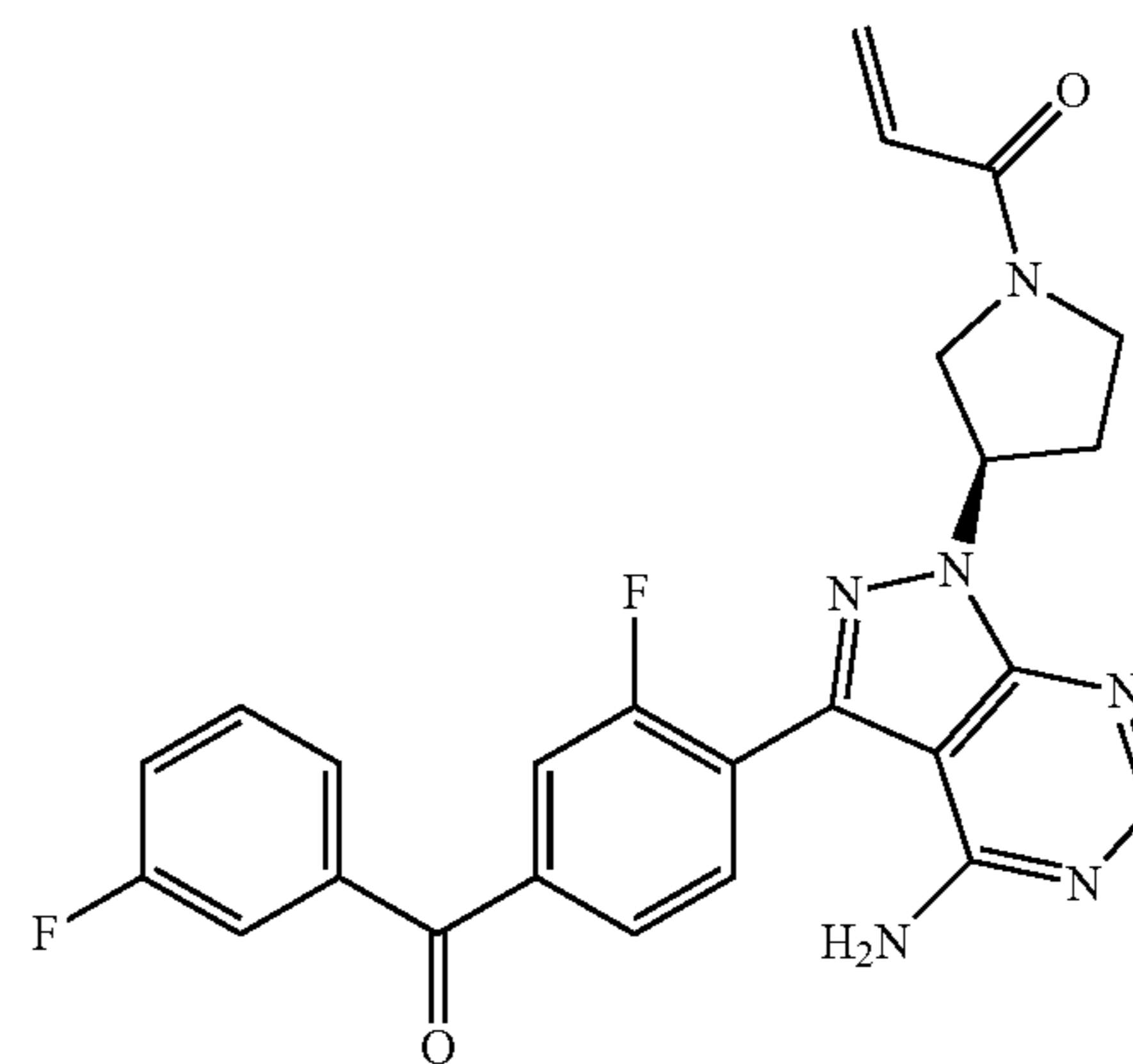
1-((R)-3-(4-amino-3-(2-fluoro-4-(3-fluorobenzoyl)phenyl)-1H-pyrazolo[3,4-d]pyrimidin-1-yl)pyrrolidin-1-yl)prop-2-en-1-one
