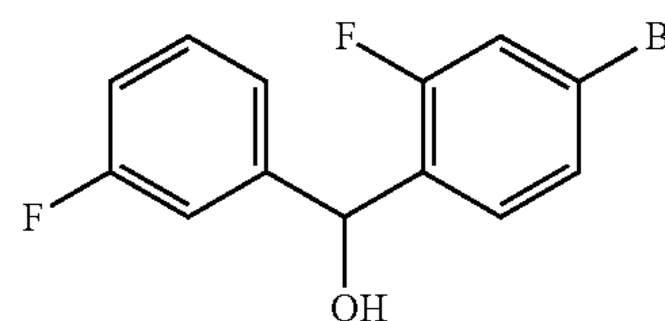
(4-bromo-2-fluorophenyl)(3-fluorophenyl)methanol
