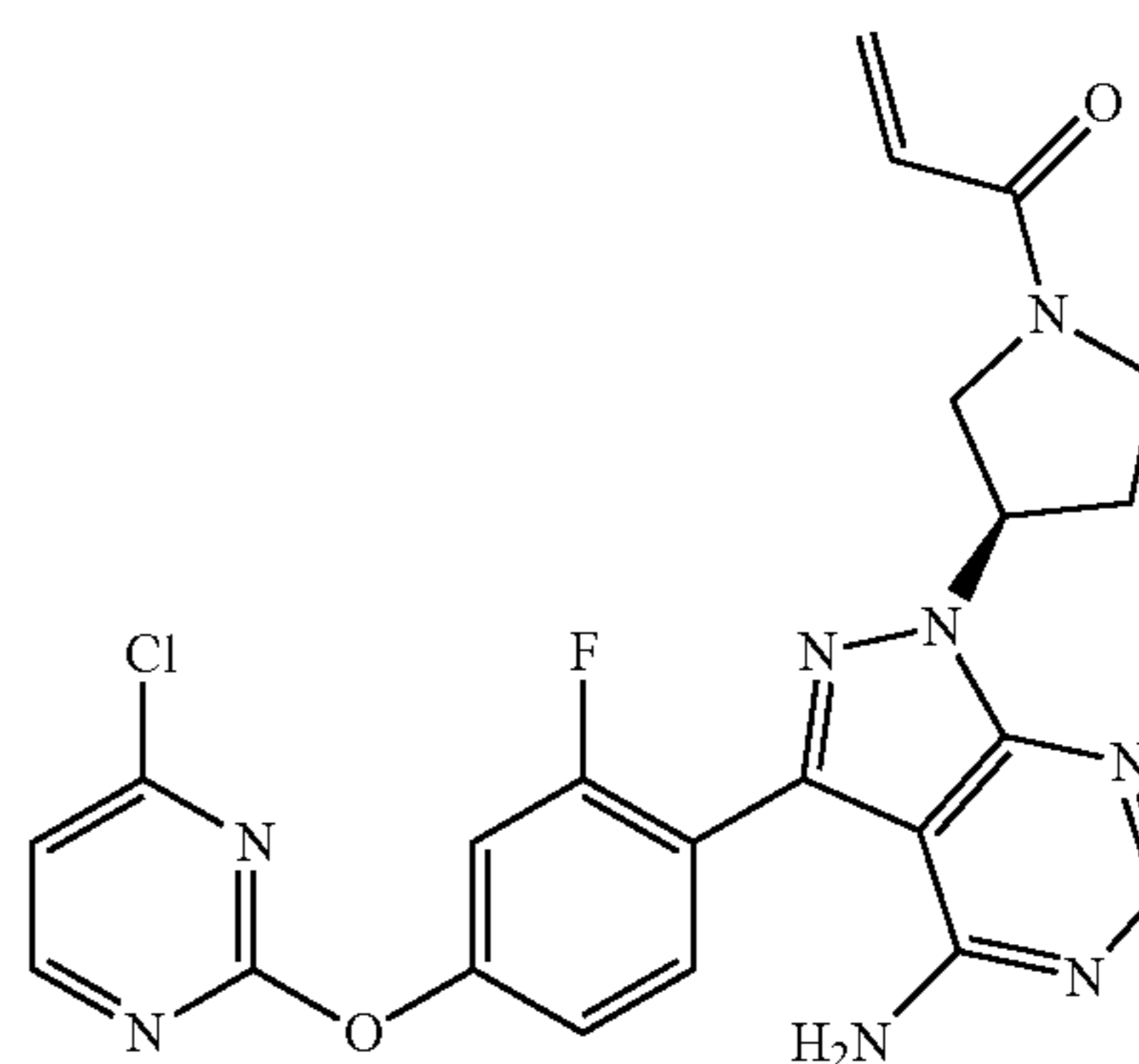
1-((R)-3-(4-amino-3-(4-(4-chloropyrimidin-2-yloxy)-2-fluorophenyl)-1H-pyrazolo[3,4-d]pyrimidin-1-yl)pyrrolidin-1-yl)prop-2-en-1-one
