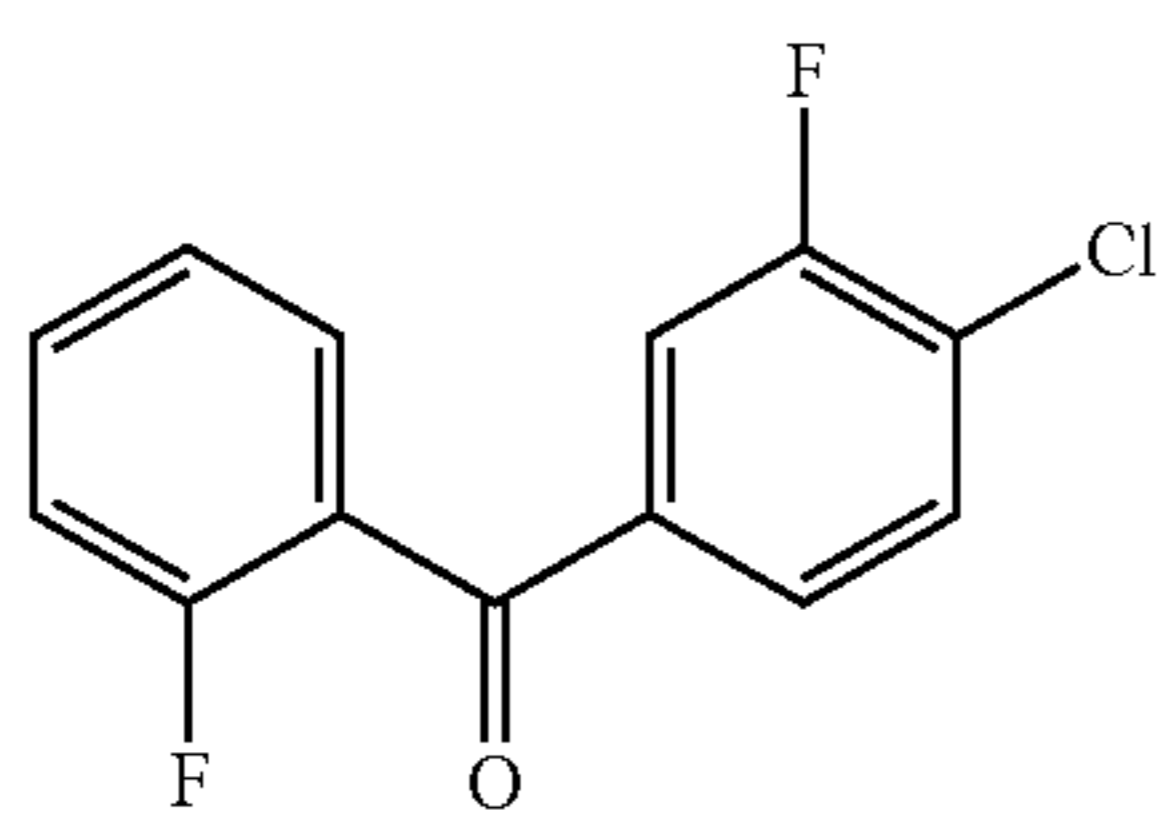
(4-chloro-3-fluorophenyl)(2-fluorophenyl)methanone
