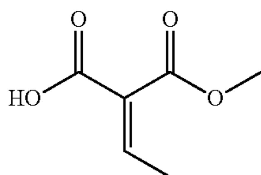
(Z)-2-(methoxycarbonyl)but-2-enoic Acid
