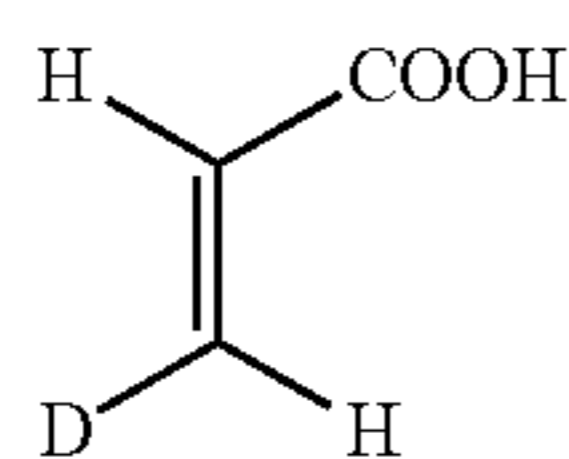
(E)-3-deuterium acrylate
