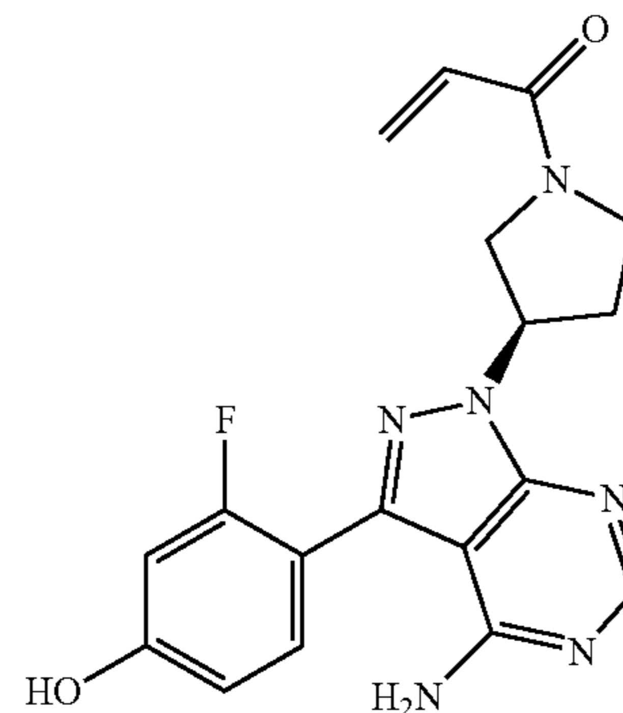
1-((R)-3-(4-amino-3-(2-fluoro-4-hydroxyphenyl)-1H-pyrazolo[3,4-d]pyrimidin-1-yl)pyrrolidin-1-yl)prop-2-en-1-one
