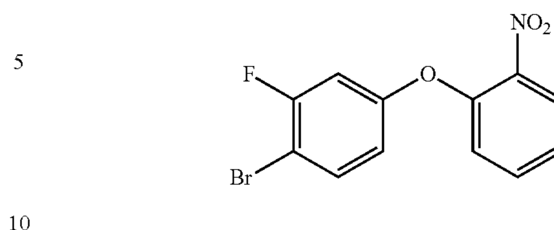
1-(4-bromo-3-fluorophenoxy)-2-nitrobenzene
