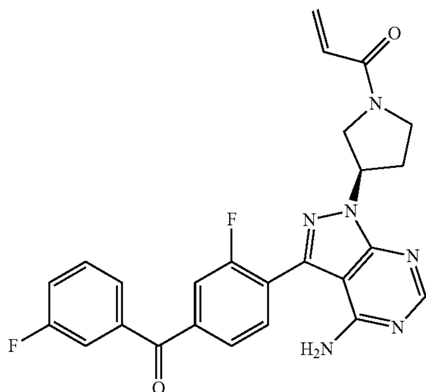
1-((R)-3-(4-amino-3-(2-fluoro-4-(3-fluorobenzoyl)phenyl)-1H-pyrazolo[3,4-d]pyrimidin-1-yl)pyrrolidin-1-yl)prop-2-en-1-one
