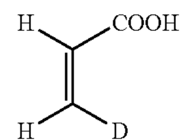
(Z)-3-deuterium acrylate
