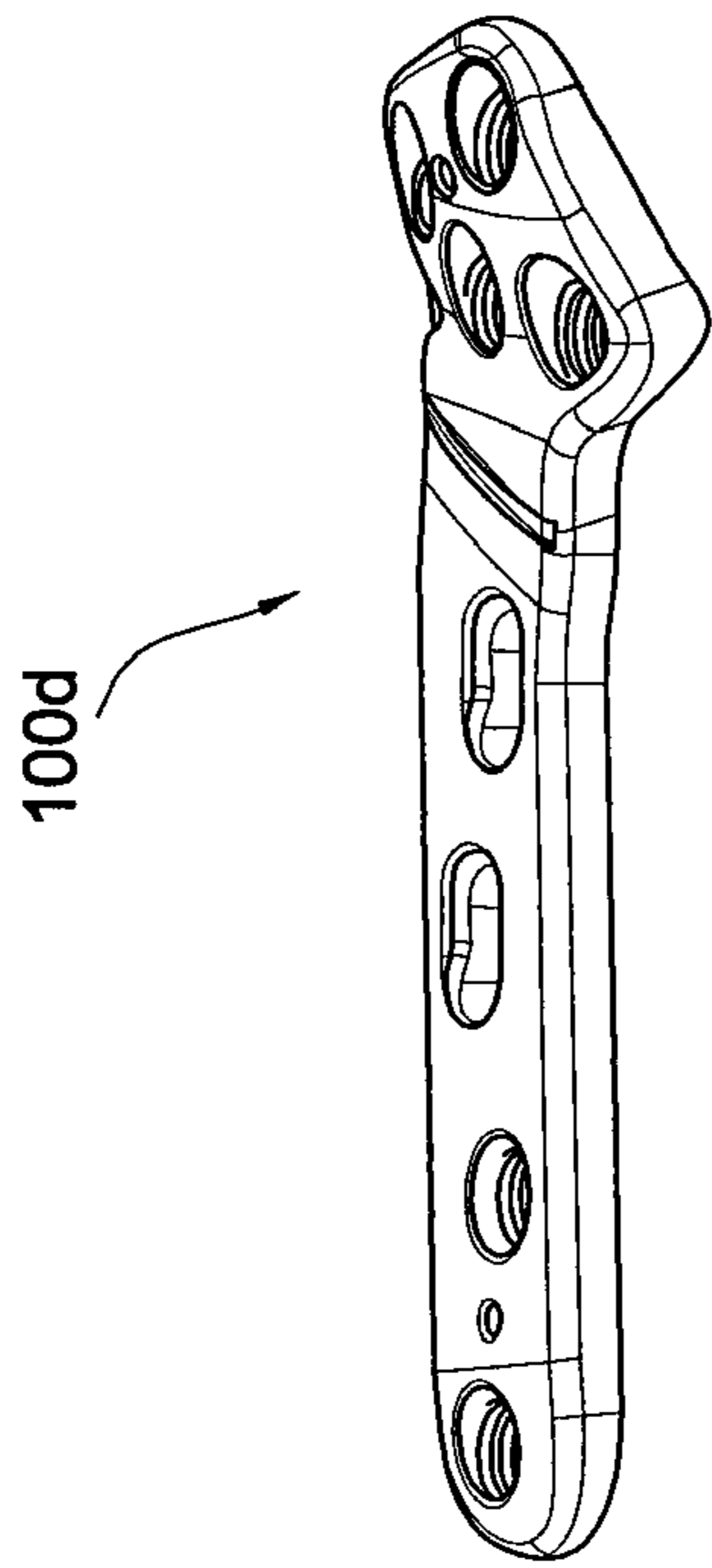
FIG. 13(a)
