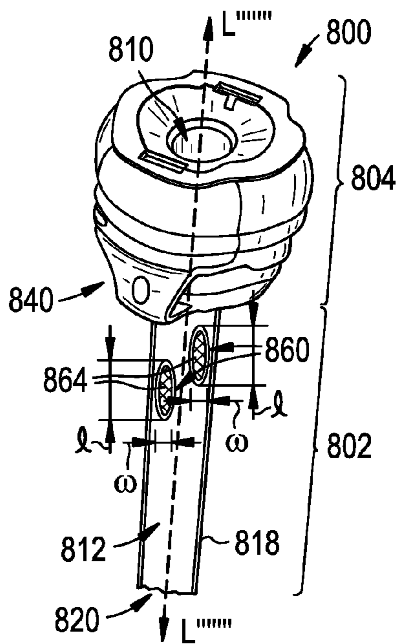
FIG. 17
