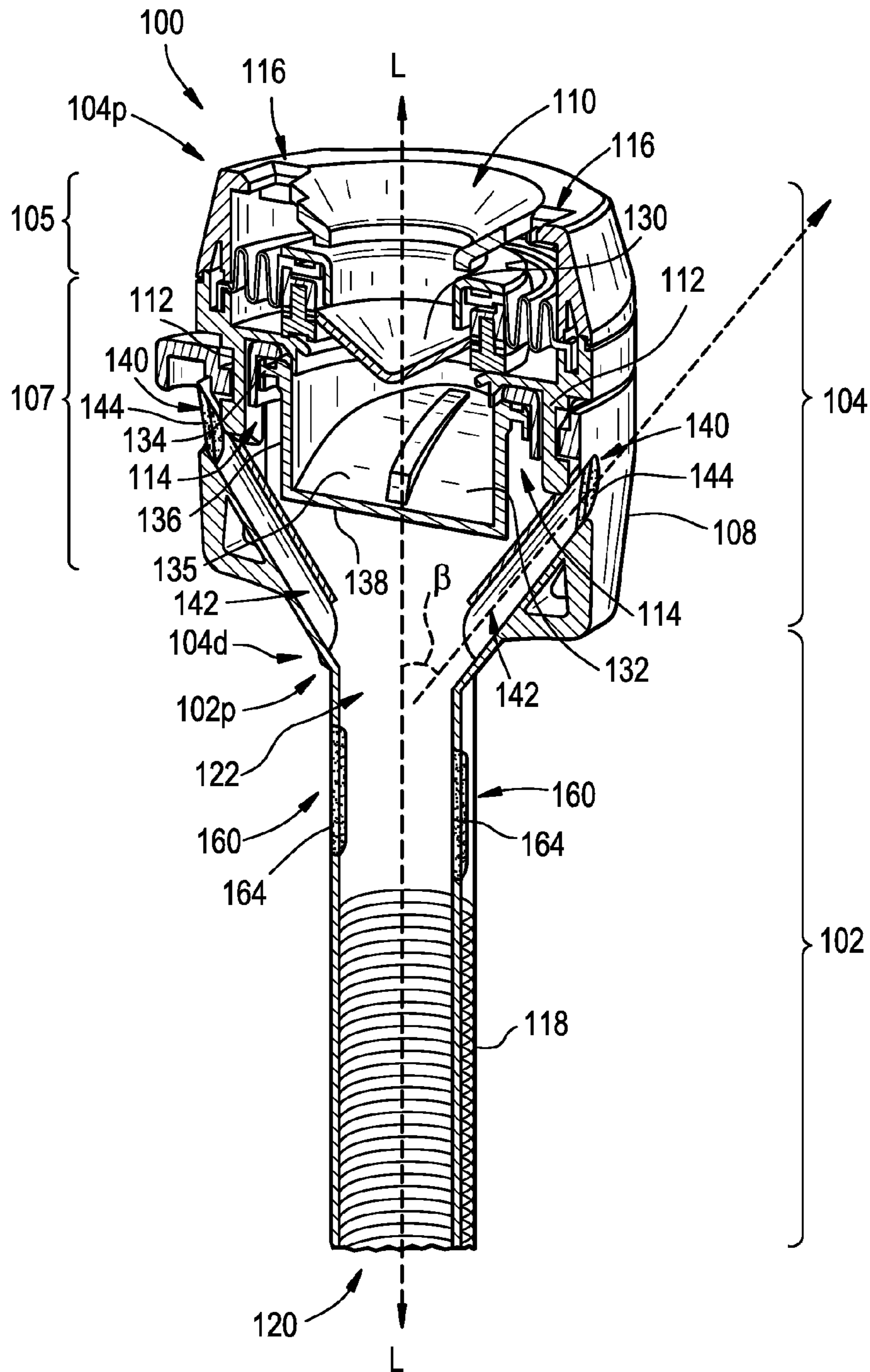
FIG. 2C
