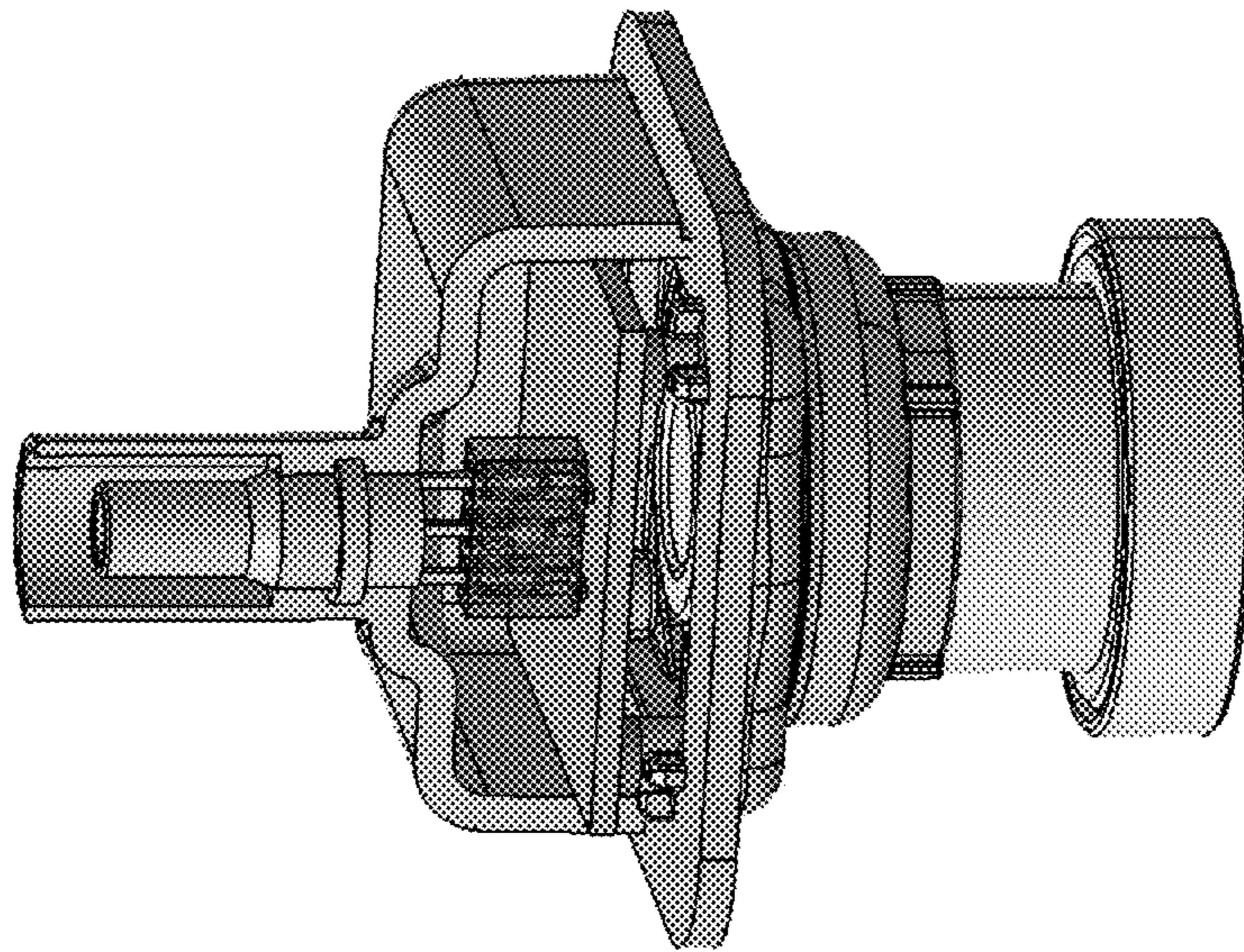
FIG. 12A
