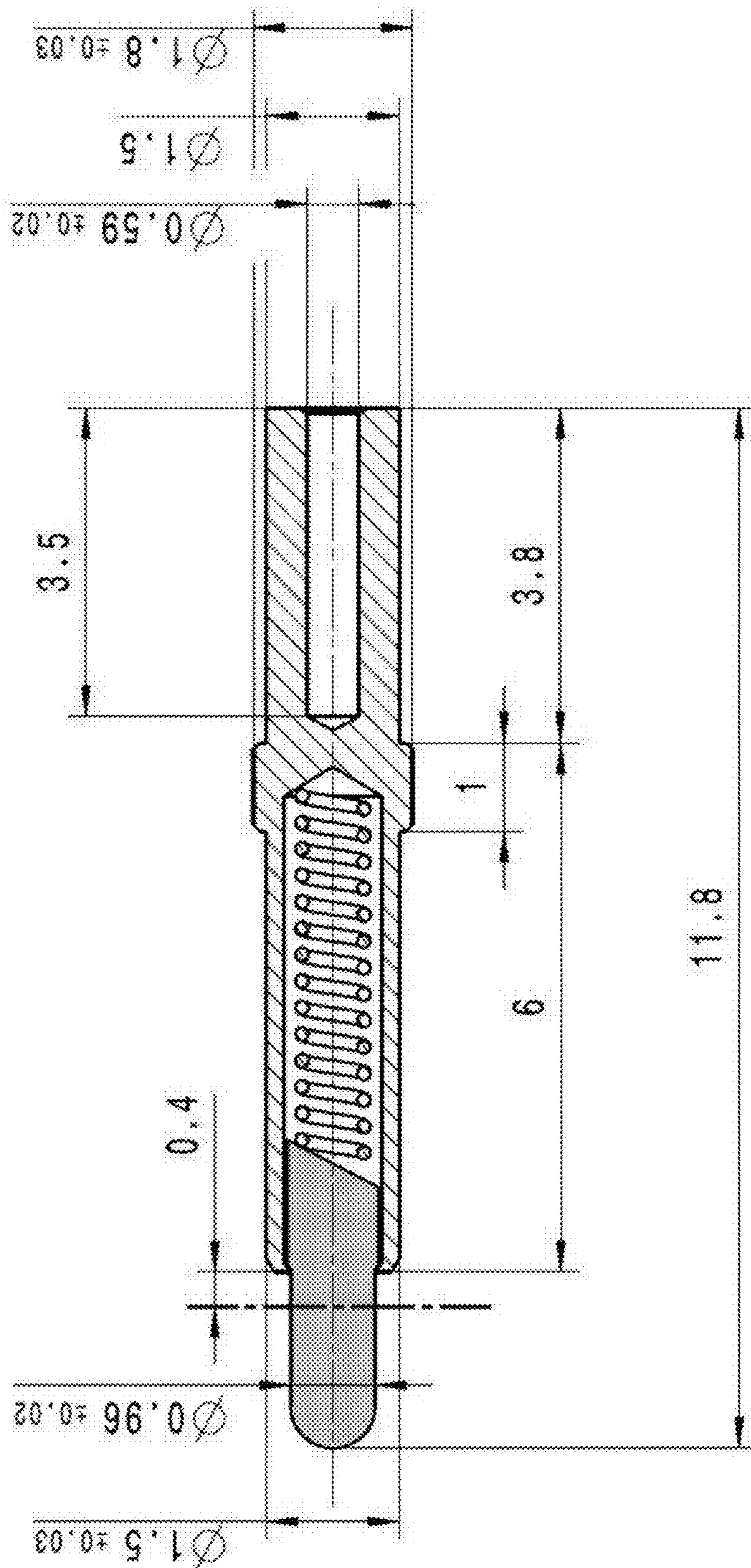
FIG. 39K
