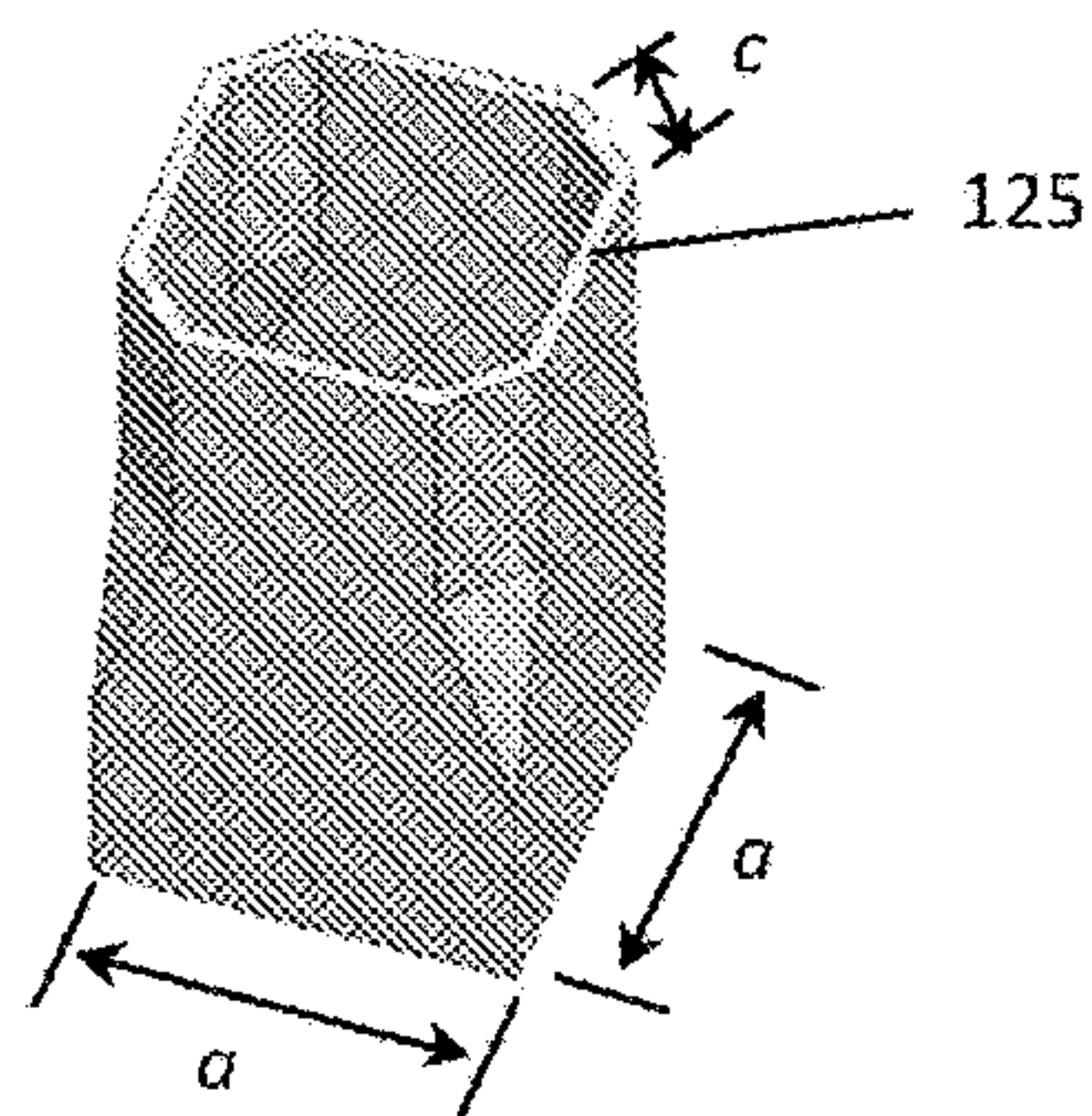
Fig. 4b B-B section
