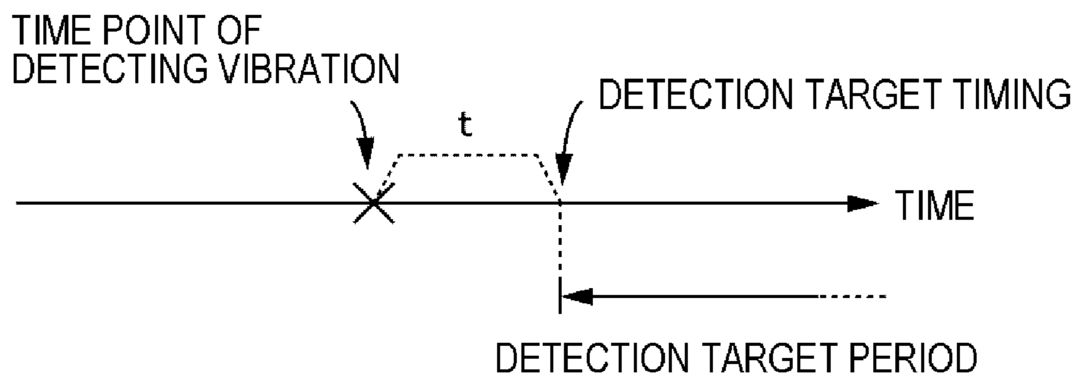
FIG. 11C
