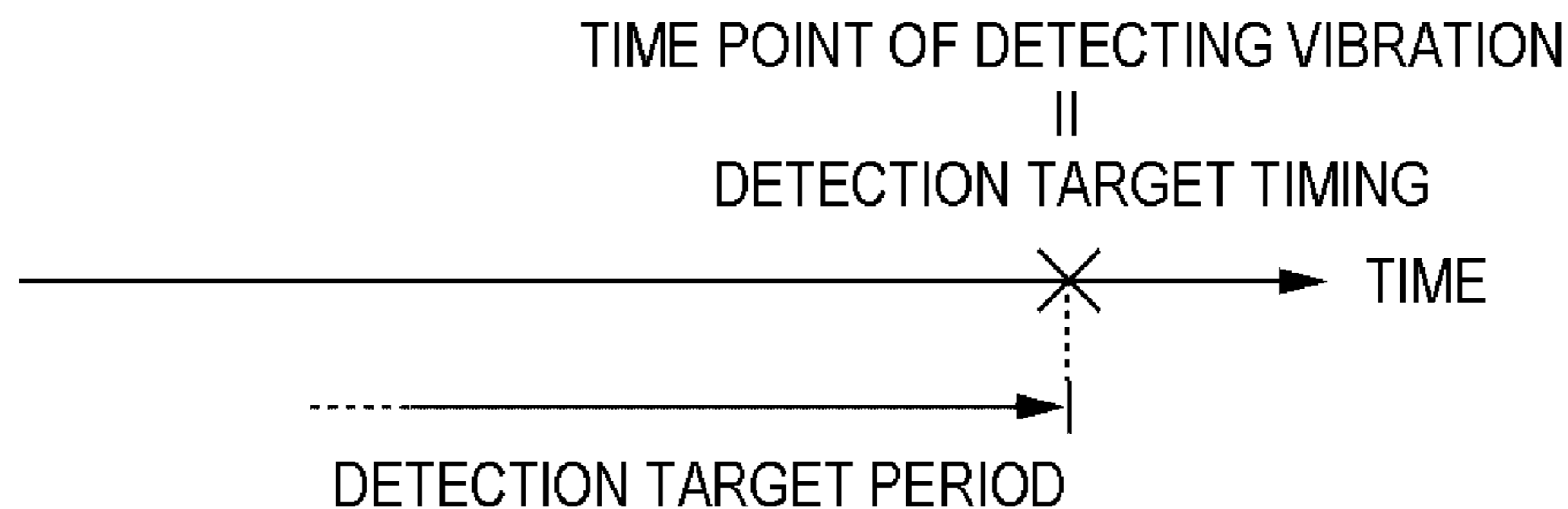
FIG. 12A
