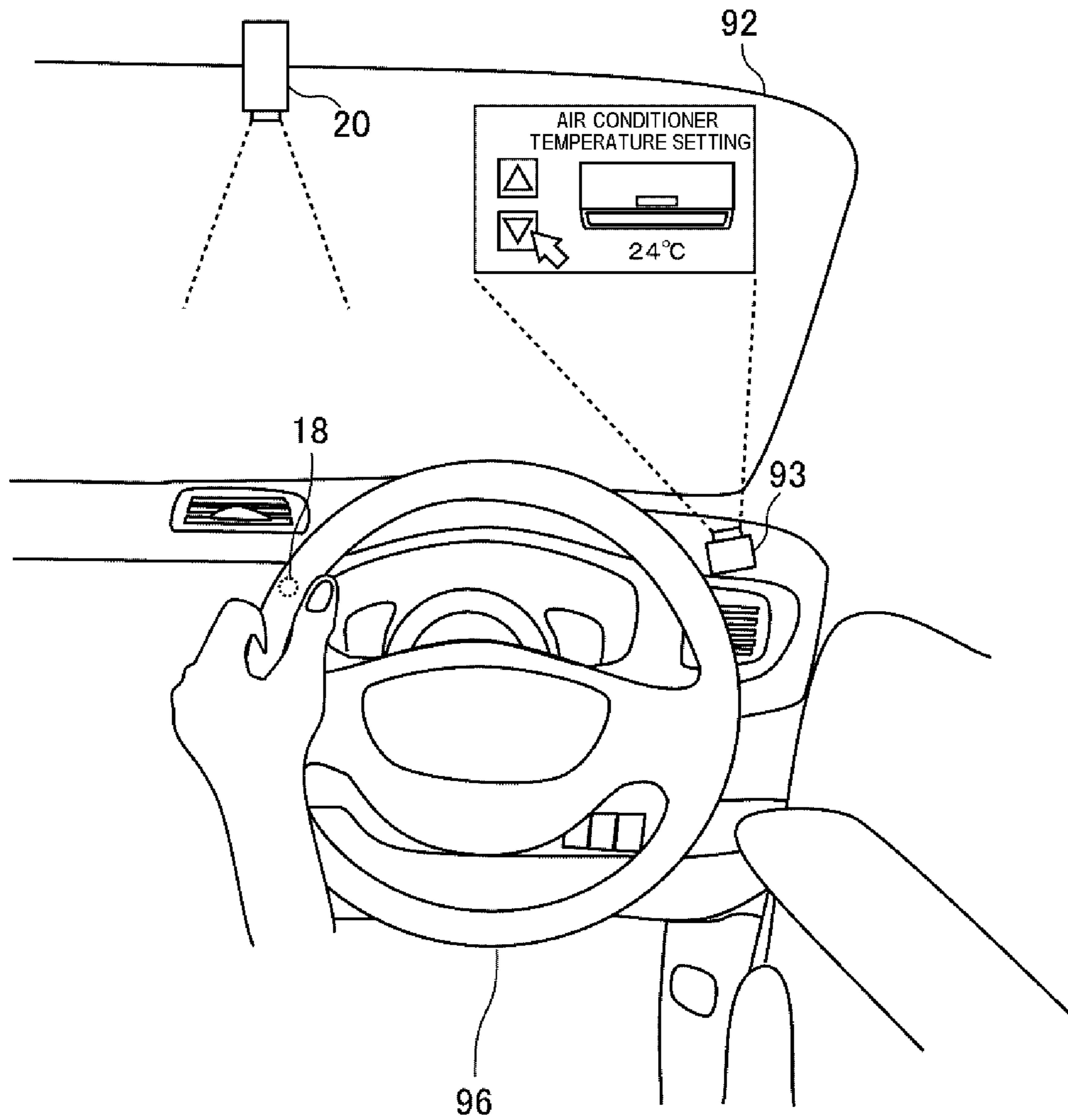
FIG. 27
